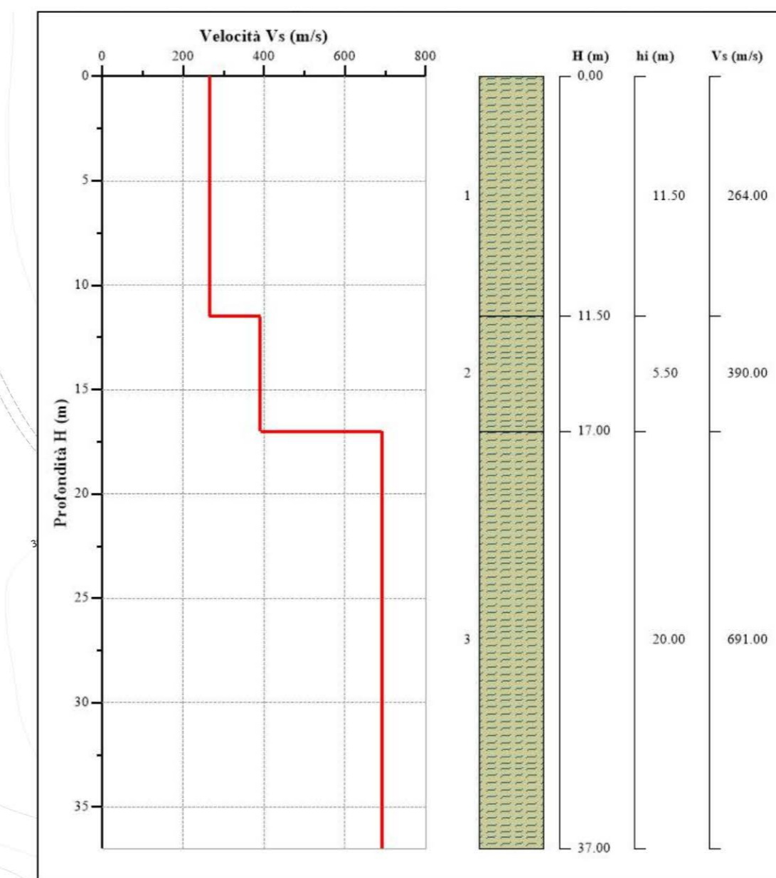
SISMOSTRATIGRAFIA MASW 2 - ZONA 2
