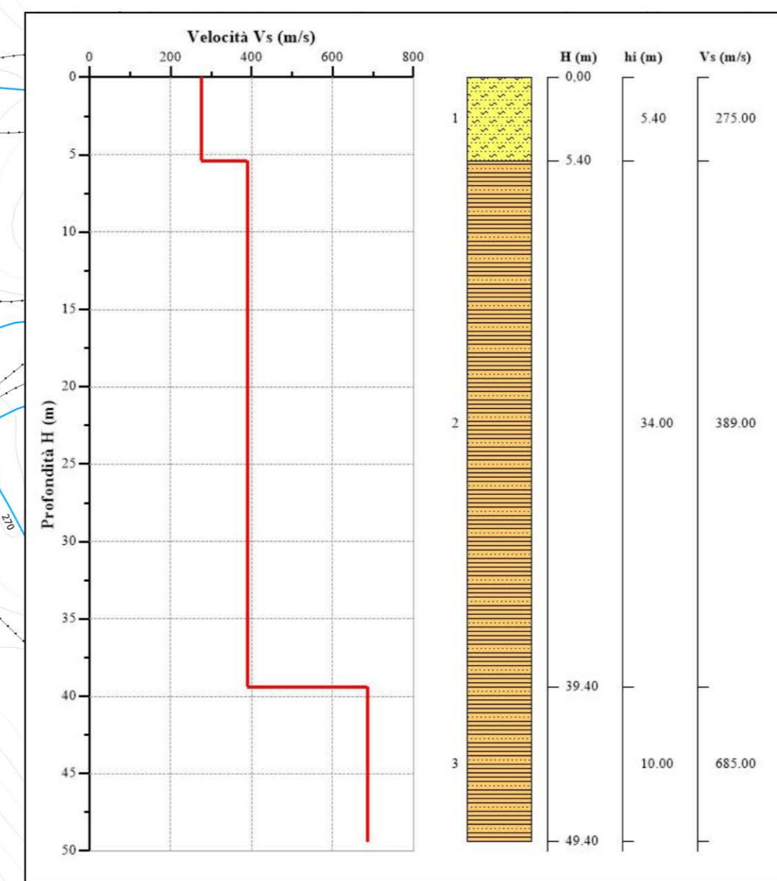
SISMOSTRATIGRAFIA MASW 1 - ZONA 1
