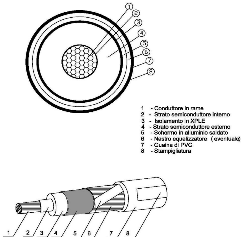
Figura 3 - Schema tipo cavo 150 kV
