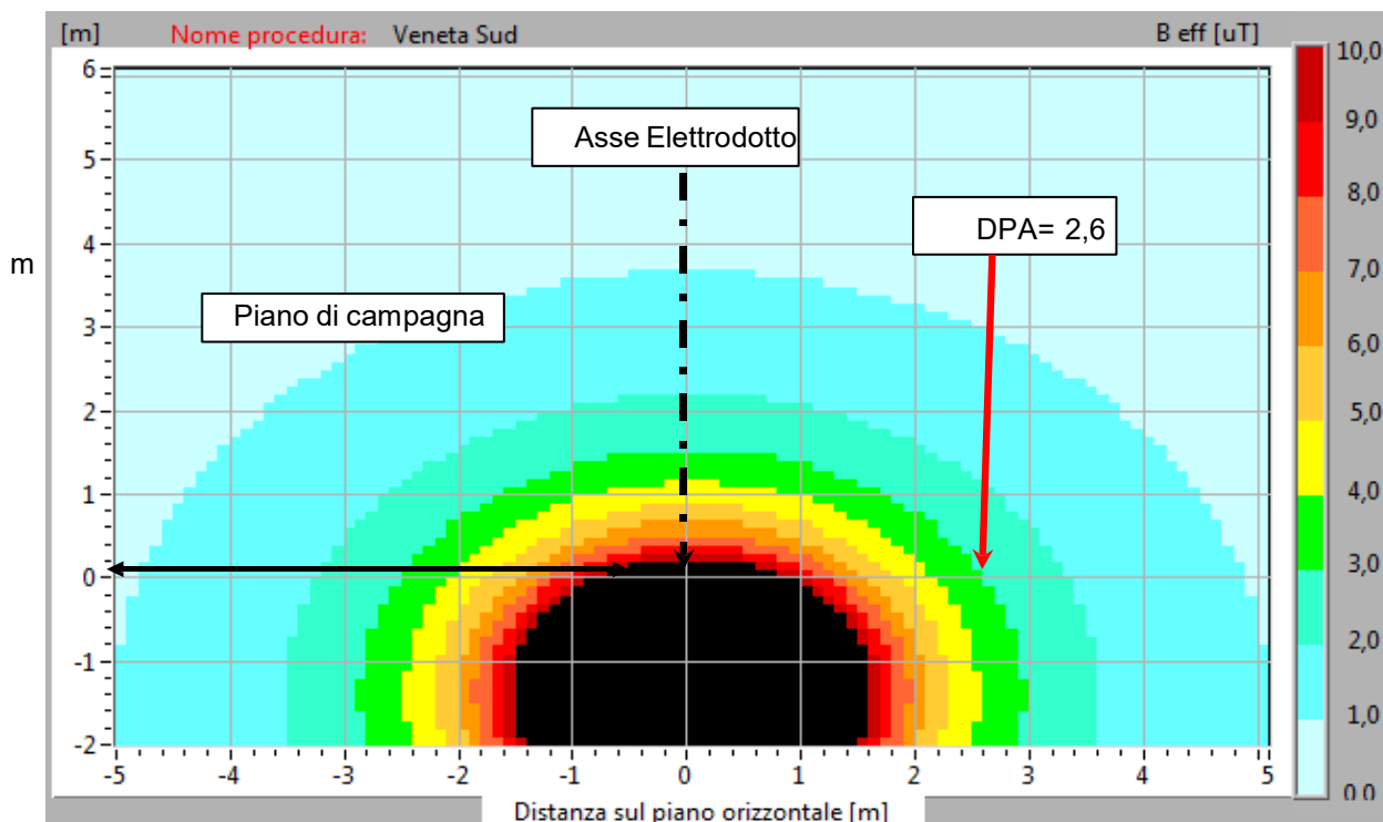
Figura 5 - Mappa verticale induzione magnetica (B) sezione tipo con indicazione della DPA - V=150 kV I = 900 A
