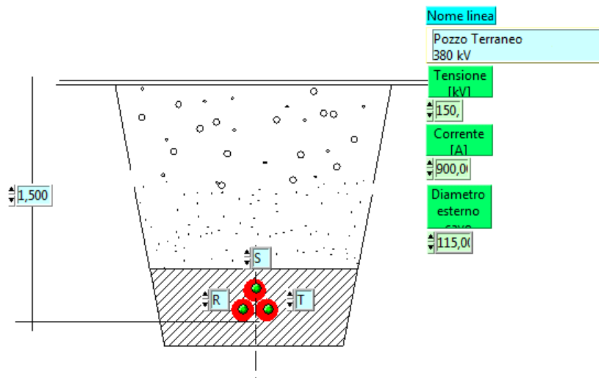
Figura 4 - Sezione tipo
