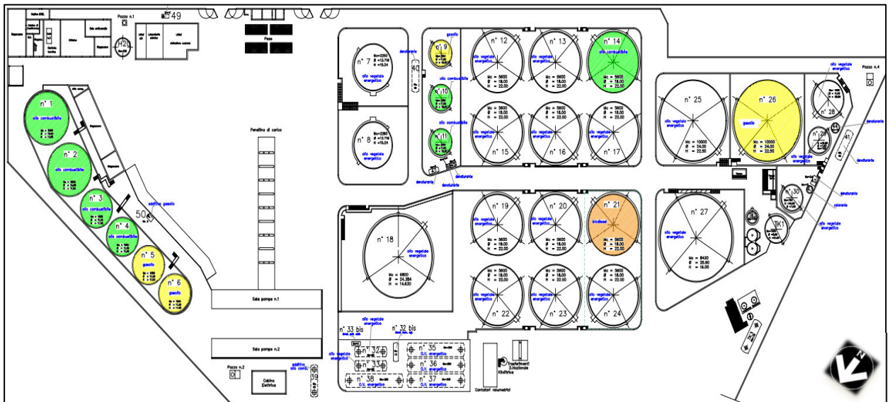
Figura 3-1 - Planimetria stato di fatto Deposito Costiero
