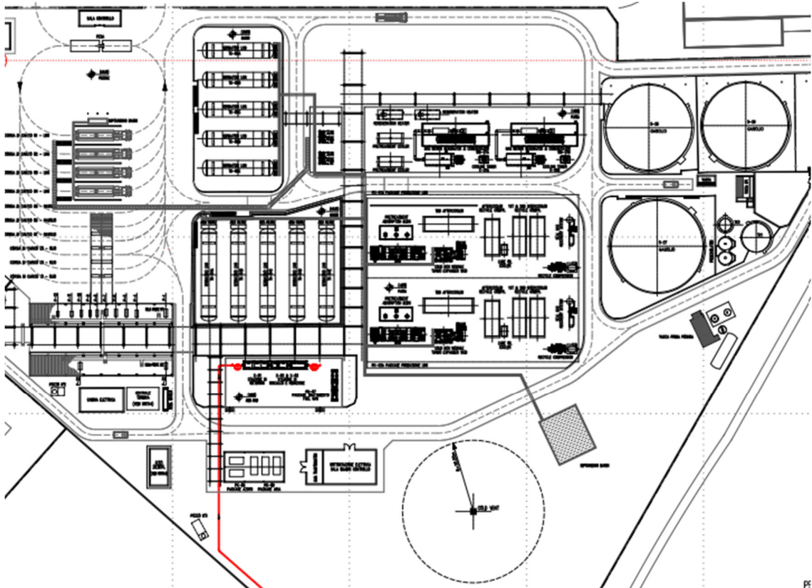
Figura 3-3 – Estratto planimetria di progetto per impianto LNG
