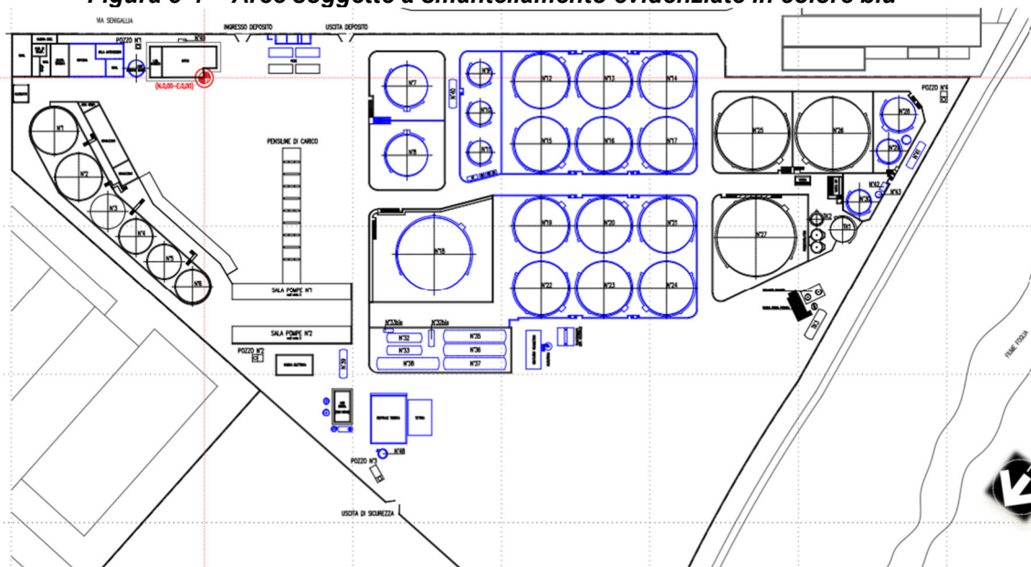
Figura 3-4 - Aree soggette a smantellamento evidenziate in colore blu
