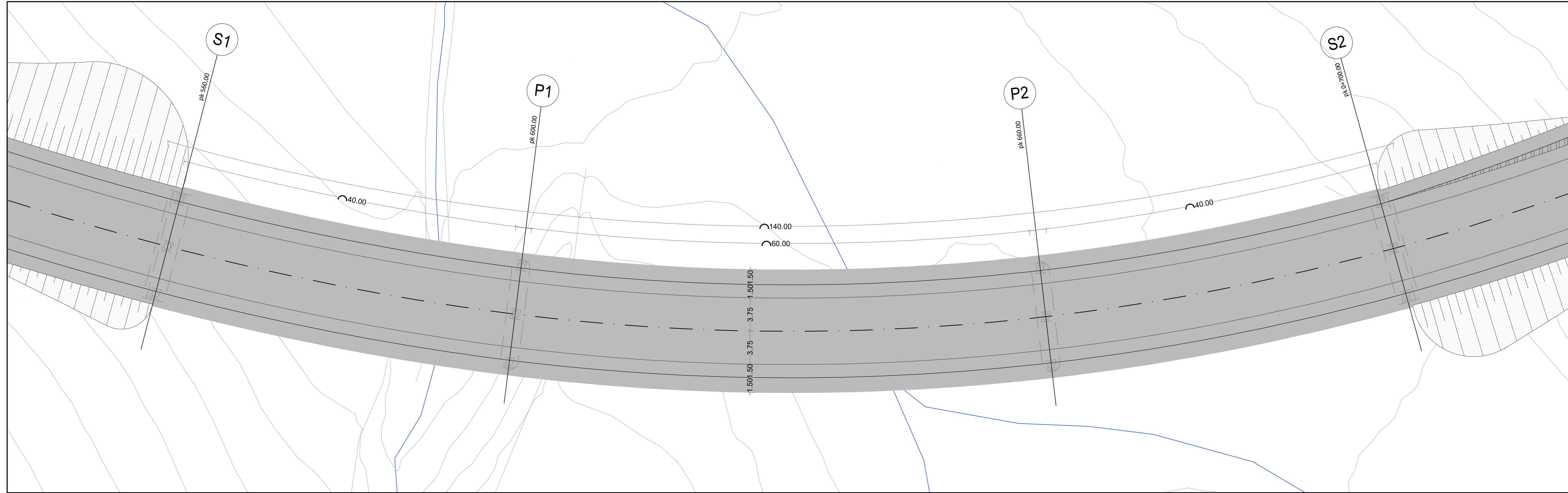
PIANTA IMPALCATO SCALA 1:200
