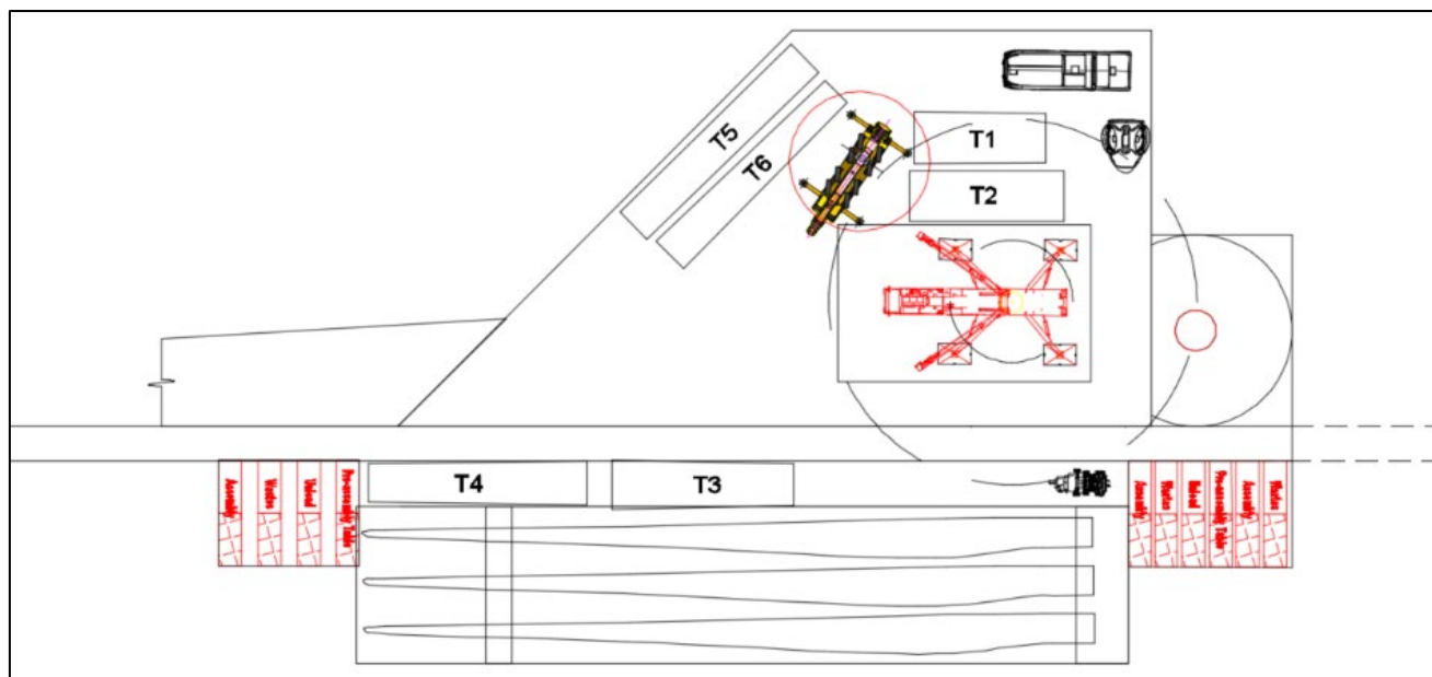
Tipico Piazzola di Cantiere durante la Prima Fase di Montaggio
