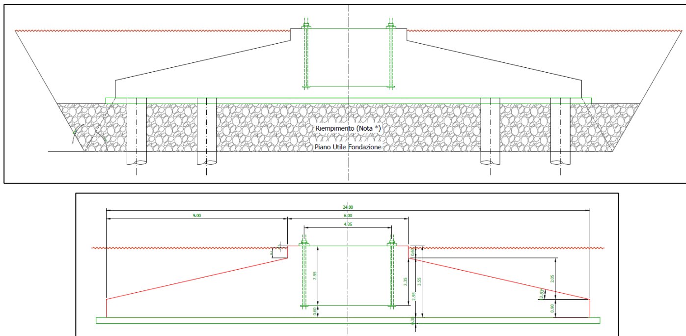
Tipica Sezione di scavo con ingombri di massima del Plinto di Fondazione degli aerogeneratori
