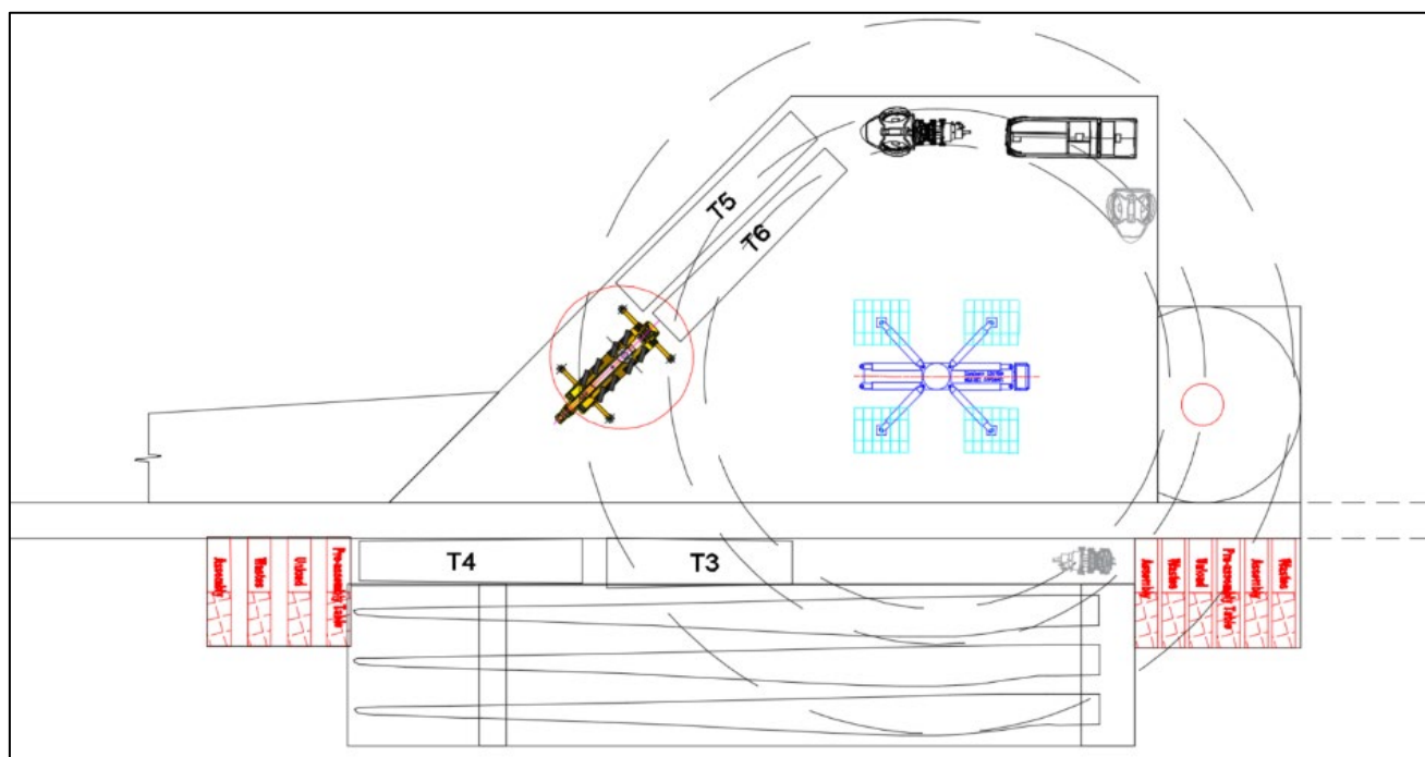
Tipico Piazzola di Cantiere durante la Seconda Fase di Montaggio
