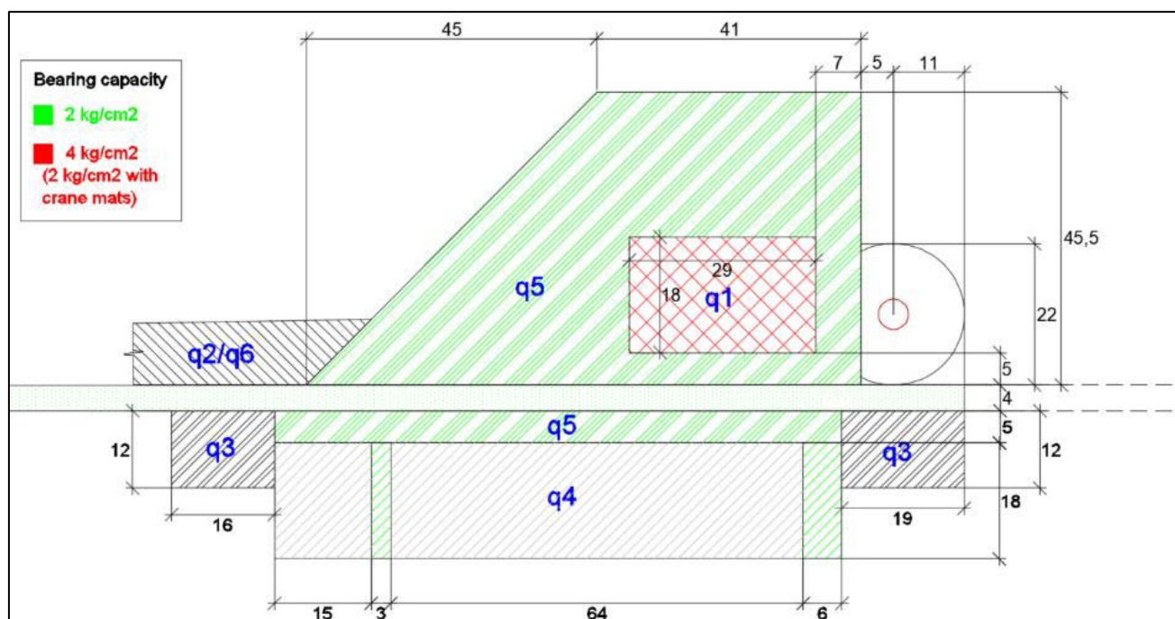
Tipico Piazzola di Cantiere o Montaggio
