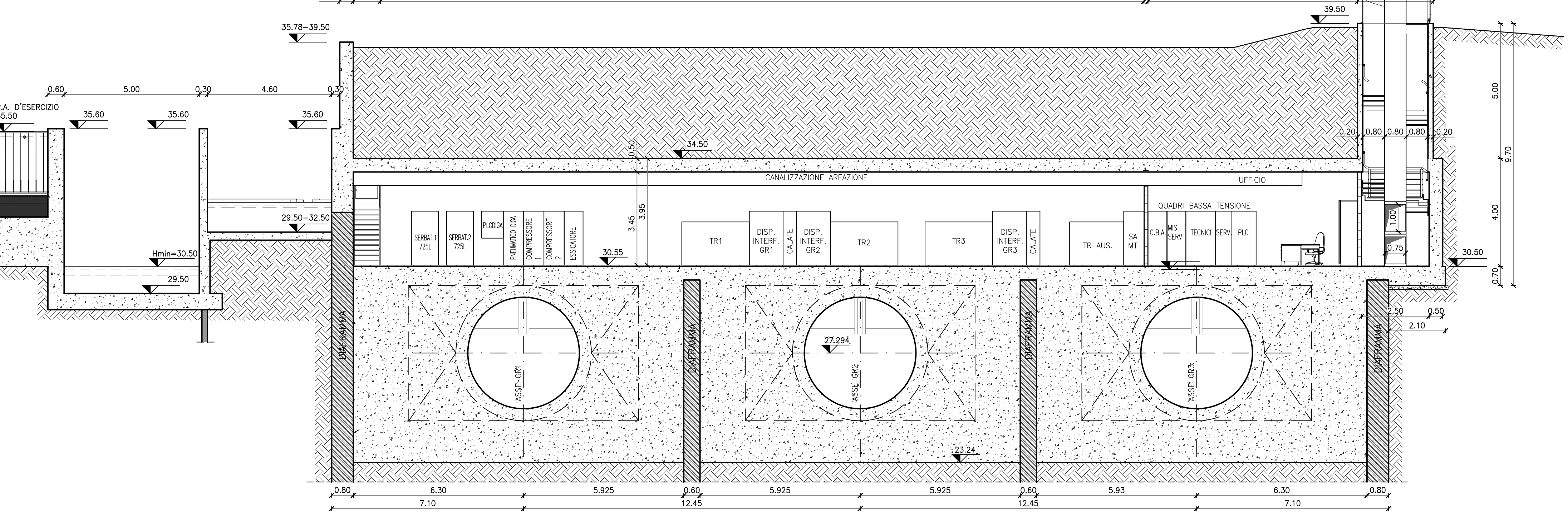
SEZIONE TRASVERSALE C-C 1:100
