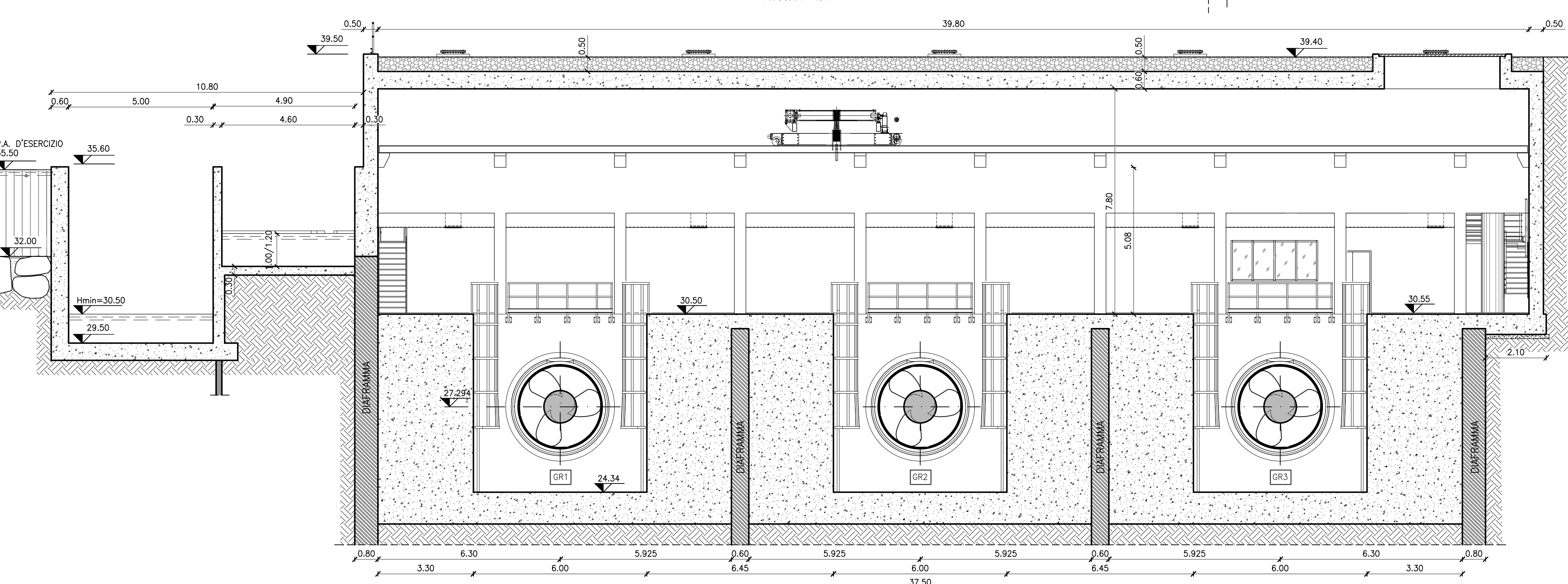
SEZIONE TRASVERSALE B-B 1:100
