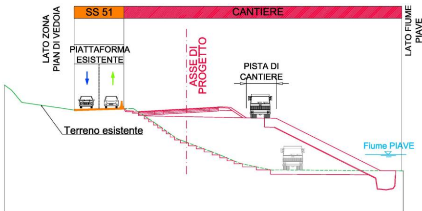
SUBCANTIERE C – MACROFASE 1 – Sezione trasversale di cantierizzazione
