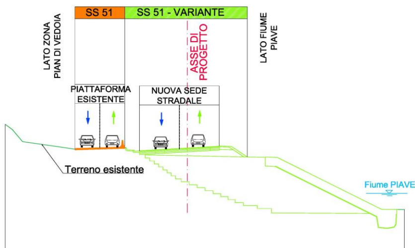
SUBCANTIERE C – MACROFASE 2 - Sezione trasversale di cantierizzazione
