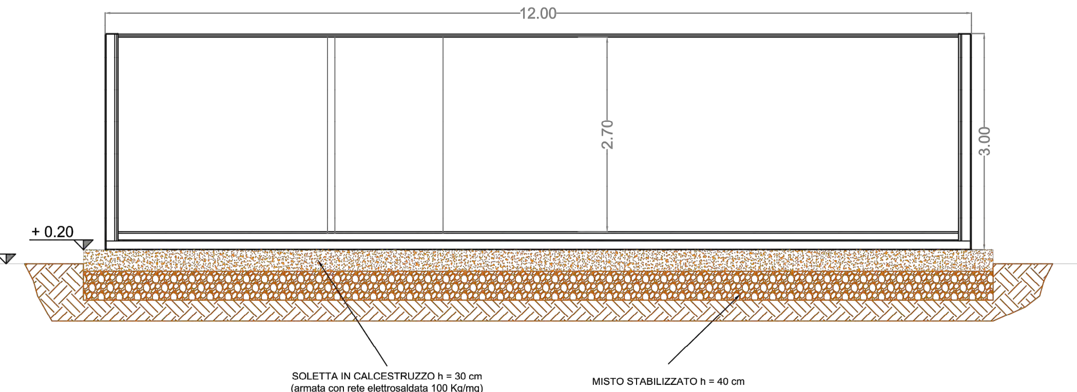
SEAZIONE LONGITUDINALE
