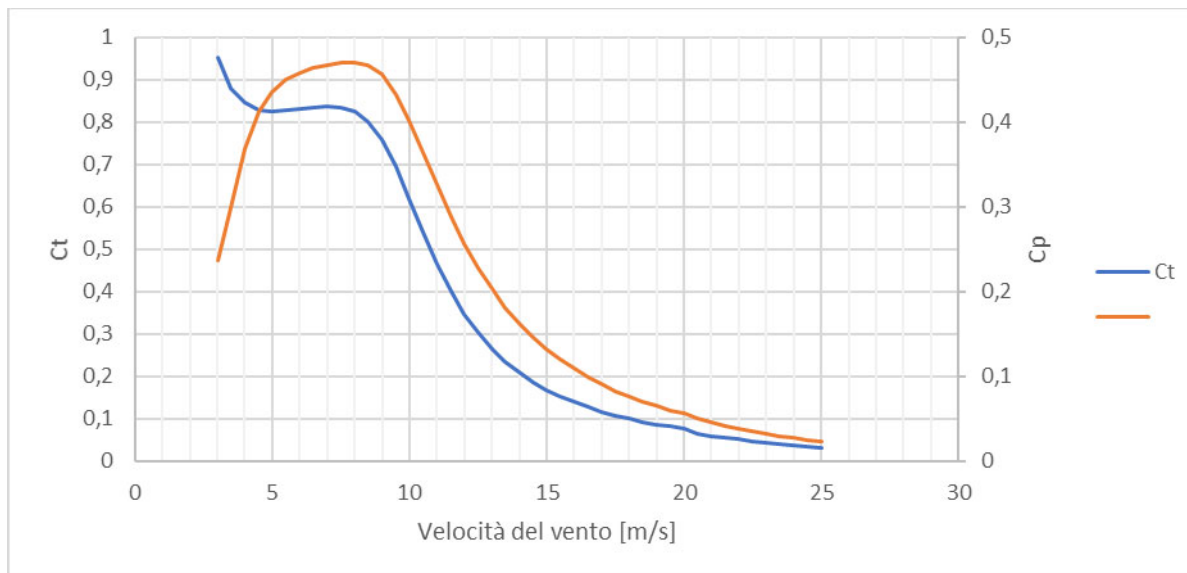
Figura 6 Coefficienti di spinta e di potenza dell'aerogeneratore Siemes Gamesa SG170 da 6,2 MW in funzione della velocità del vento al mozzo in condizioni standard
