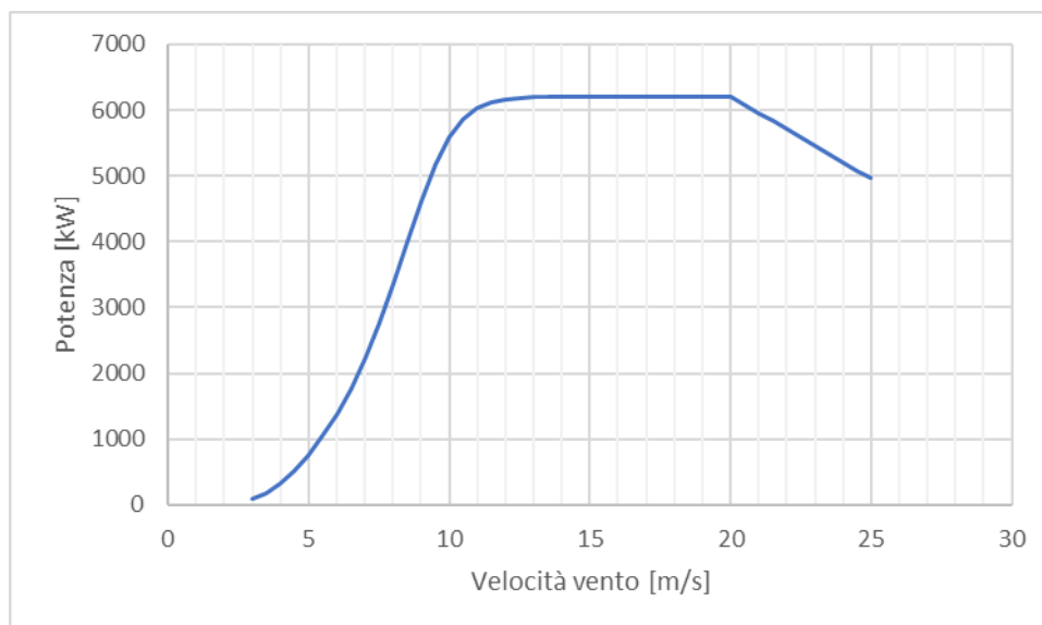
Figura 5 Curva di potenza dell'aerogeneratore Siemens Gamensa SG170 da 6,2 MW in funzione della velocità del vento al mozzo in condizioni standard
