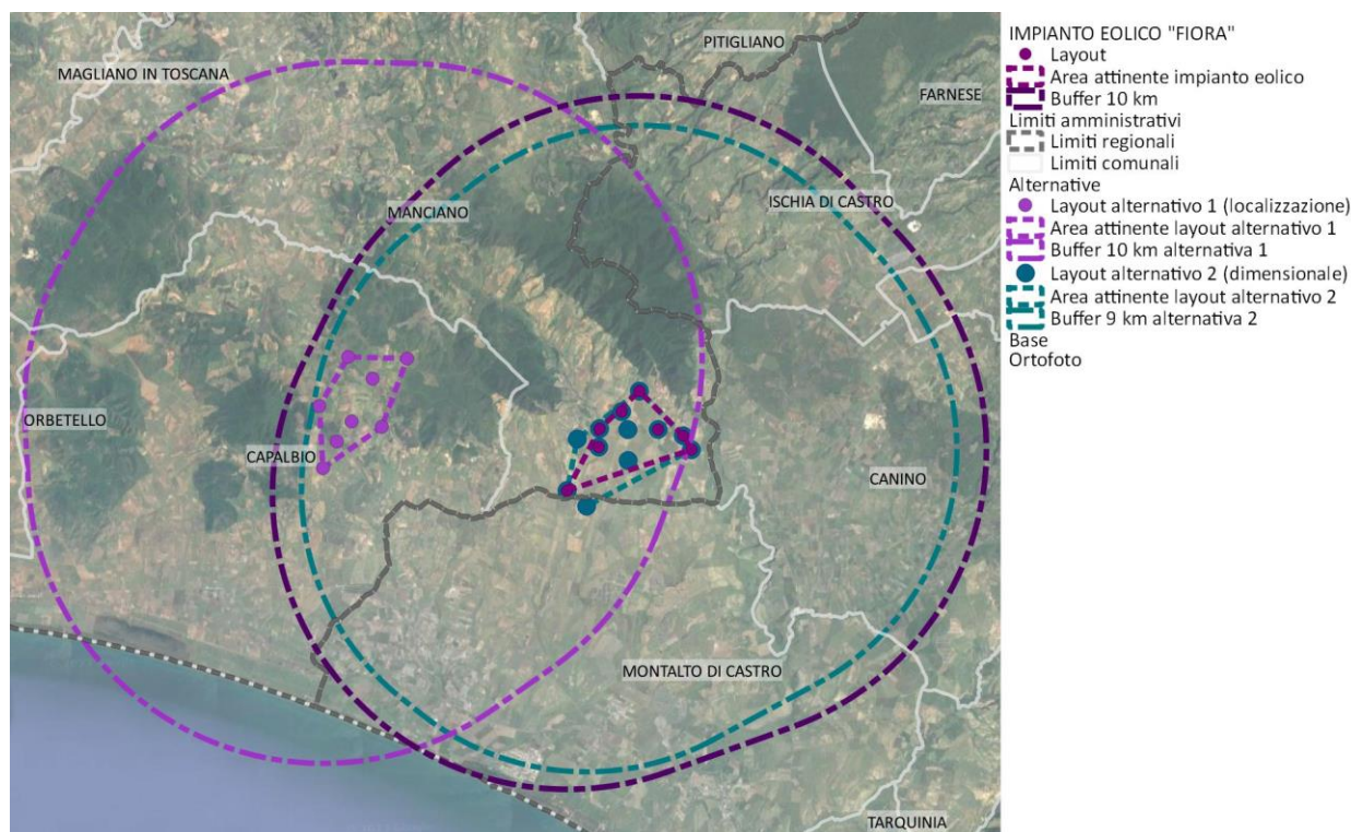
Figura 3. Localizzazione del layout di progetto e dei layout alternativi su base ortofoto
