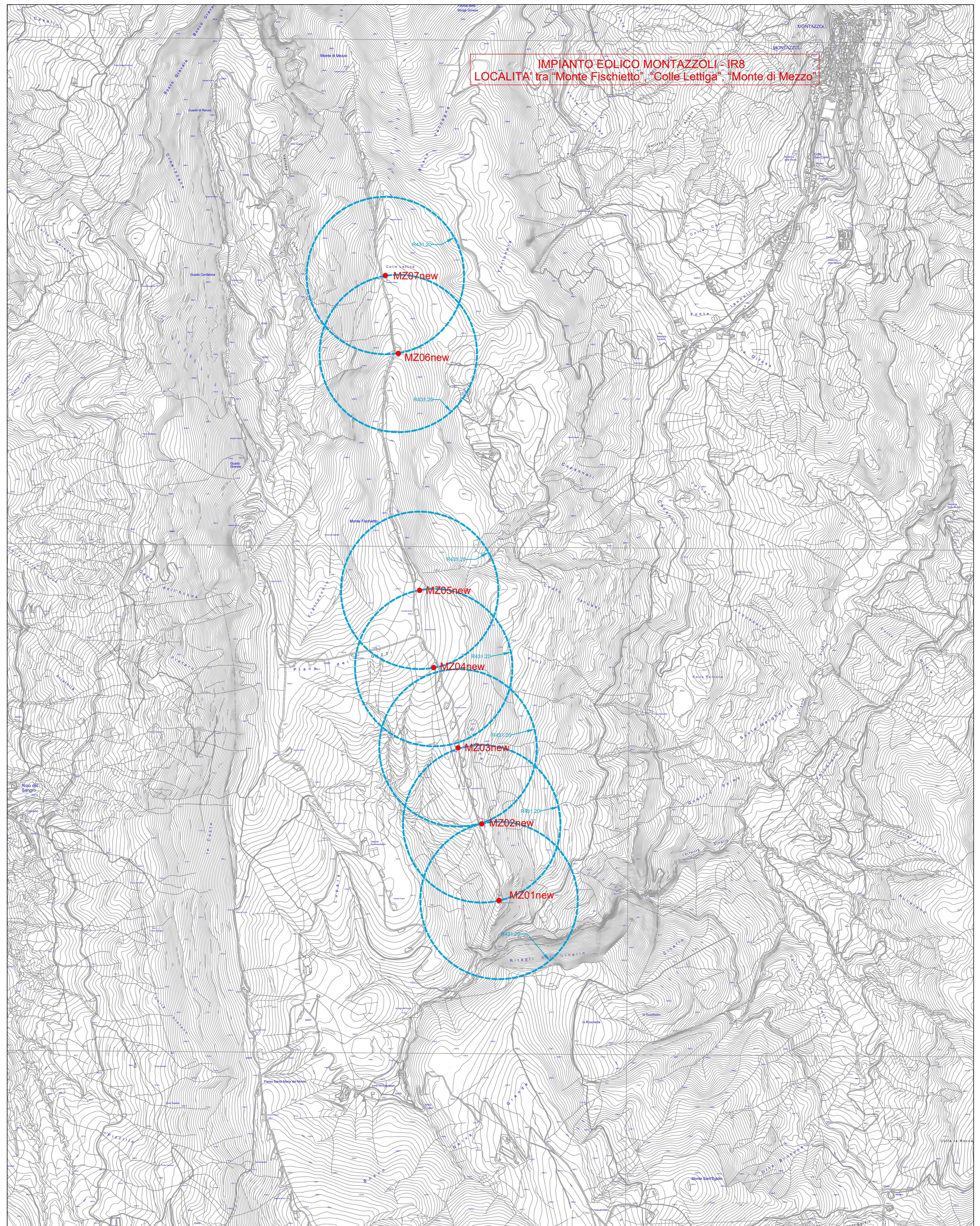
PLANIMETRIA CTR CON CERCHI CONCENTRICI Scala 1:10000
