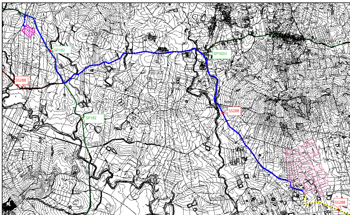
Fig.1.3 - Percorso elettrodotta di collegamento fino alla nuova SST Terna
