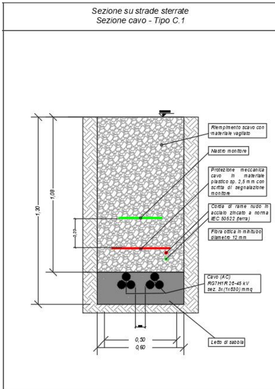
Fig. 3.3.2-1- Doppia Terna di cavi unipolari posati a trifoglio su strada sterrata
