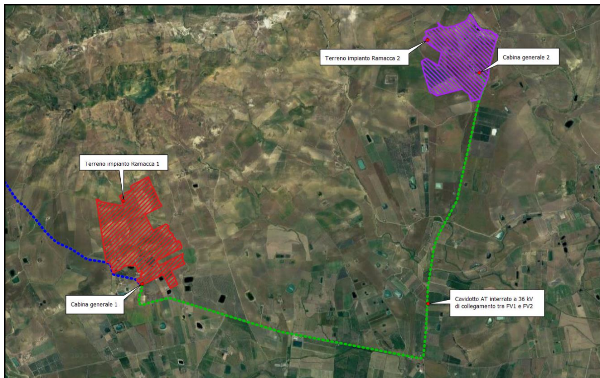
Fig. 1.1 – Planimetria della rete oggetto di studio
