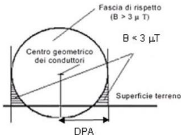
Figura 3.1- Fascia di Rispetto
