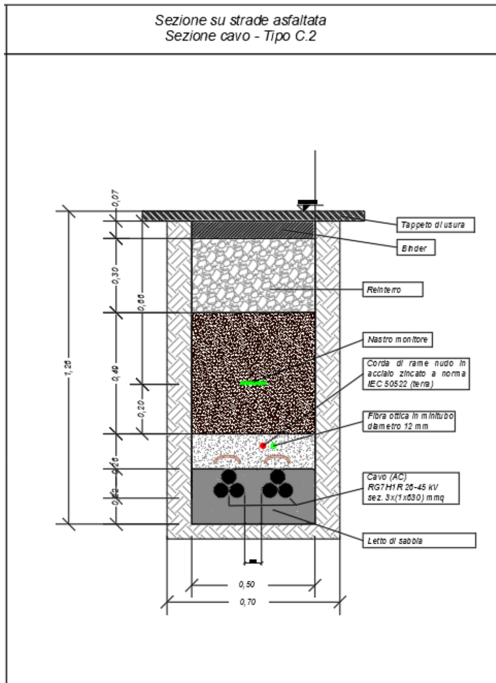
Fig. 3.3.2-2 - Doppia Terna di cavi unipolari posati a trifoglio su strada asfaltata
