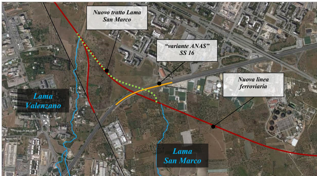
Planimetria dell'attraversamento ferroviario e stradale della Lama Valenzano e della Lama San Marco
