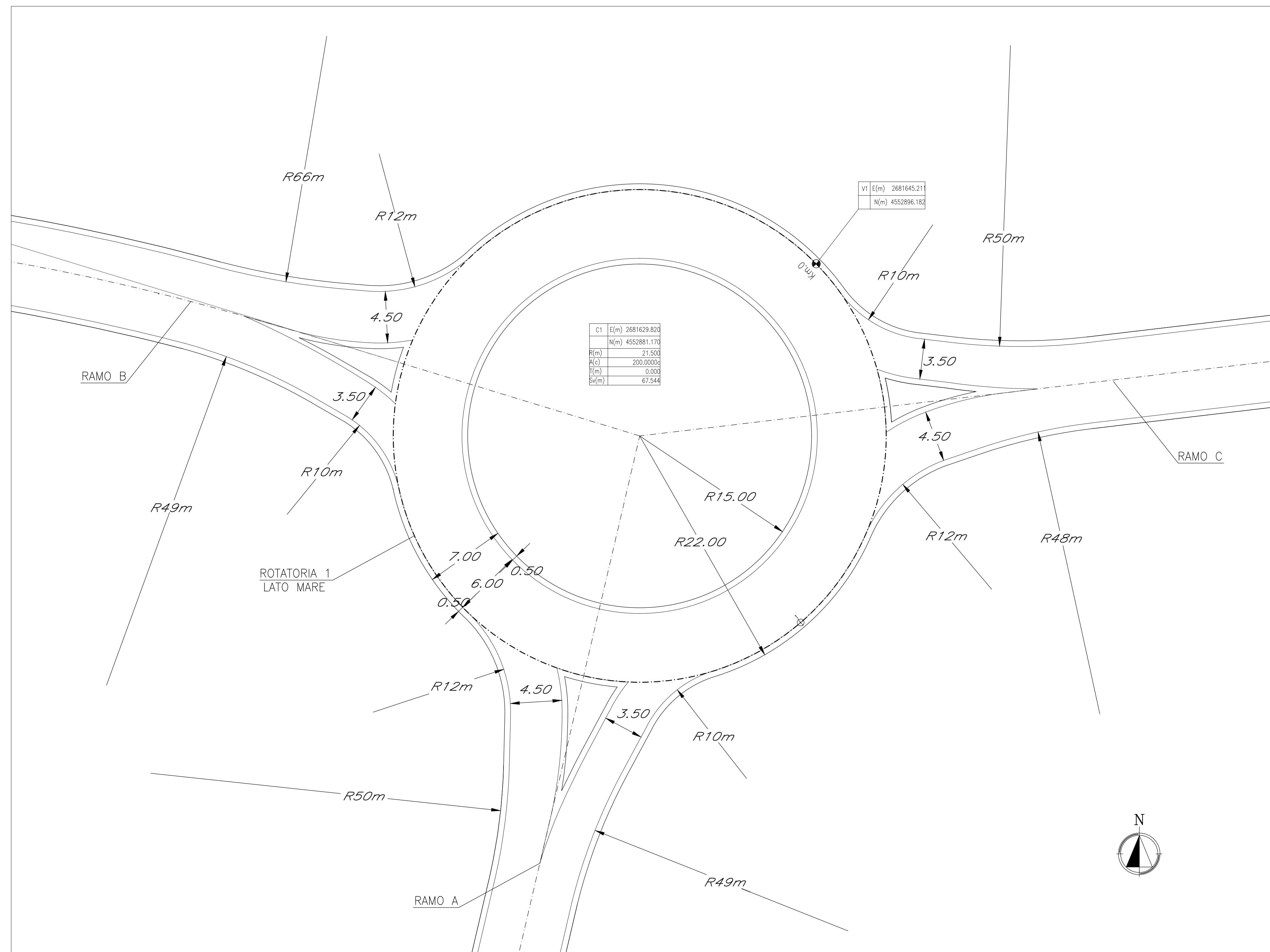
TRACCIAMENTO ROTATORIA 1 "LATO MARE" scala 1:200
