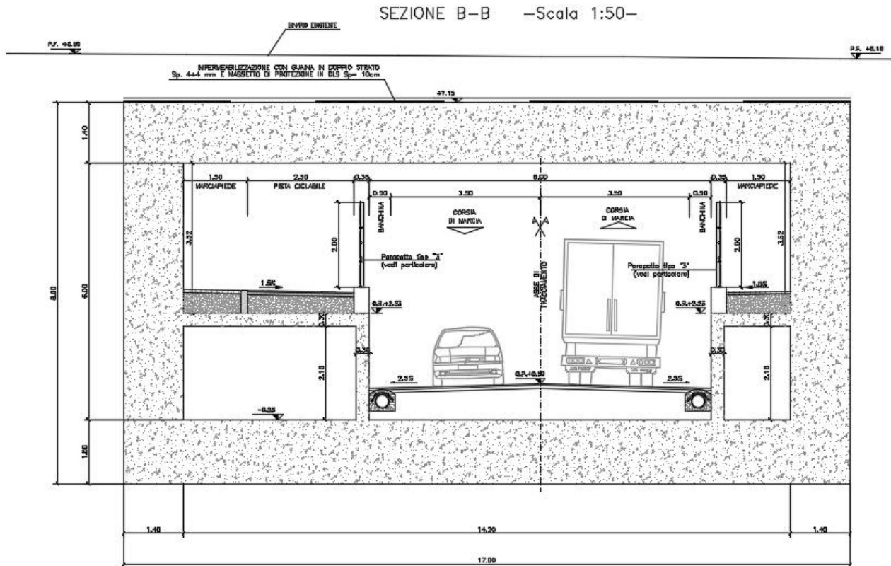
Figura 9. Sezione tipo sottovia
