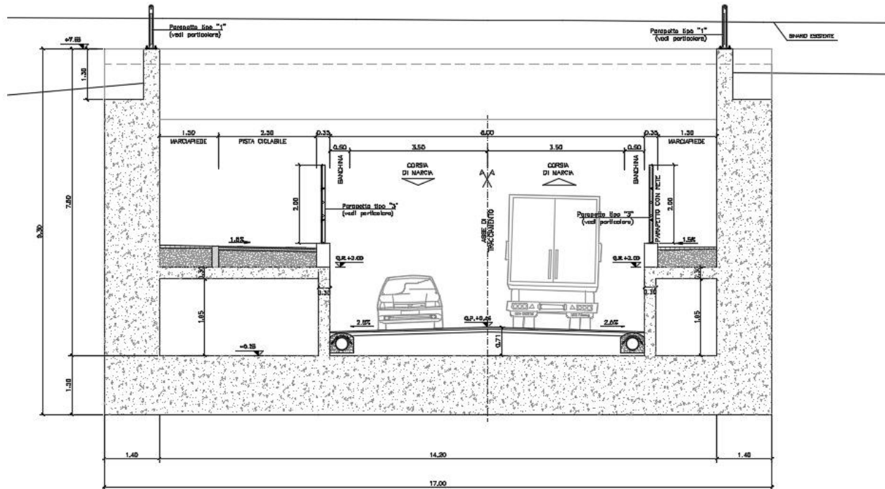
Figura 8. Sezione tipo tra muri
