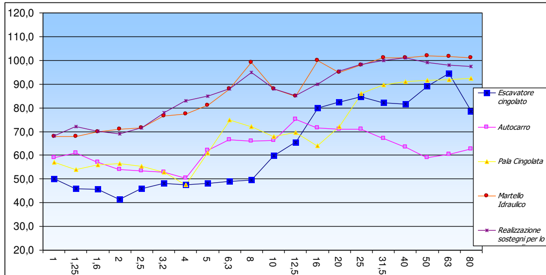
Figura 60. Spettri di sorgente dei macchinari da cantiere, misurati a distanza nota dalla sorgente
