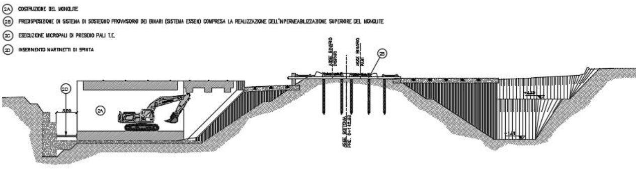
Figura 10. Sistema di sostegno del binario Essen
