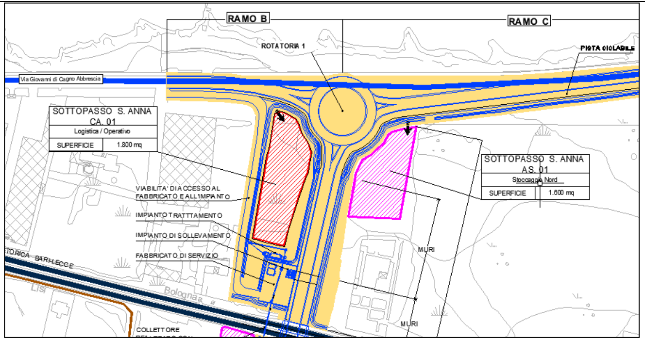
Vista planimetrica dell'area CA.01 con posizionamento del tracciato
