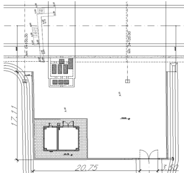
Figura 11. planimetria posizionamento del F.T.
