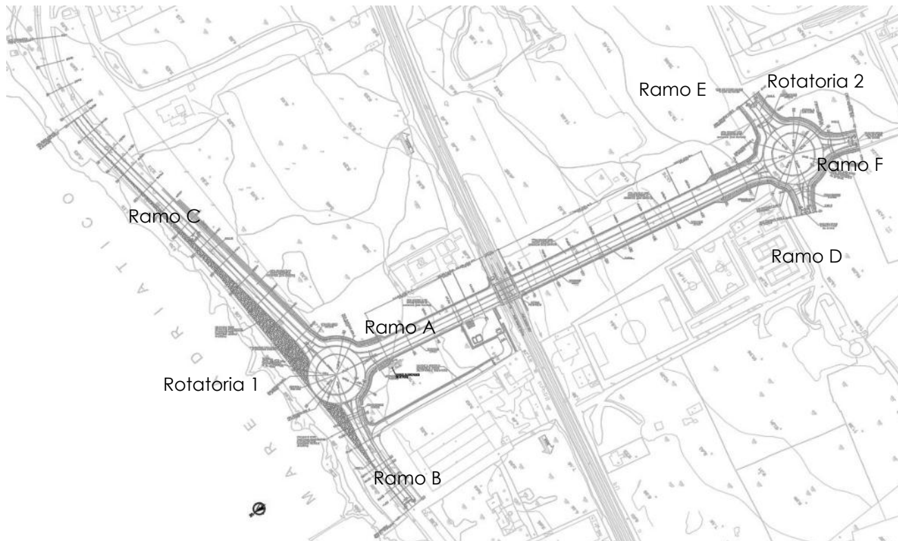
Figura 6. Planimetria di progetto
