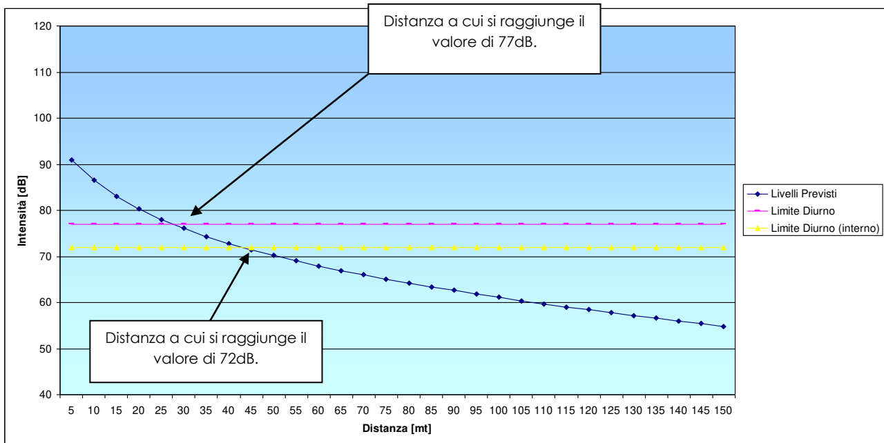
Figura 64. Livelli di accelerazione complessiva in dB stimati durante la fase palificazione Considerata la vicinanza del ricevitore individuato ed identificato in area 4 rispetto all'area di cantiere, si suggerisce di monitorare la componente vibrazione presso tale punto.
