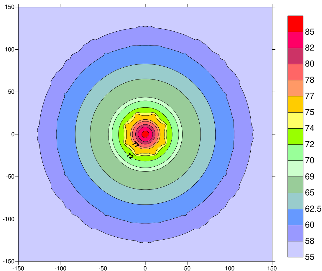
Figura 61. Livelli di accelerazione ponderata complessiva in dB stimati durante la fase di scavo e movimentazioni materiali
