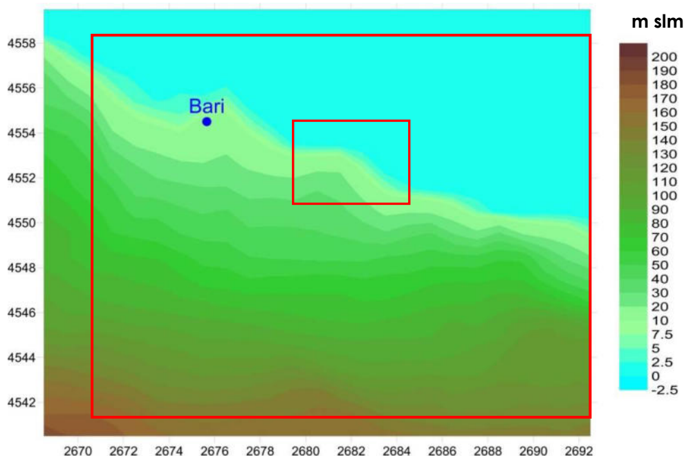
Figura 43. Orografia del dominio di calcolo meteorologico, con indicazione dei sottodomini di calcolo per la dispersione degli inquinanti nelle varie simulazioni.
