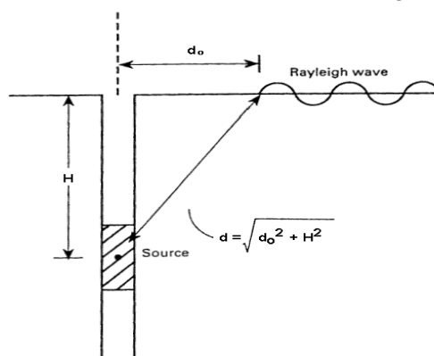
Figura 59– Schema della propagazione a partire da una sorgente profonda
