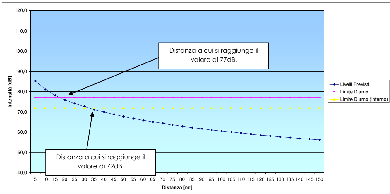
Figura 63. Livelli di accelerazione complessiva in dB stimati durante la fase di scavo e movimentazione materiali all'interno del cantiere
