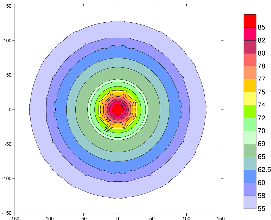
Figura 62. Livelli di accelerazione ponderata complessiva in dB stimati durante la fase di demolizione all'interno del cantiere – palificazione
