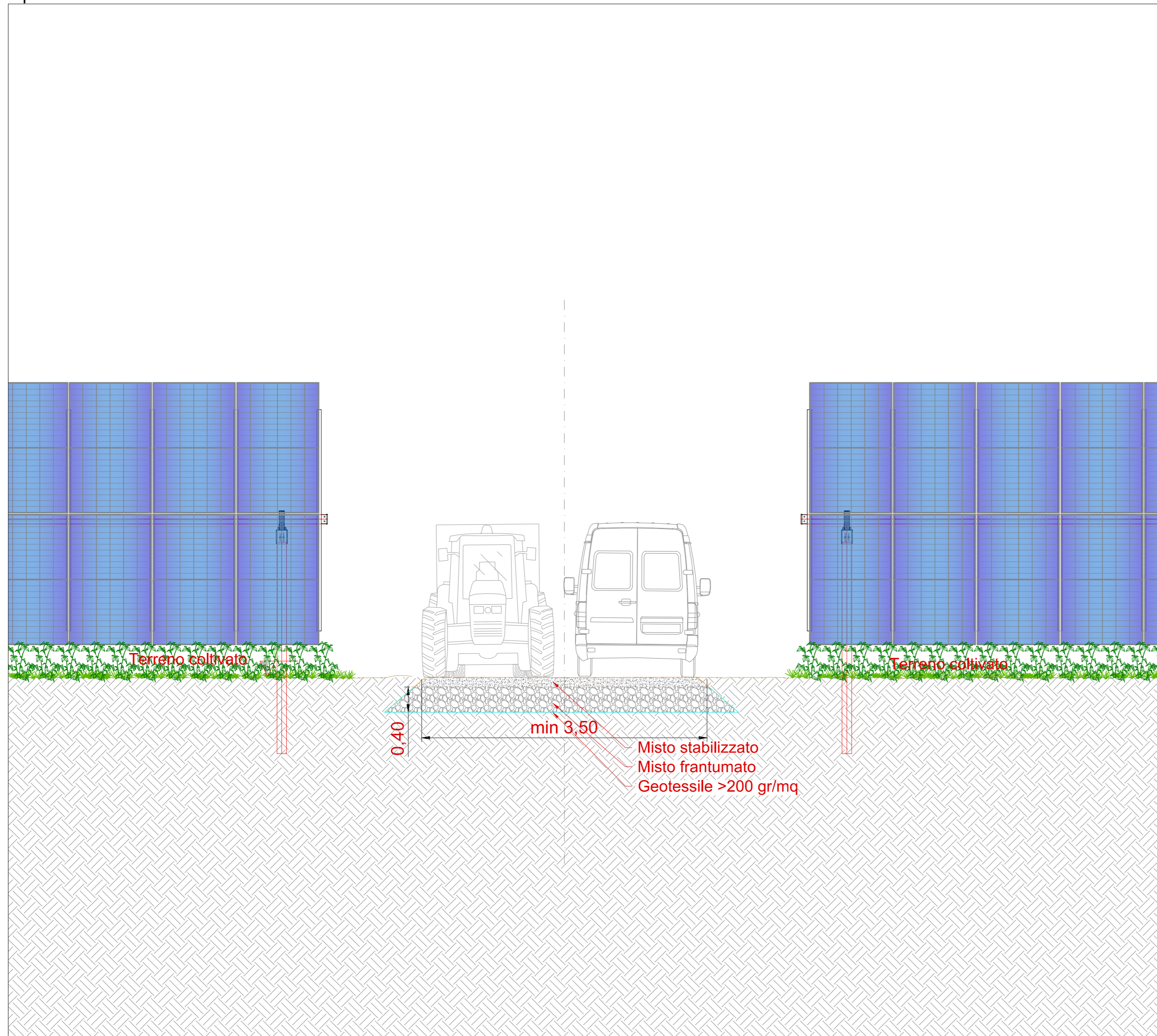
Tipico strada interna - scala 1:50
