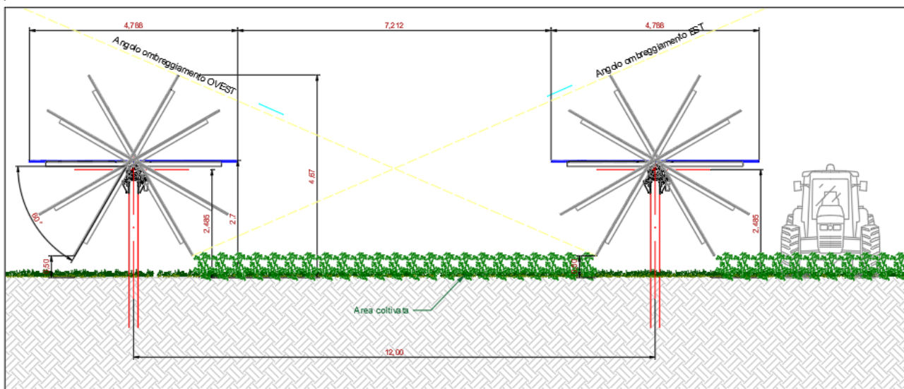
Figura 5.3 – Disposizione delle strutture di sostegno dei moduli fotovoltaici
