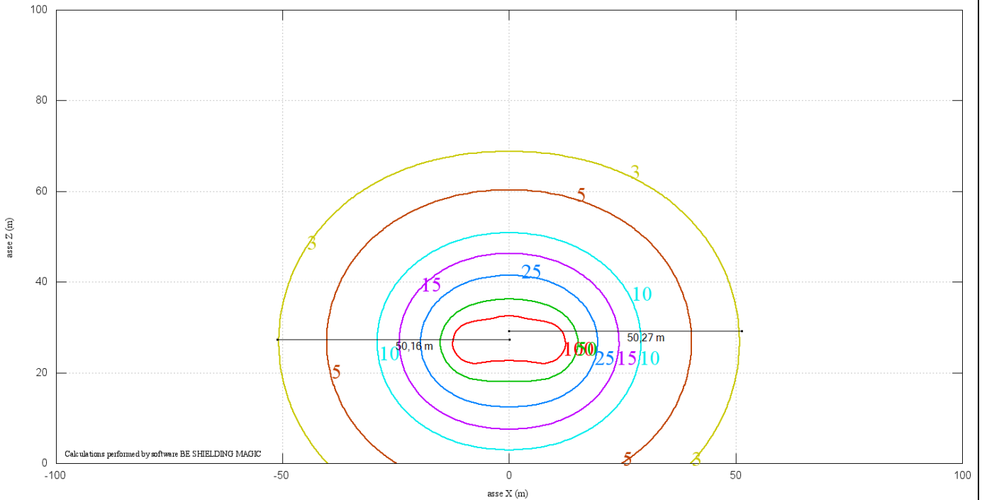
Figura 4 – Livelli di campo magnetico prodotti dalla configurazione dei conduttori su sostegno a Y con angolo
