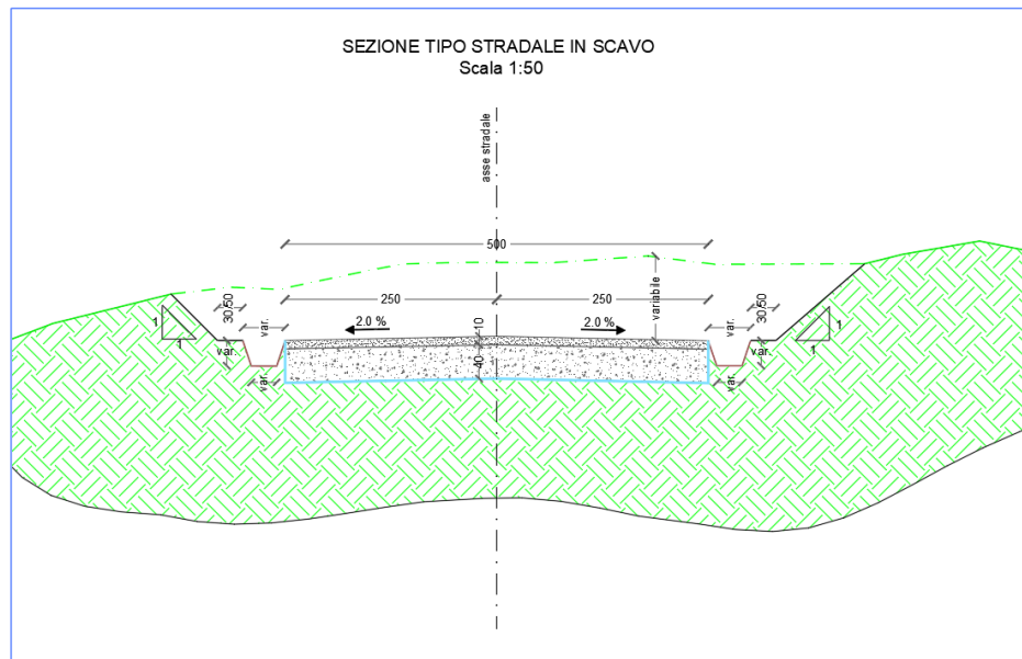
Fig 2: Sezione tipo di strada in scavo
