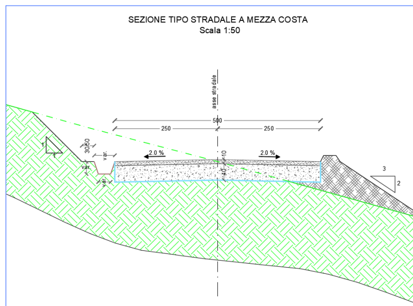
Fig 3: Sezione tipo di strada a mezzacosta
