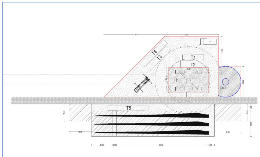
Schema tipo piazzola
