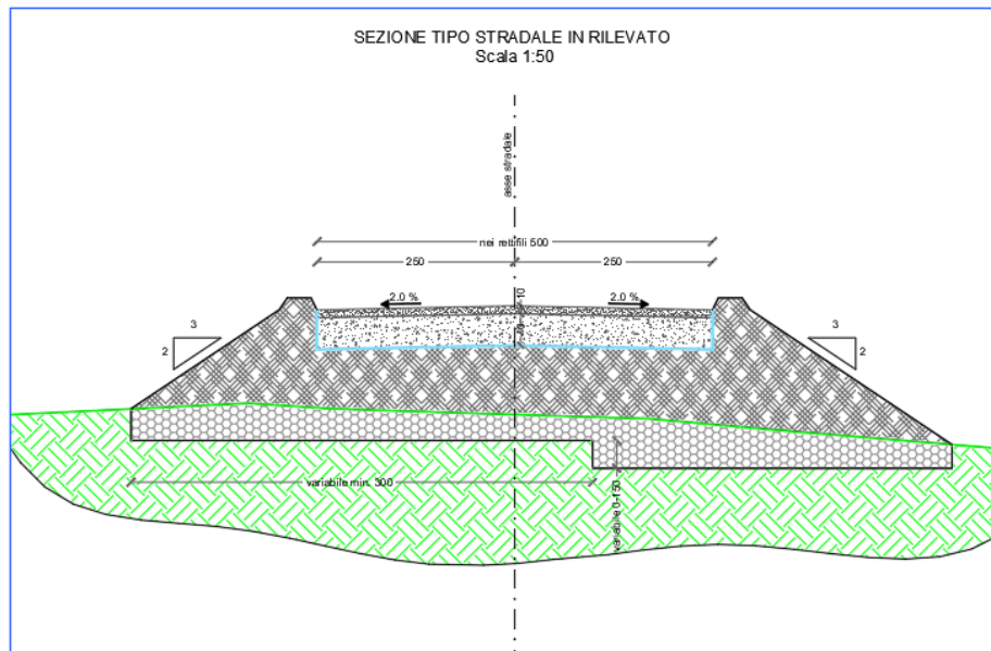
Fig 4: Sezione tipo di strada in rilevato
