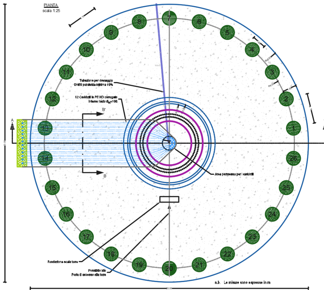
Fig.1 Tipologia della fondazione su pali prevista
