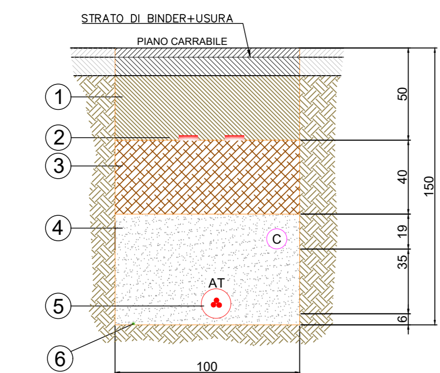
TIPOLOGICO SEZIONE CAVIDOTTO INTERRATO SU STRADA ASFALTATA SCALA 1:20
