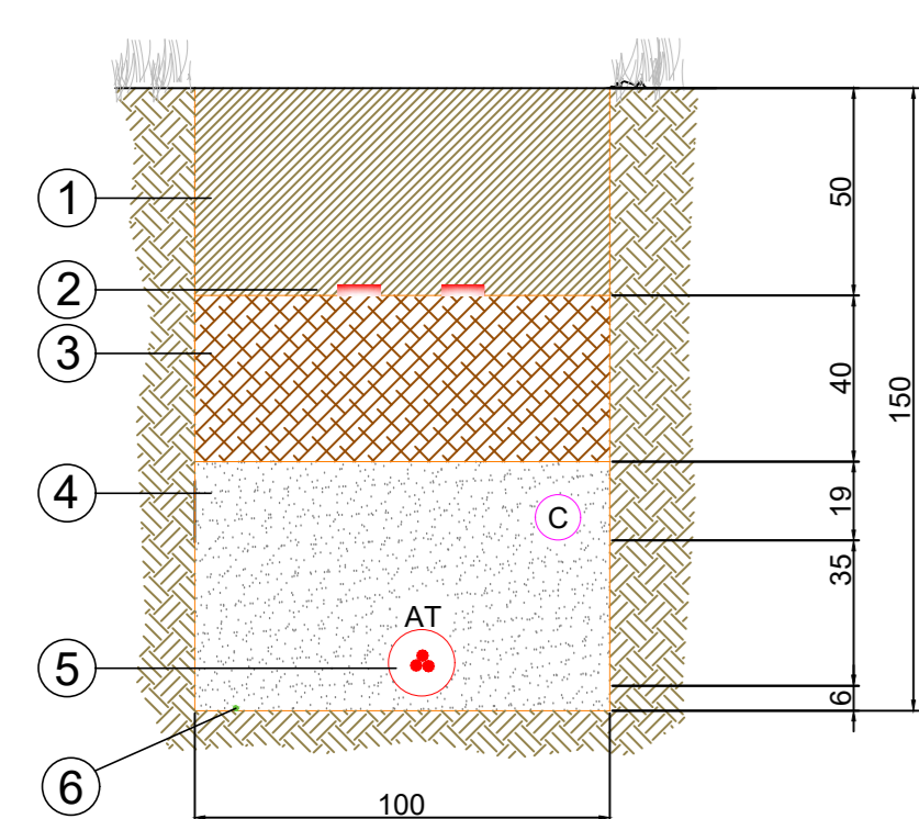
TIPOLOGICO SEZIONE CAVIDOTTO INTERRATO SU STRADA BIANCA SCALA 1:20
