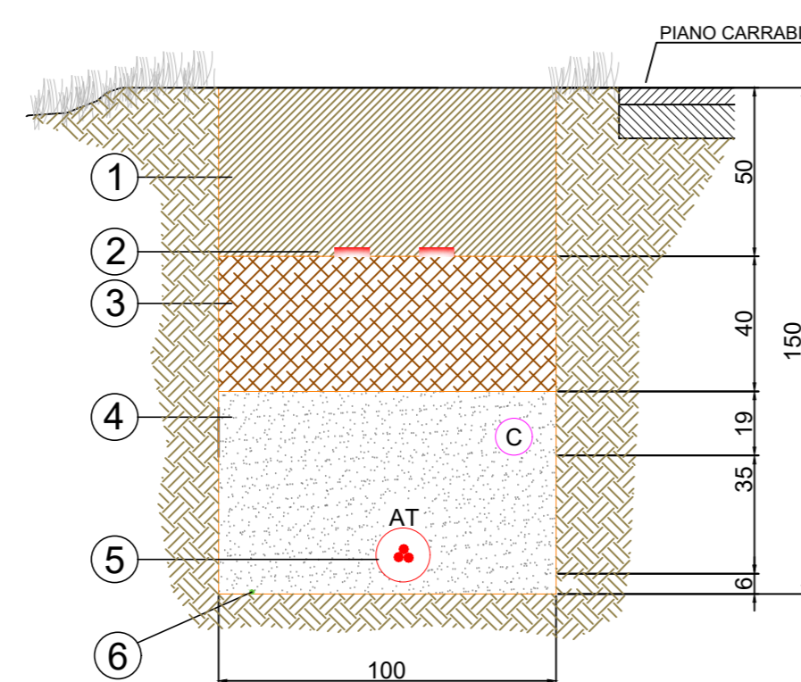
TIPOLOGICO SEZIONE CAVIDOTTO INTERRATO IN BANCHINA SCALA 1:20
