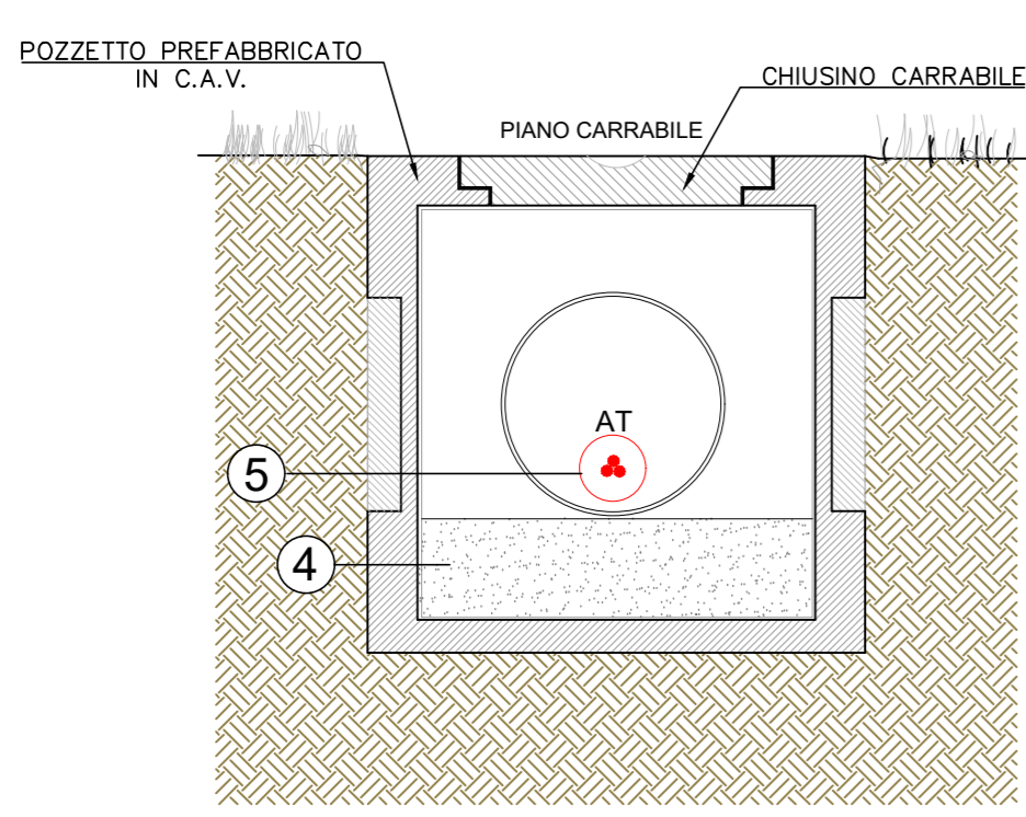
TIPOLOGICO SEZIONE CAVIDOTTO INTERRATO POZZETTO DI ISPEZIONE SCALA 1:20
