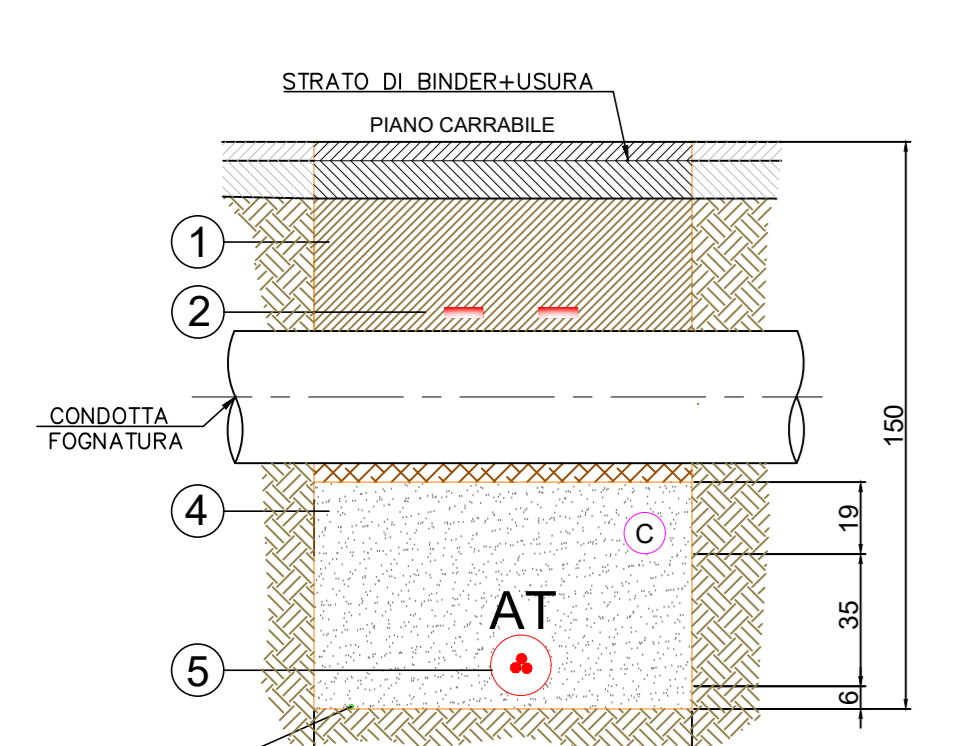
TIPOLOGICO SEZIONE CAVIDOTTO INTERRATO SUPERAMENTO FOGNATURA SCALA 1:20
