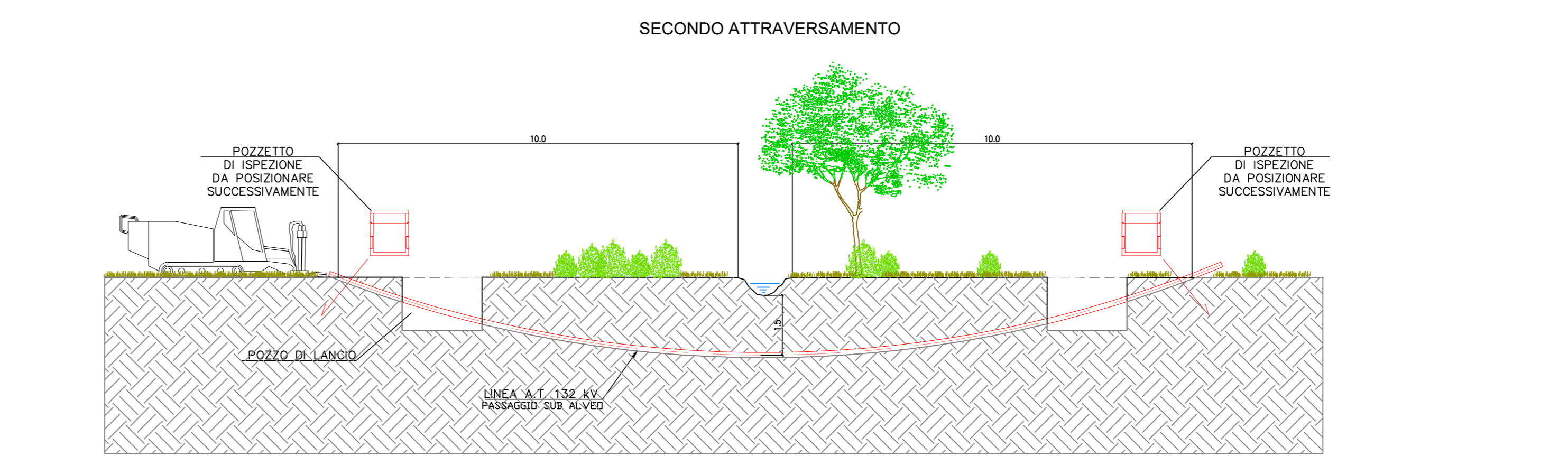
TIPOLOGICO ATTRAVERSAMENTO - SUB ALVEO CON TECNICA NO-DIG SCALA 1:100
