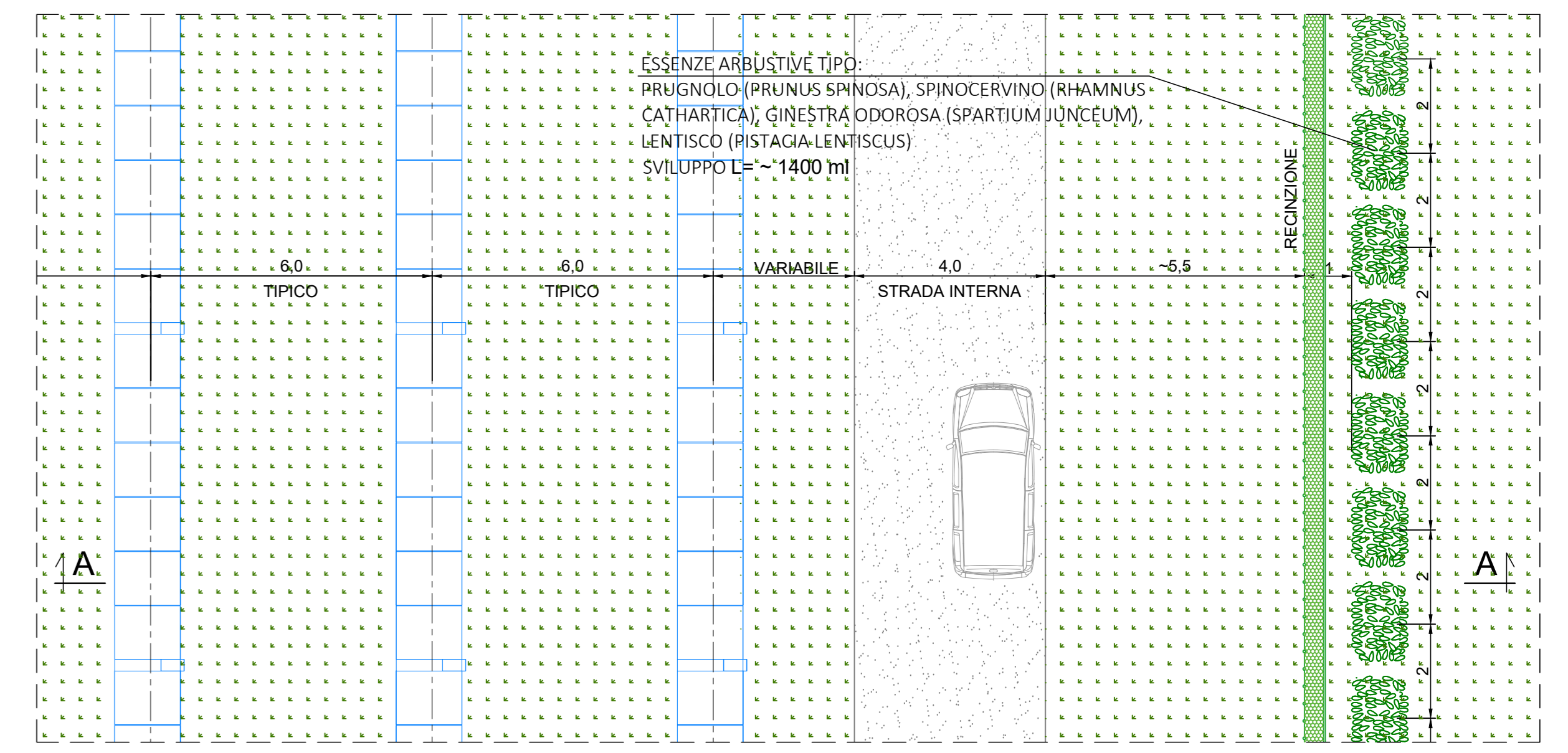
DETT. "1" VISTA IN PIANTE OPERE DI MITIGAZIONE INTERPOSTE TRA CAMPO F.V. E S.P. 67 DI CAMPIGNOLA Scala 1:100
