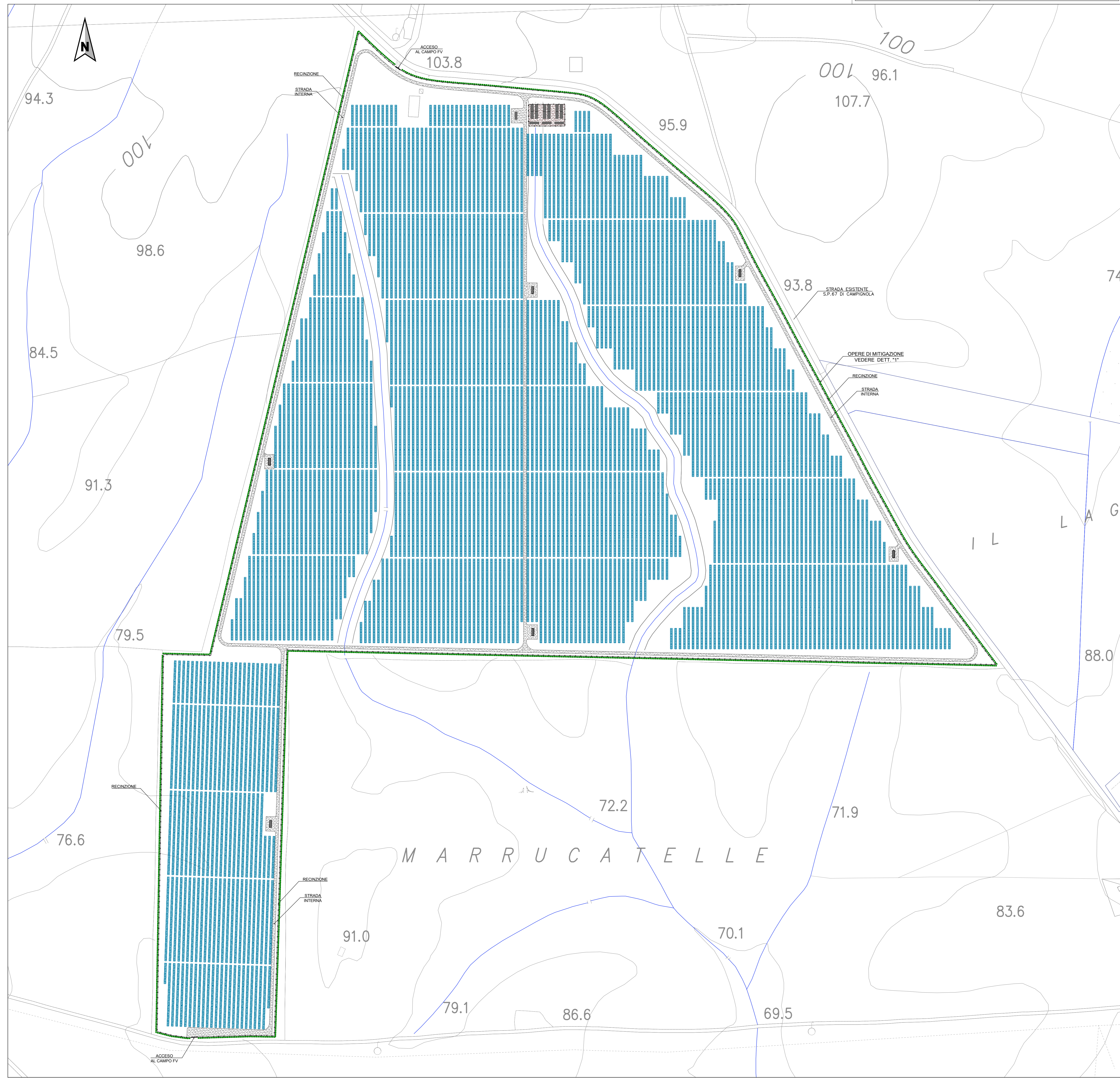
ESTRATTO PLANIMETRICO ZONA IMPIANTO FV Scala 1:2000
