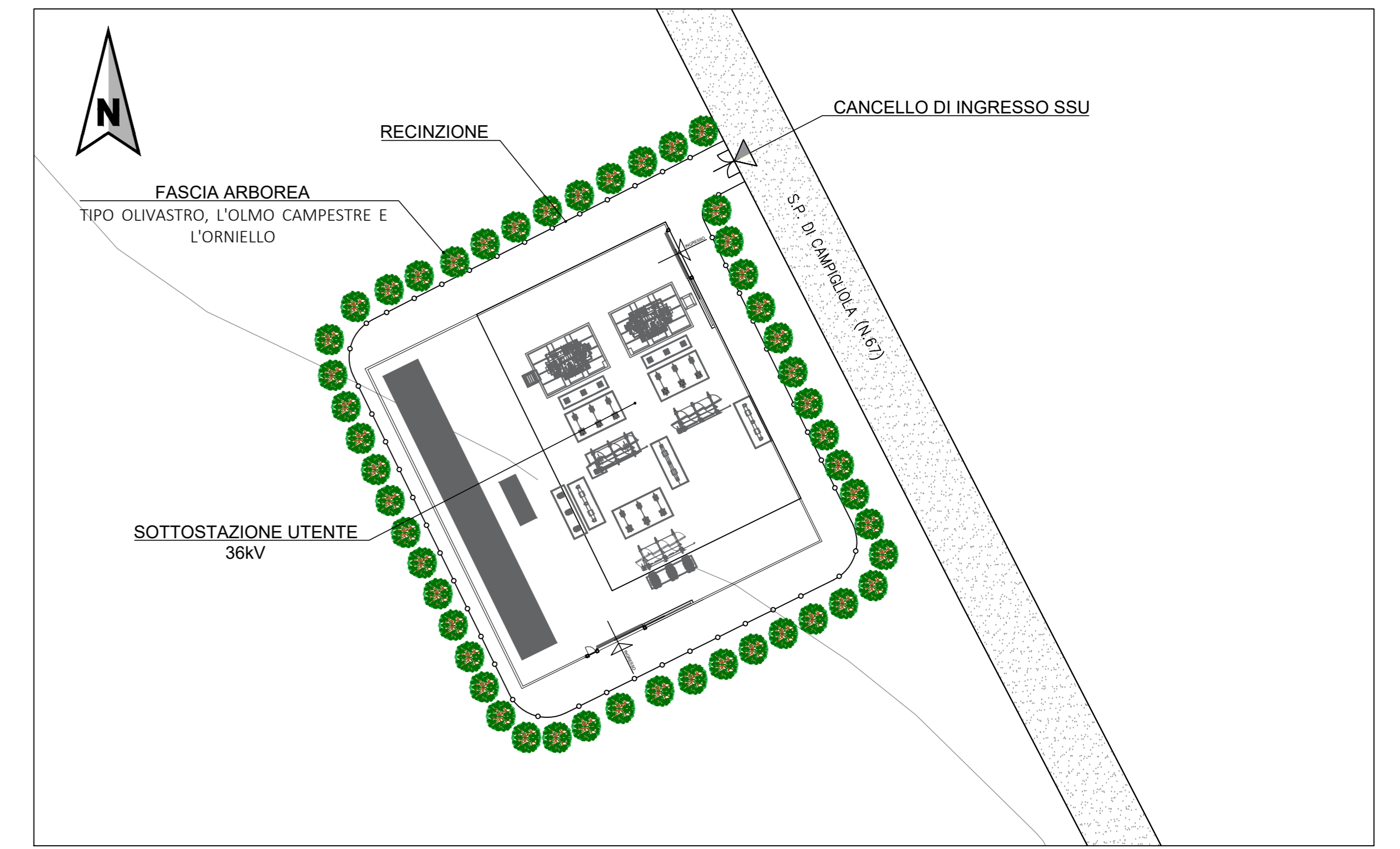
ESTRATTO PLANIMETRICO ZONA SOTTOSTAZIONE UTENTE 36kV Scala 1:500
