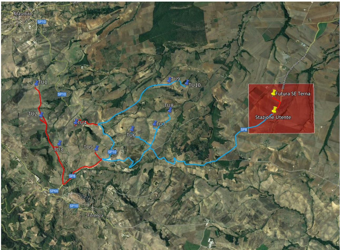
Figura 11 – Localizzazione della Stazione utente (1/2) Coordinate WGS84 UTM33 Stazione Utente: 577830 E; 4526367 N
