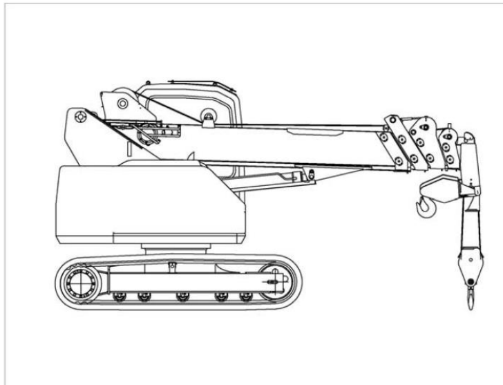
Figura 5 - Gru cingolata
