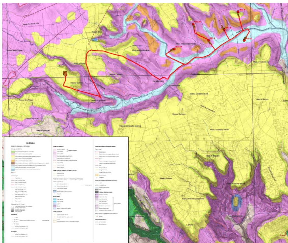
Figura 3 - Inquadramento su Carta Idrogeomorfologica
