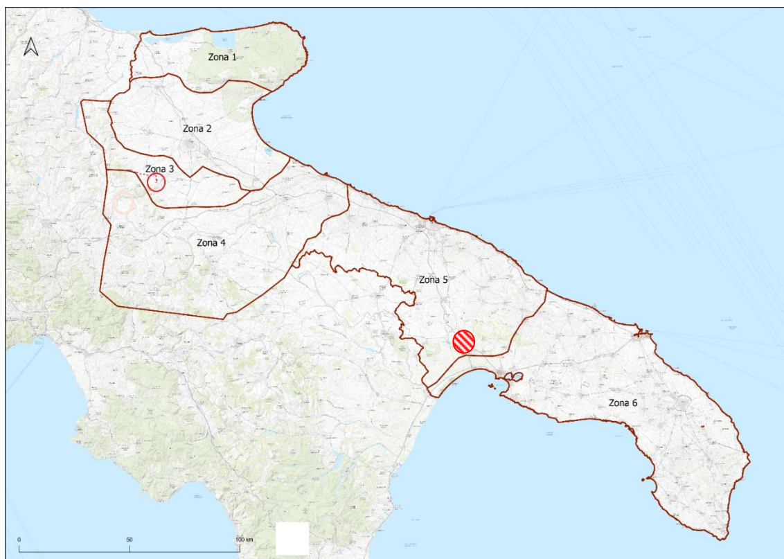
Figura 4 - Livello di regionalizzazione della Regione Puglia
