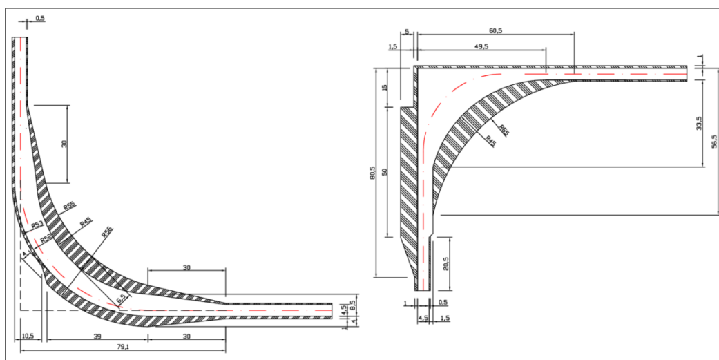
Figura 11 - Particolare realizzazione raccordo strade
