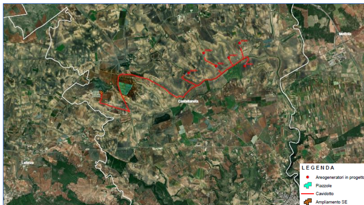
Figura 5 - layout impianto definitivo a n.6 aerogeneratori
