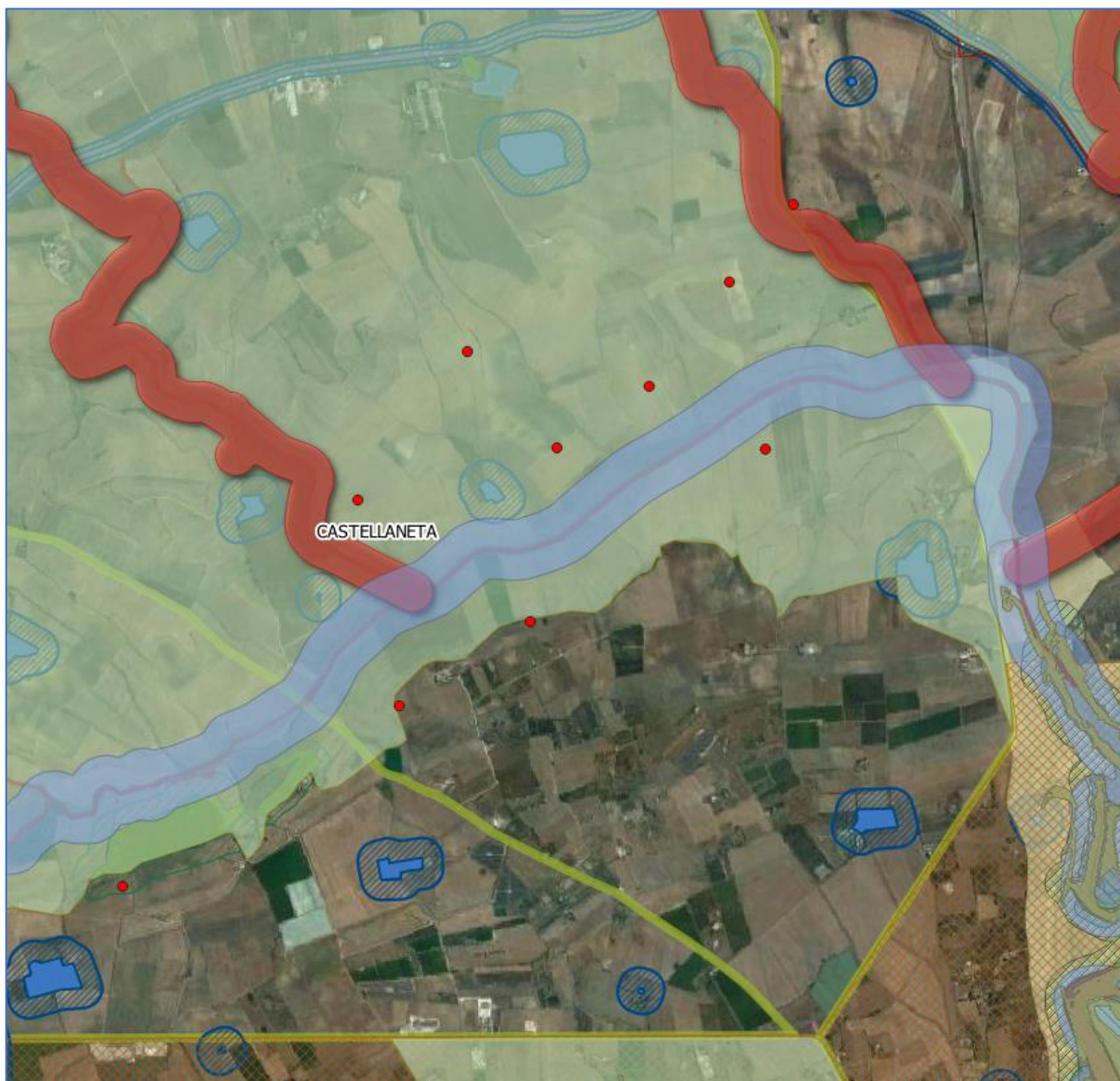
Figura 4 - Ipotesi di layout a 10 aerogeneratori - analisi vincolistica e buffer dai canali
