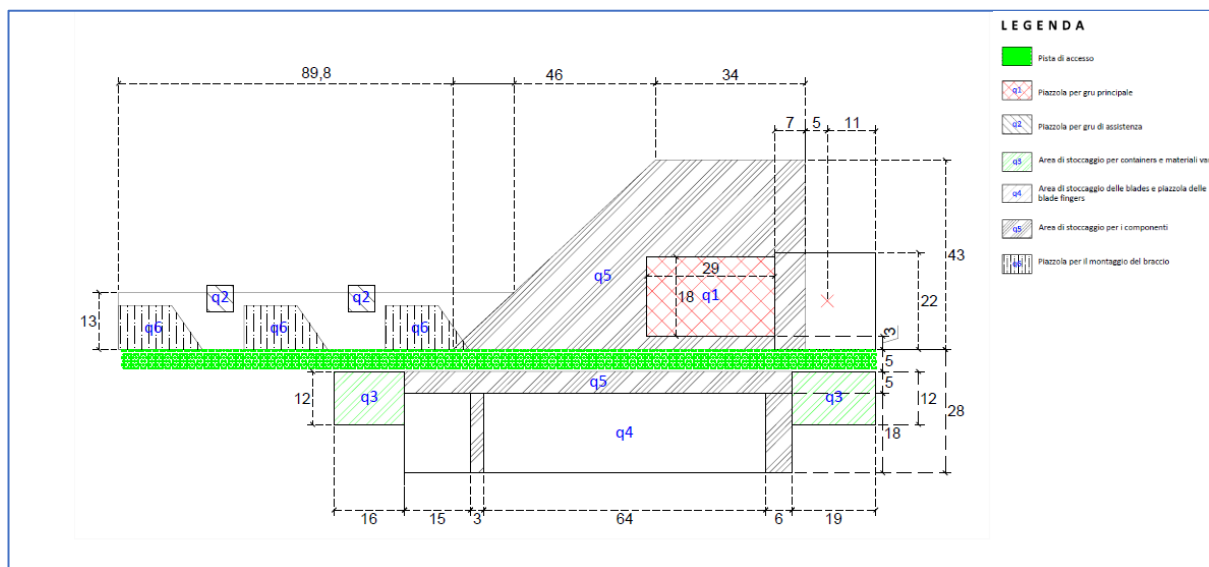
Figura 15 – tipologica della piazzola di montaggio
