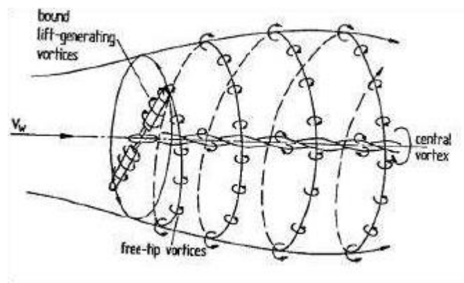
Figura 9 - Vortici e scia
