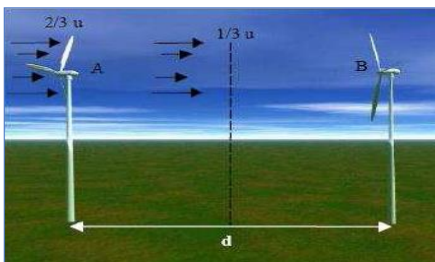
Figura 8 - Effetto di schiera
