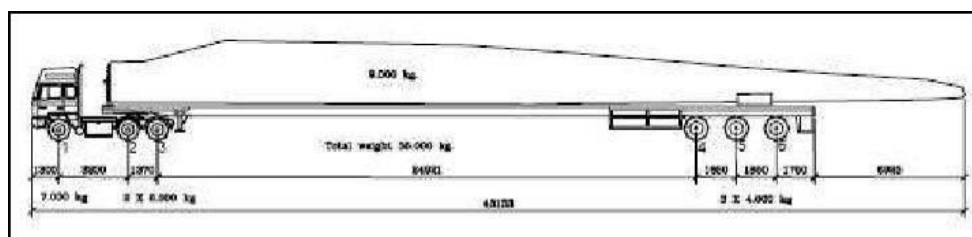
Figura 12 - Dimensioni autoarticolato
