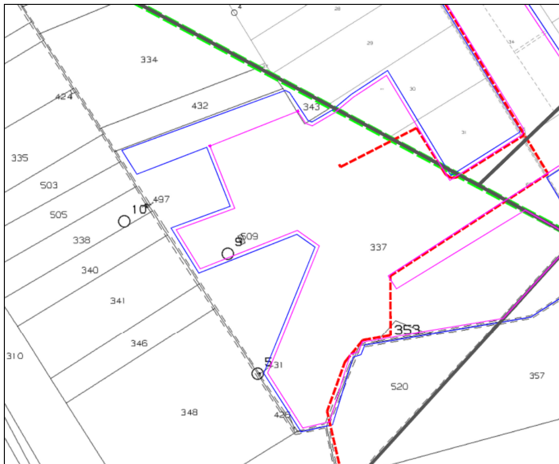
Figura 4: Stralcio catastale progetto agrivoltaico "Orta Nova"
