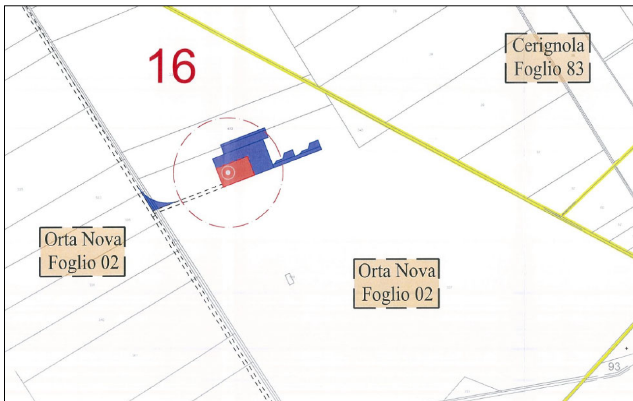
Figura 3: Stralcio catastale progetto eolico "Lampino" – aerogeneratore 16
