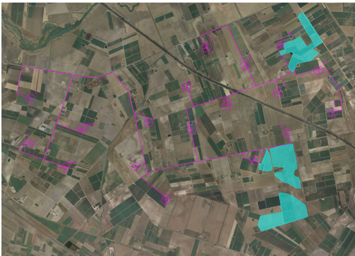
Figura 1: Evidenza dell'interferenza tra parco agrivoltaico "Orta Nova" e parco eolico "Lampino" (la cui istanza è anteriore)
