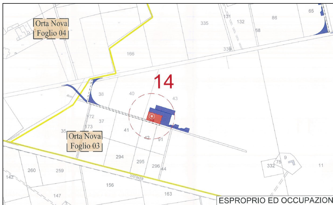
Figura 5: Stralcio catastale progetto eolico "Lampino"- aerogeneratore 14
