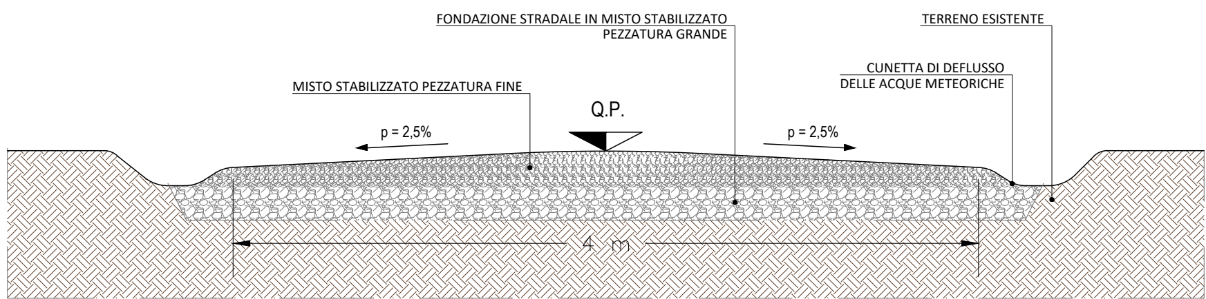
Stratigrafia della viabilità interna - Scala 1:20
