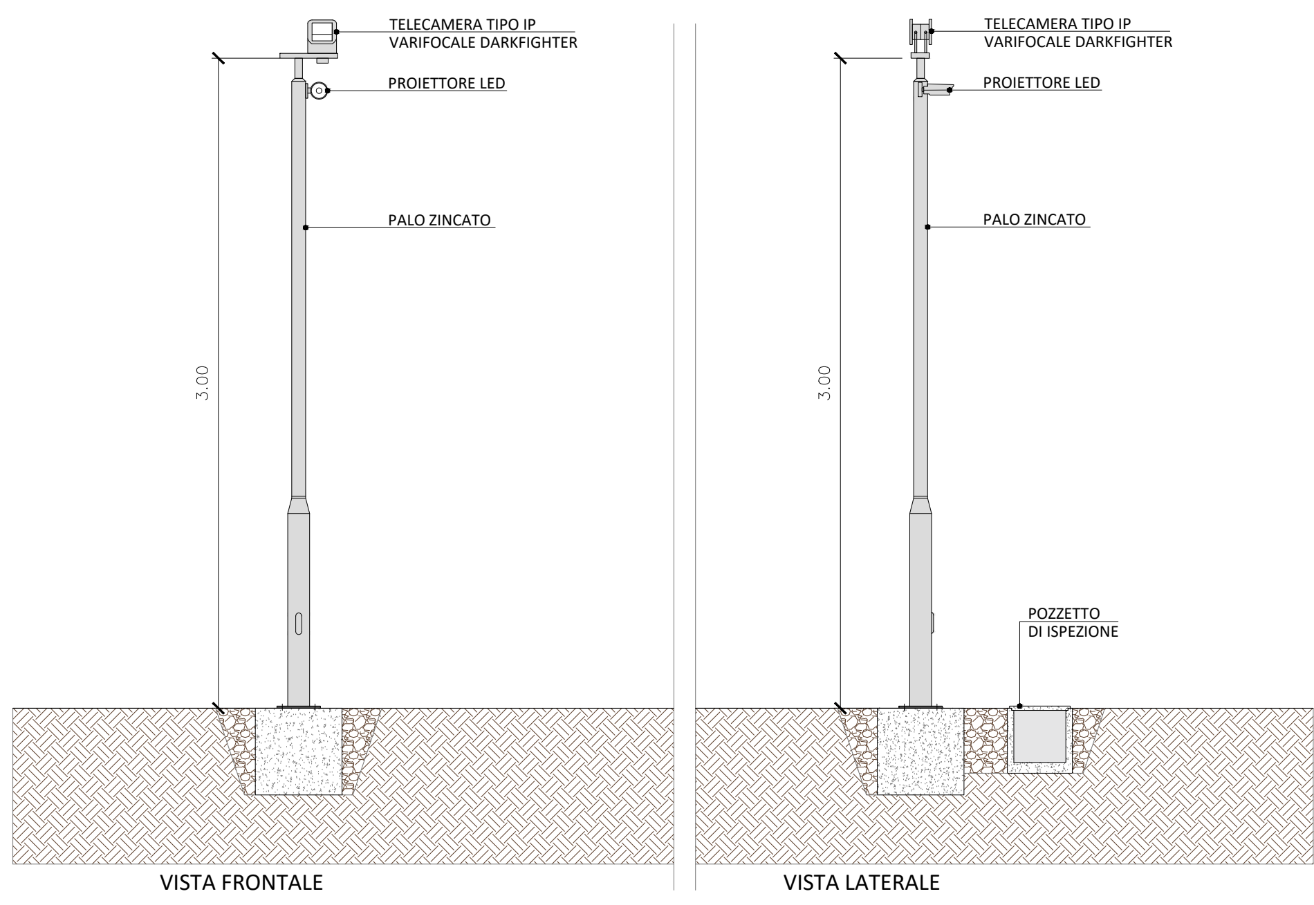
PALO ILLUMINAZIONE E VIDEOSORVEGLIANZA
