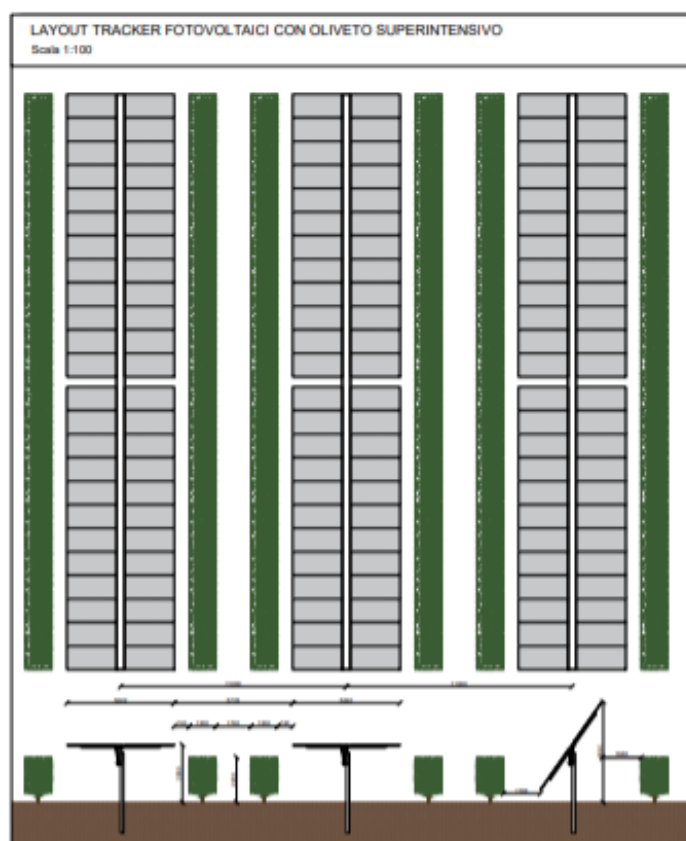
Figura 8 - Particolare disposizione dei pannelli ed olivi
