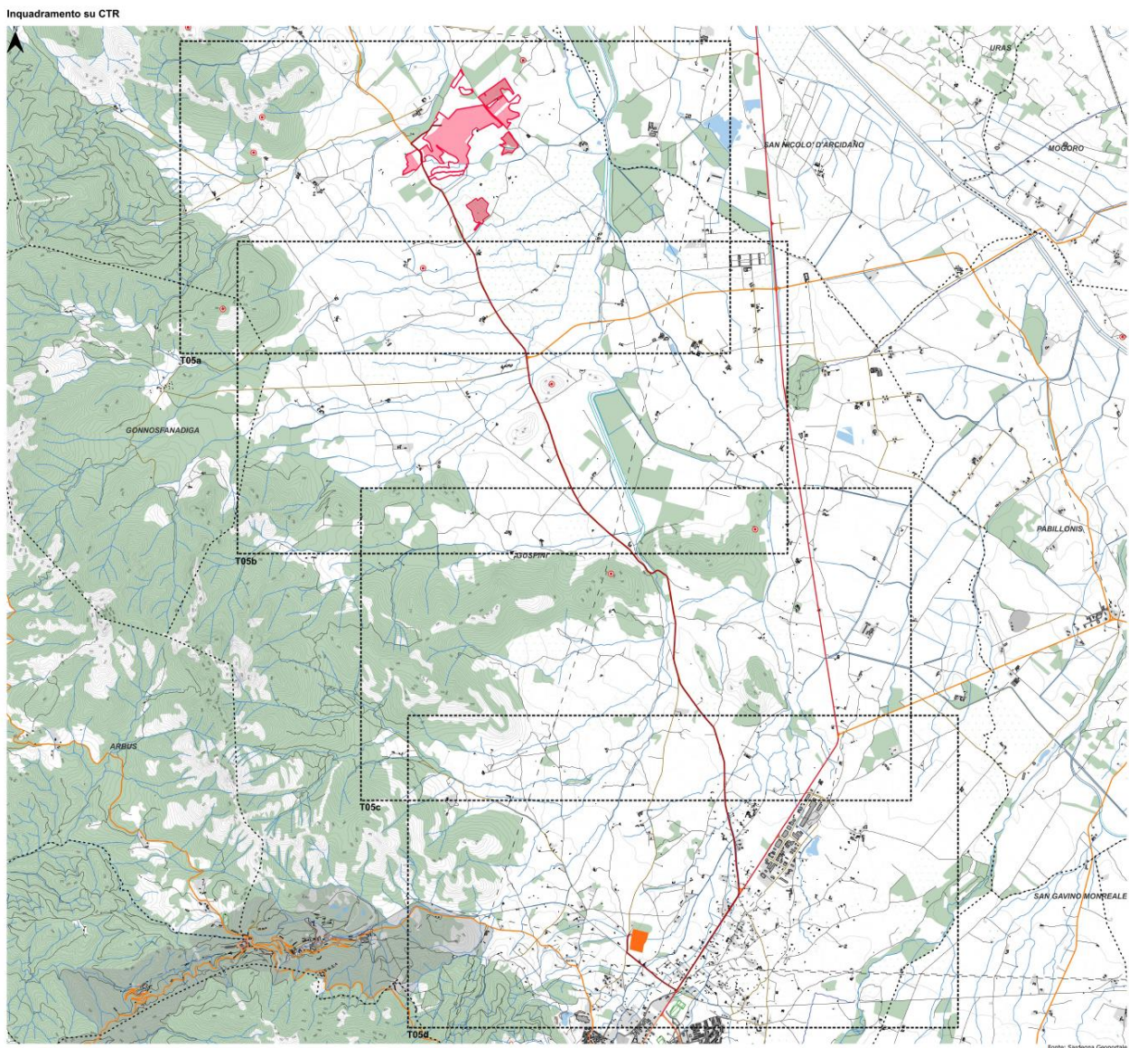
Figura 3 - Elettrodotto e sottostazione
