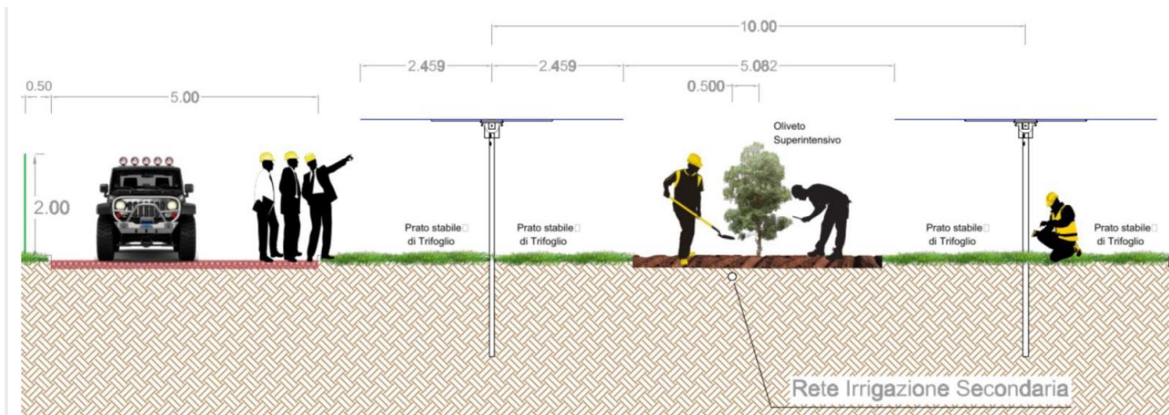
Sezione dell'impianto con l'indicazione della disposizione delle colture agrarie e della recinzione perimetrale. Area dei tracker.
