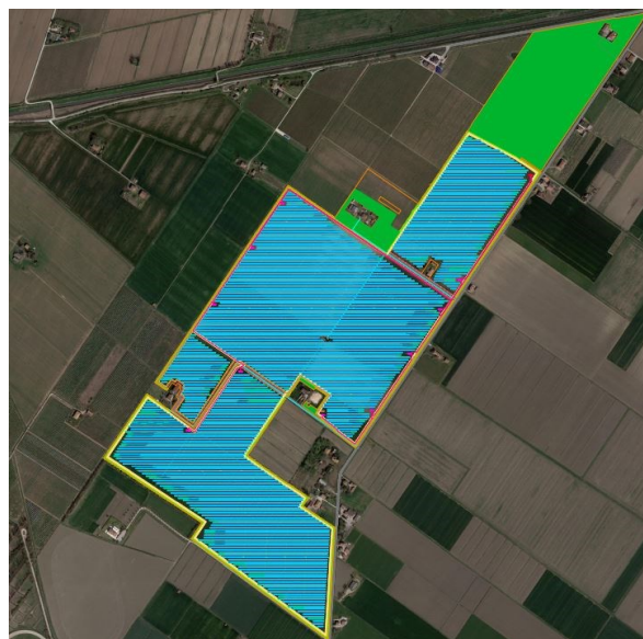
Figura 2 - Layout impianto su Ortofoto
