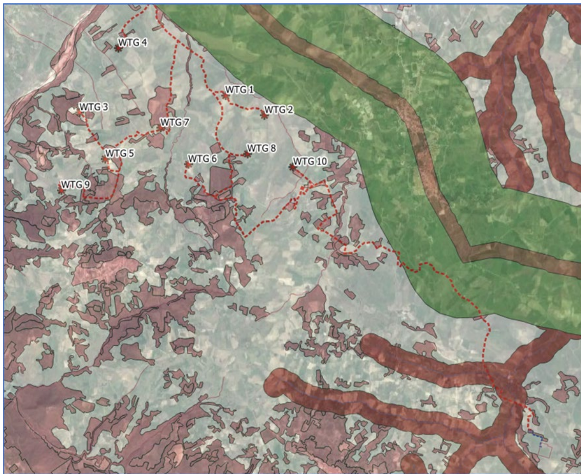
Figura 4 - layout impianto a n.10 aerogeneratori
