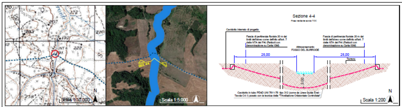
Figura 10 - Stralcio studio degli attraversamenti – tipologico
