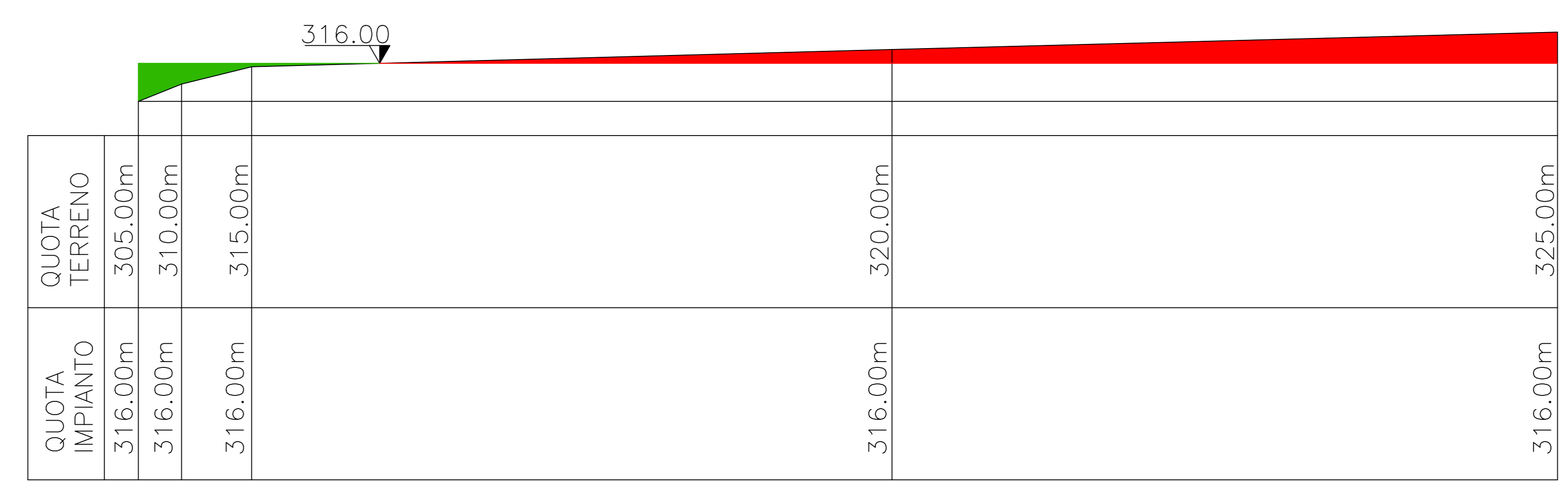
SEZIONE B-B
