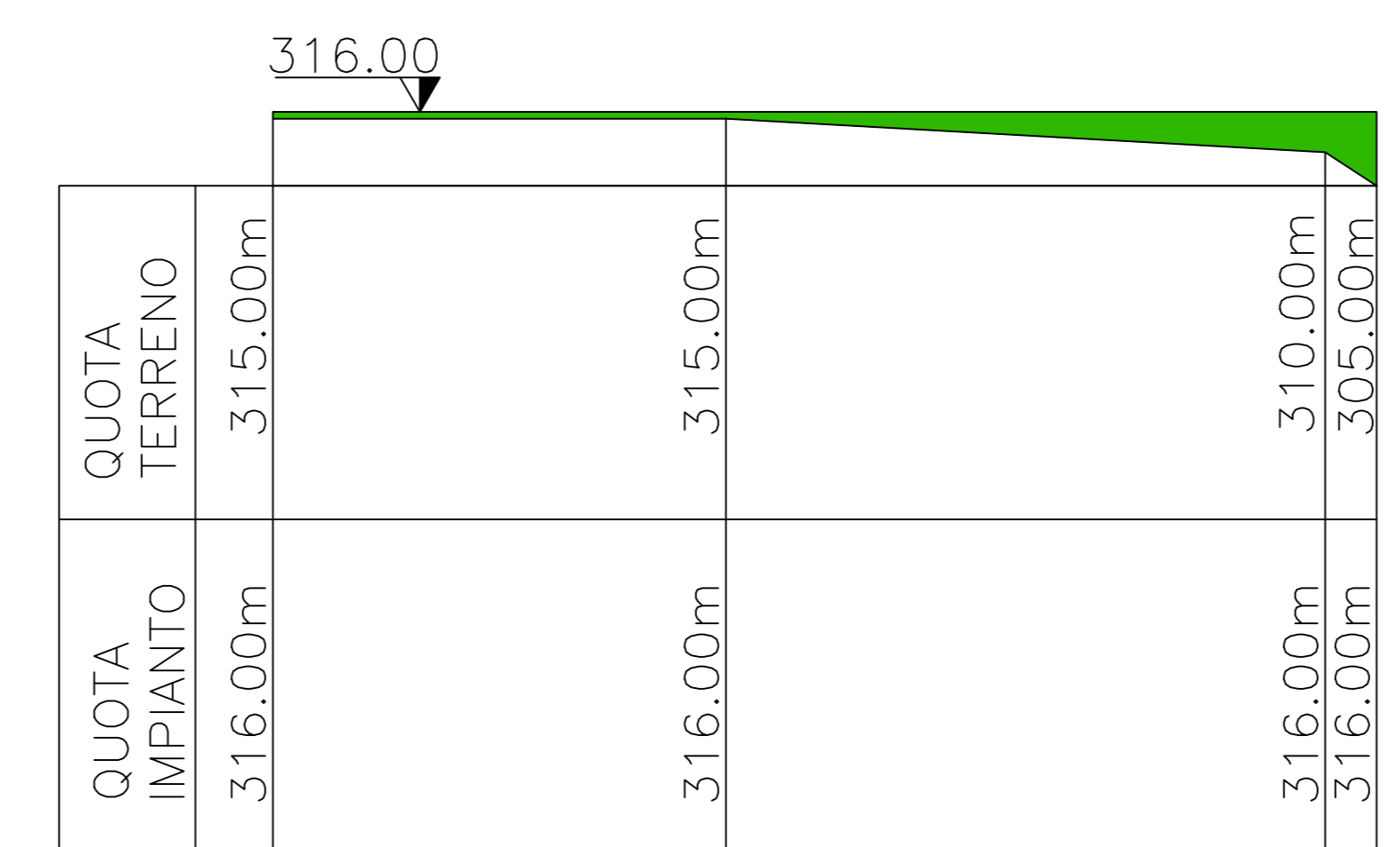
SEZIONE D-D
