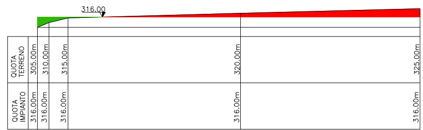
SEZIONE B-B
