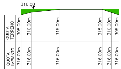
SEZIONE C-C
