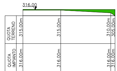
SEZIONE D-D
