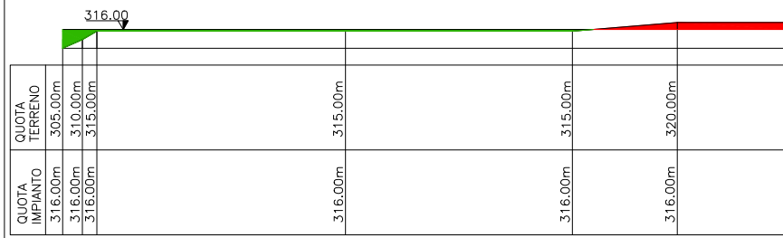
SEZIONE A-A
