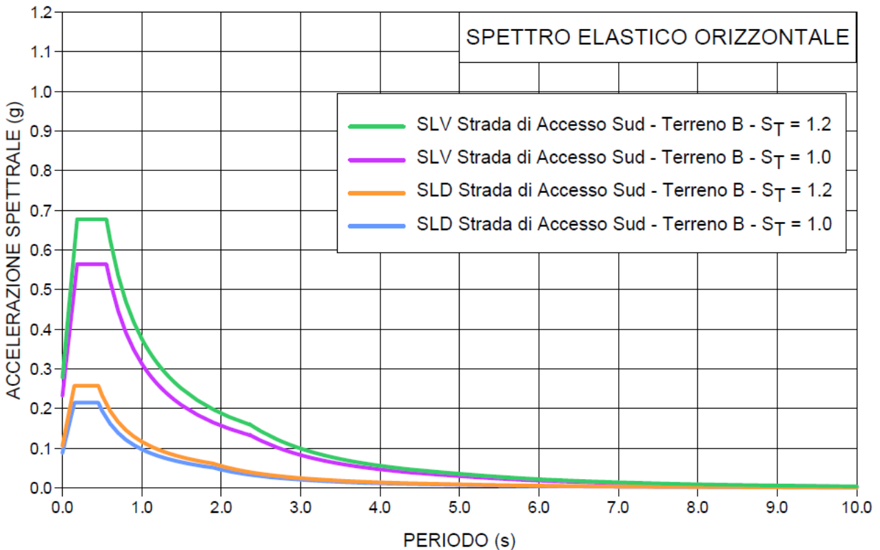
Figura 6-2 - Spettri Elastici Orizzontali – Esempio di Classe III
