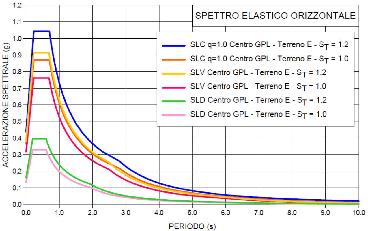
Figura 6-3 - Spettri Elastici Orizzontali – Esempio di Classe IV
