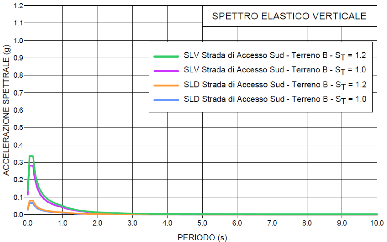
Figura 6-6 - Spettri Elastici Verticali – Esempio di Classe III
