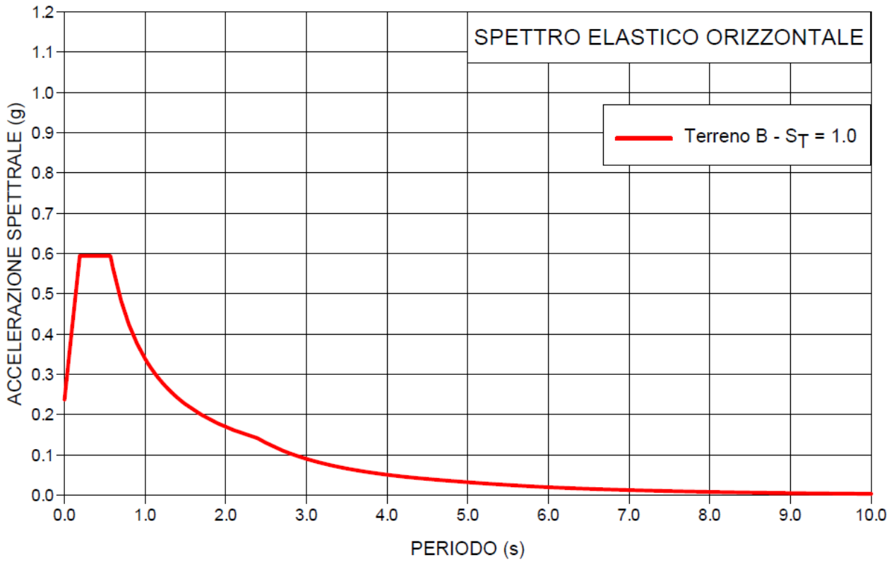
Figura B-2 - Spettri Elastici Orizzontali per Moto del Suolo Orizzontale con Smorzamento del 5% Struttura Principale nel Centro Oli - SLV
