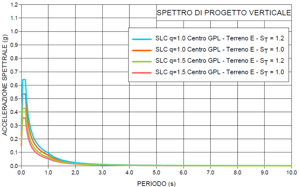
Figura 6-8 - Spettri Verticali di Progetto per lo Stato Limite SLC – Esempio di Classe IV
