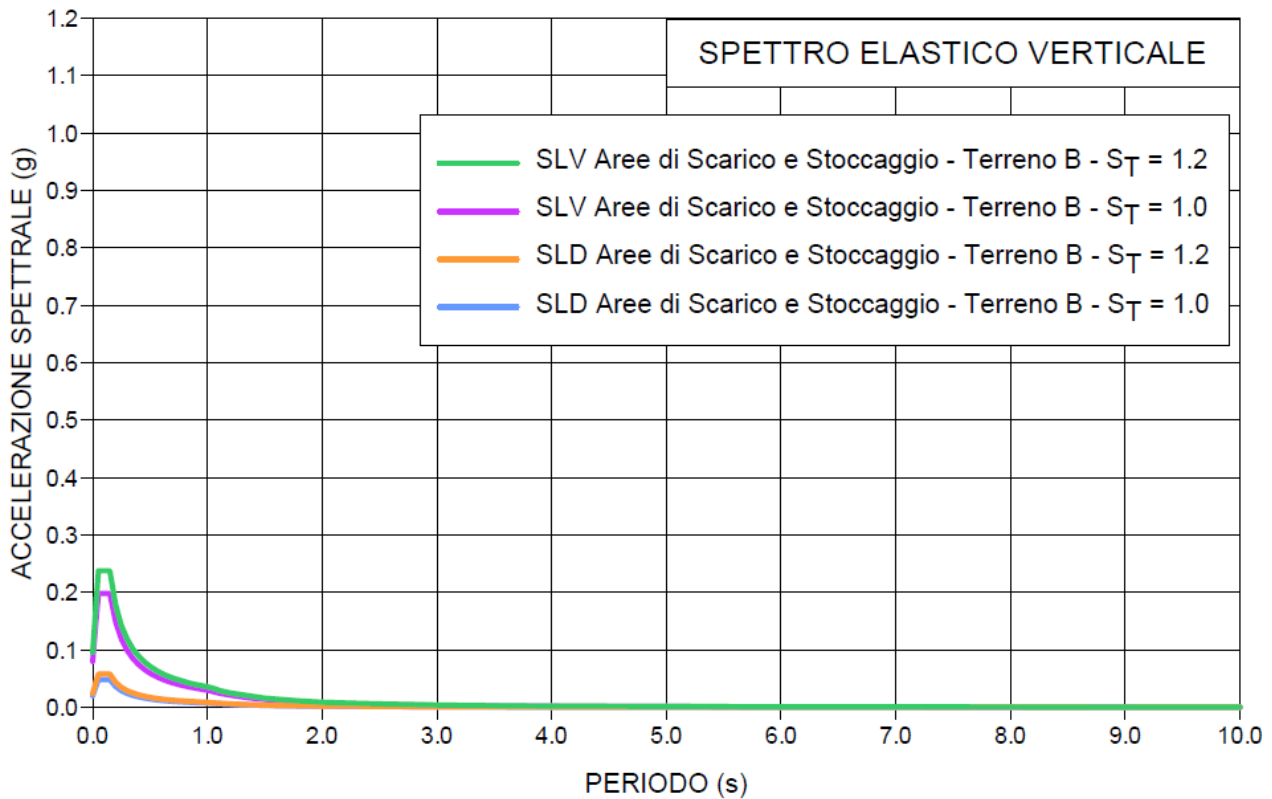
Figura 6-5 - Spettri Elastici Verticali – Esempio di Classe II
