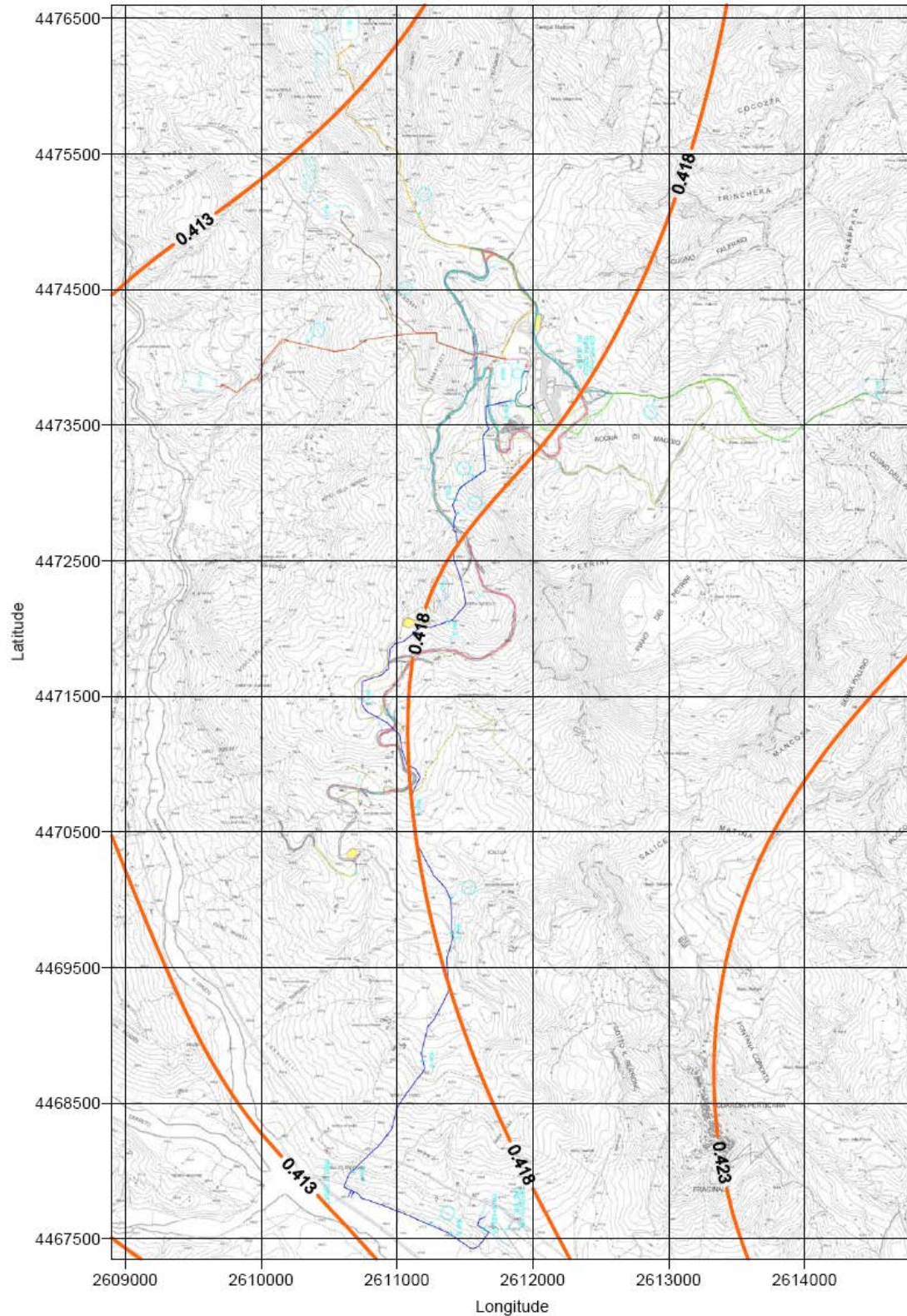
Figure A-3 - Variability of T_c – 475 years (NTC 08) Figura A-3 – Variabilità di T_c – 475 anni (NTC 08)
