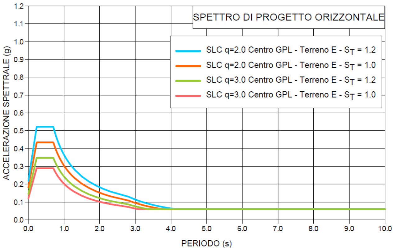
Figura 6-4 - Spettri Orizzontali di Progetto per lo Stato Limite SLC – Esempio di Classe IV
