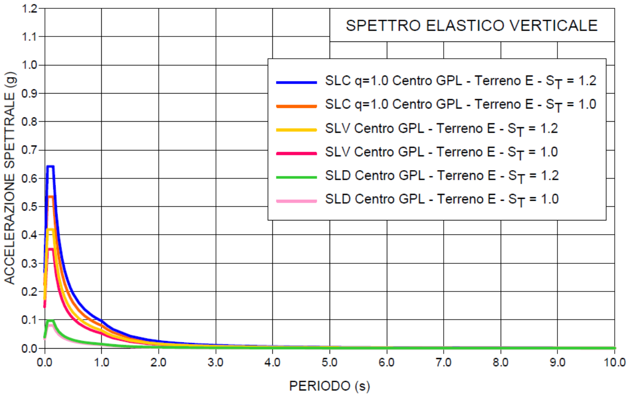
Figura 6-7 - Spettri Elastici Verticali – Esempio di Classe IV
