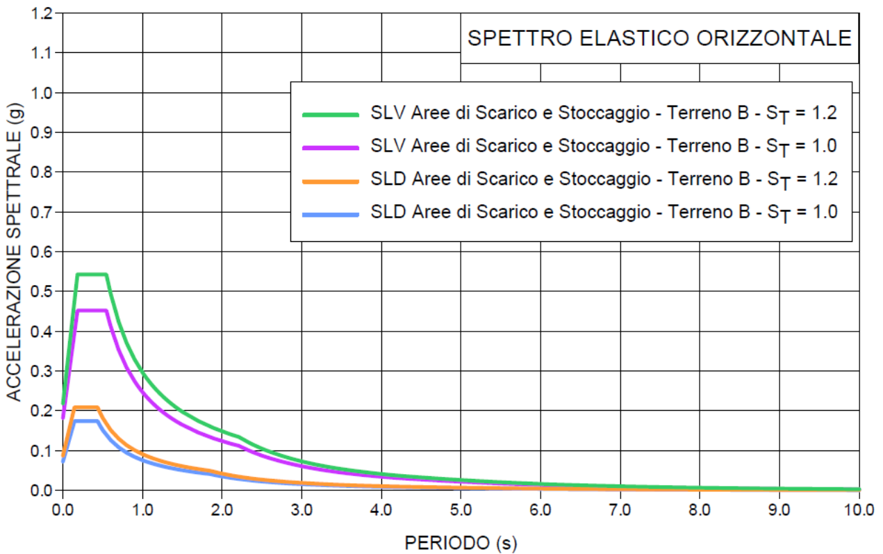
Figura 6-1 - Spettri Elastici Orizzontali – Esempio di Classe II
