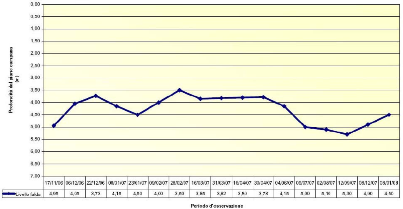
Profondità della falda dal piano campagna (Piezometro D5PZS2)
