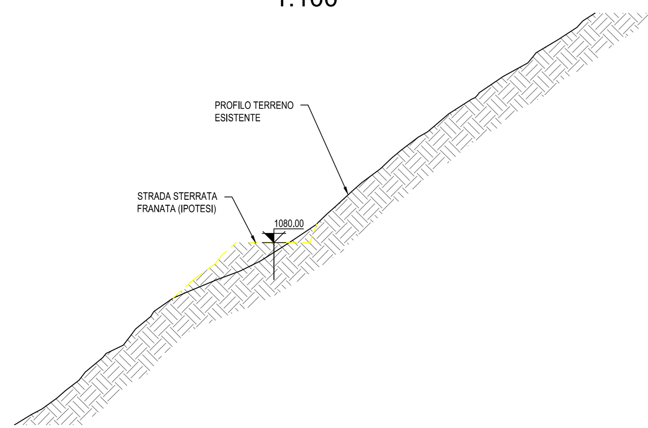
SEZIONE B-B 1:100
