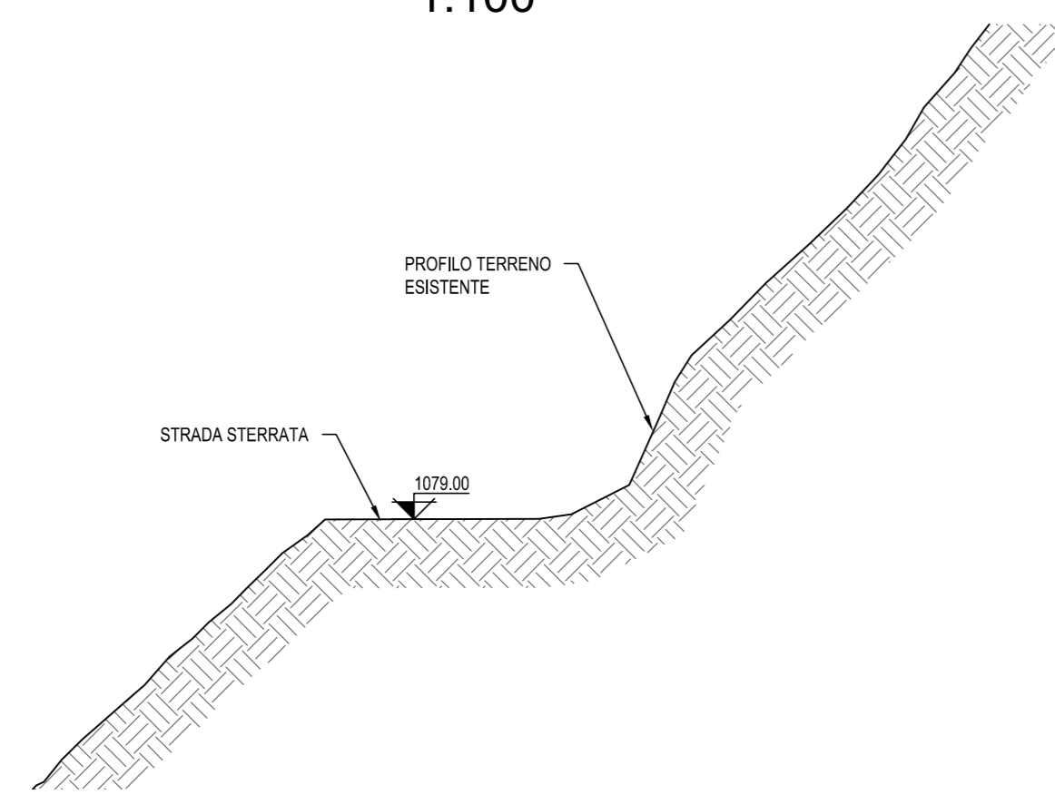
SEZIONE D-D 1:100
