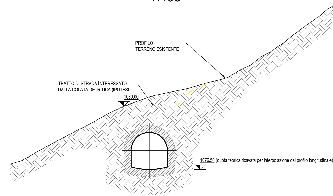
SEZIONE A-A 1:100
