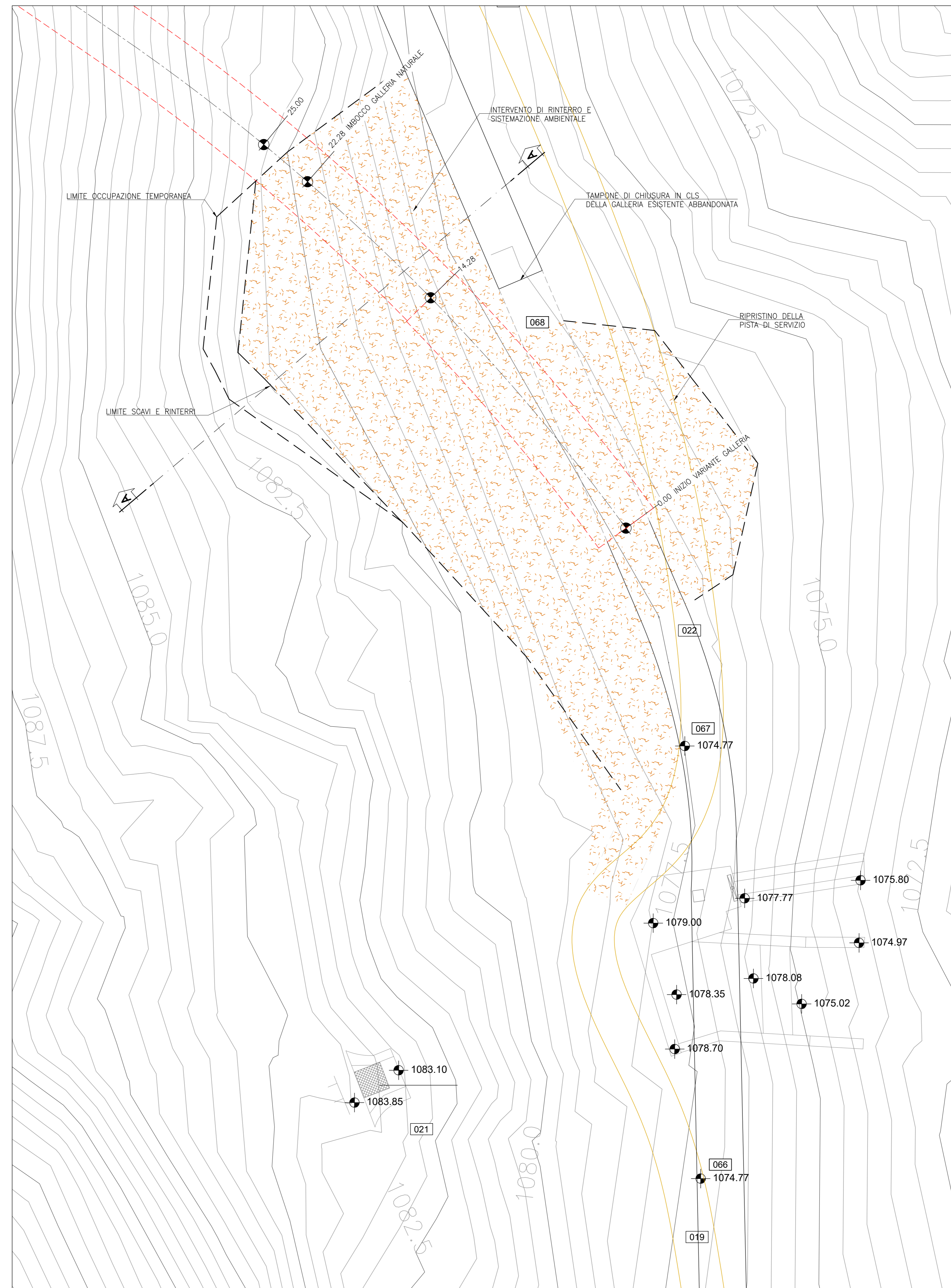
PLANIMETRIA ZONA DI IMBOCCO A LAVORI ULTIMATI - Scala 1:100
