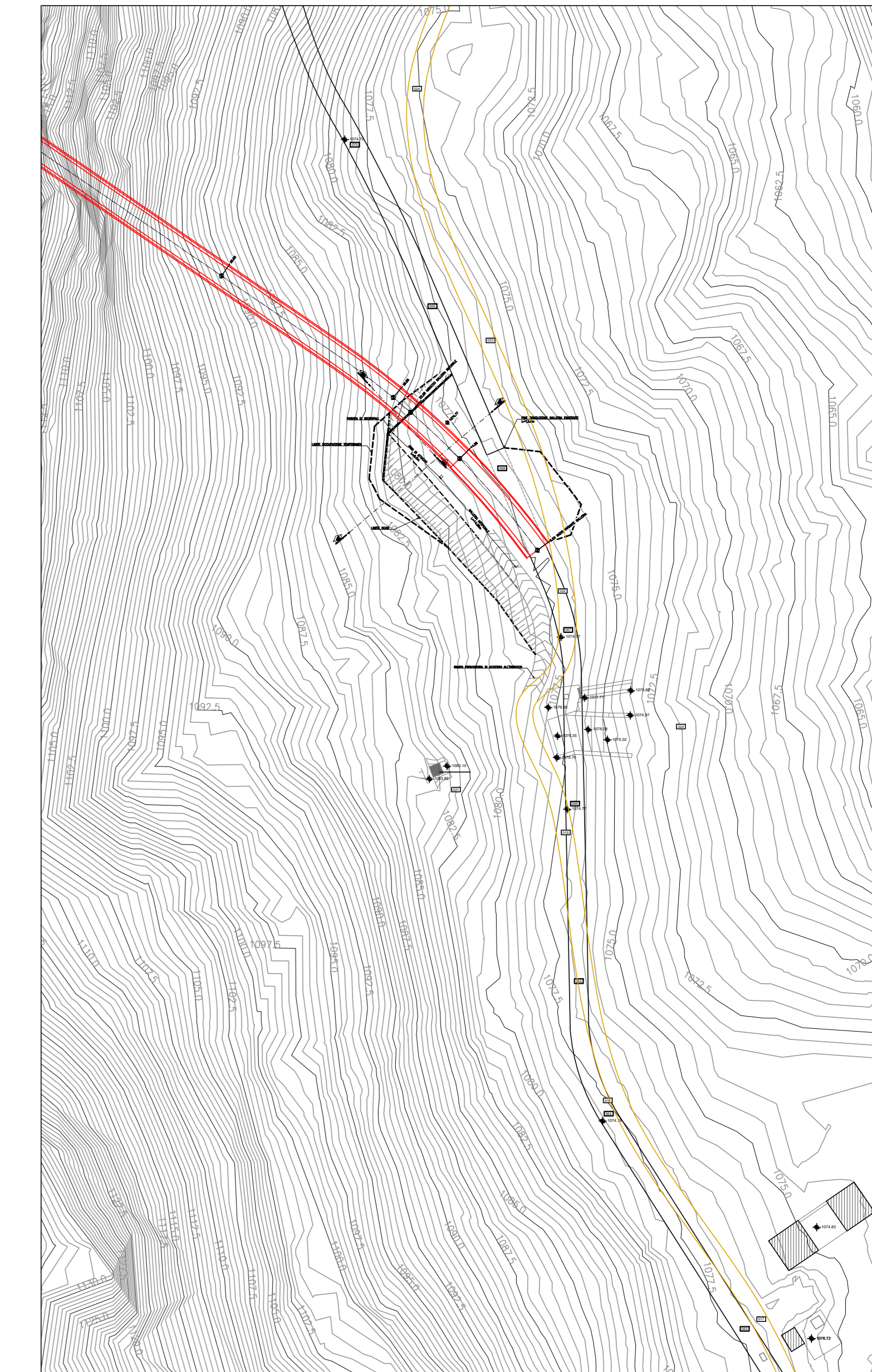
INQUADRAMENTO IMBOCCO DI MONTE - Scala 1:500
