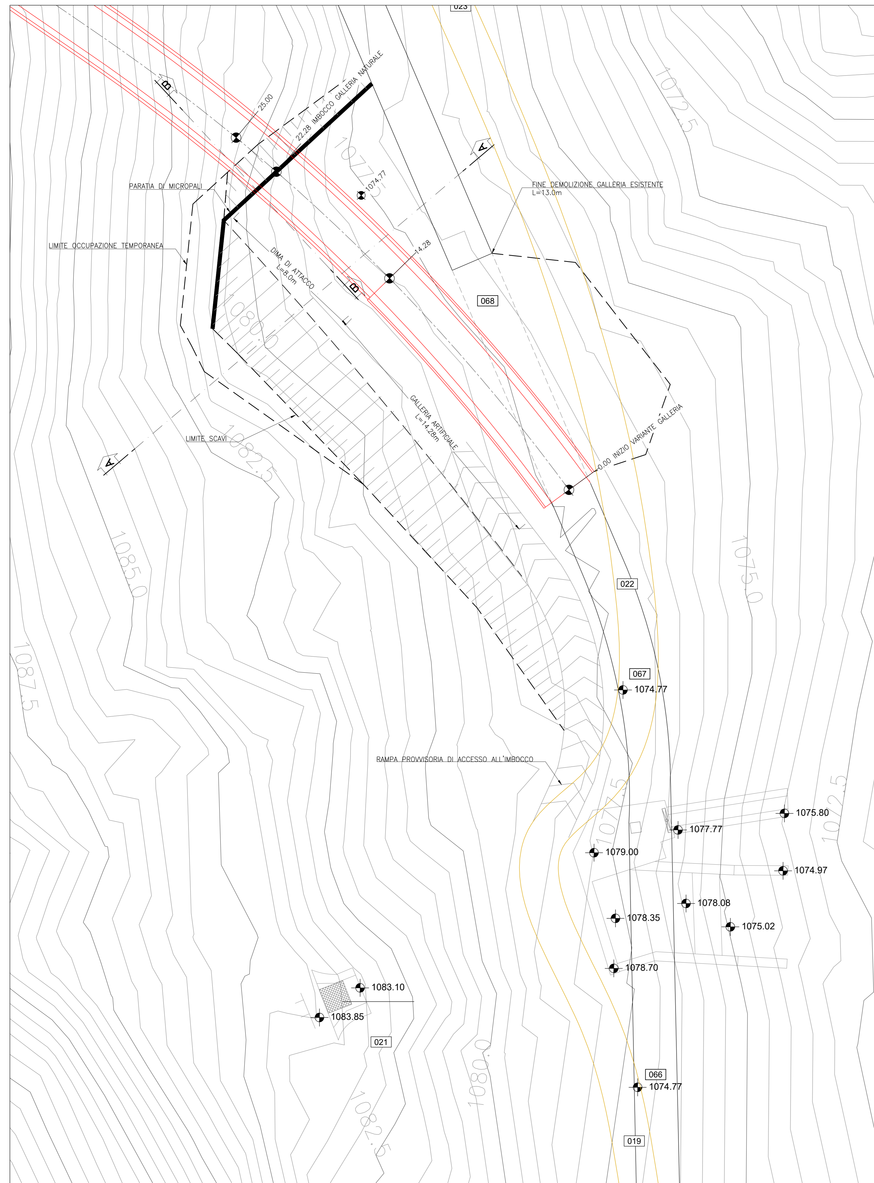
PLANIMETRIA ZONA DI IMBOCCO IN FASE DI LAVORO - Scala 1:100
