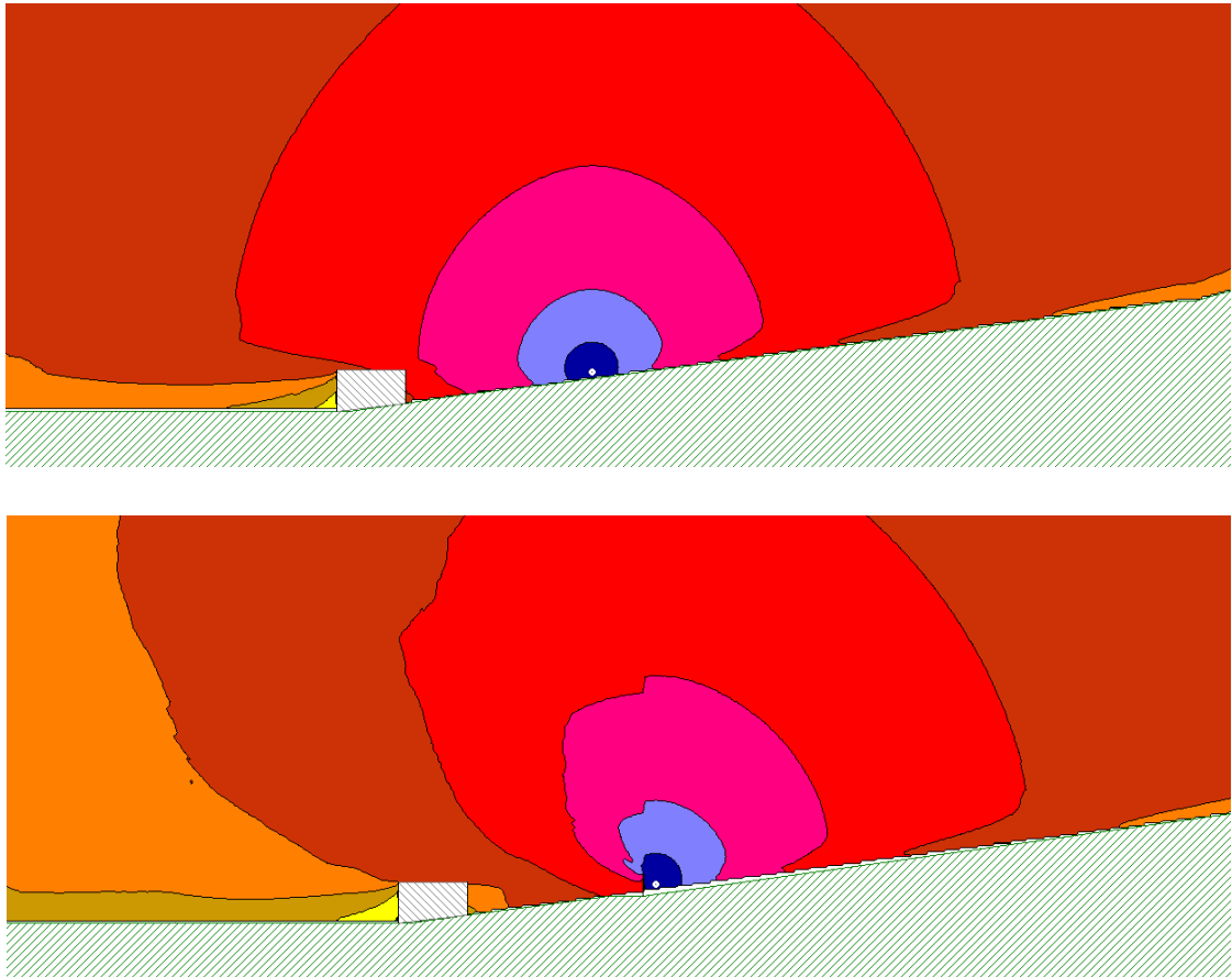
Figura 6 Rumore generato dalla lavorazione di posa cavidotto prima e dopo le opere di mitigazione riceettore RC02
