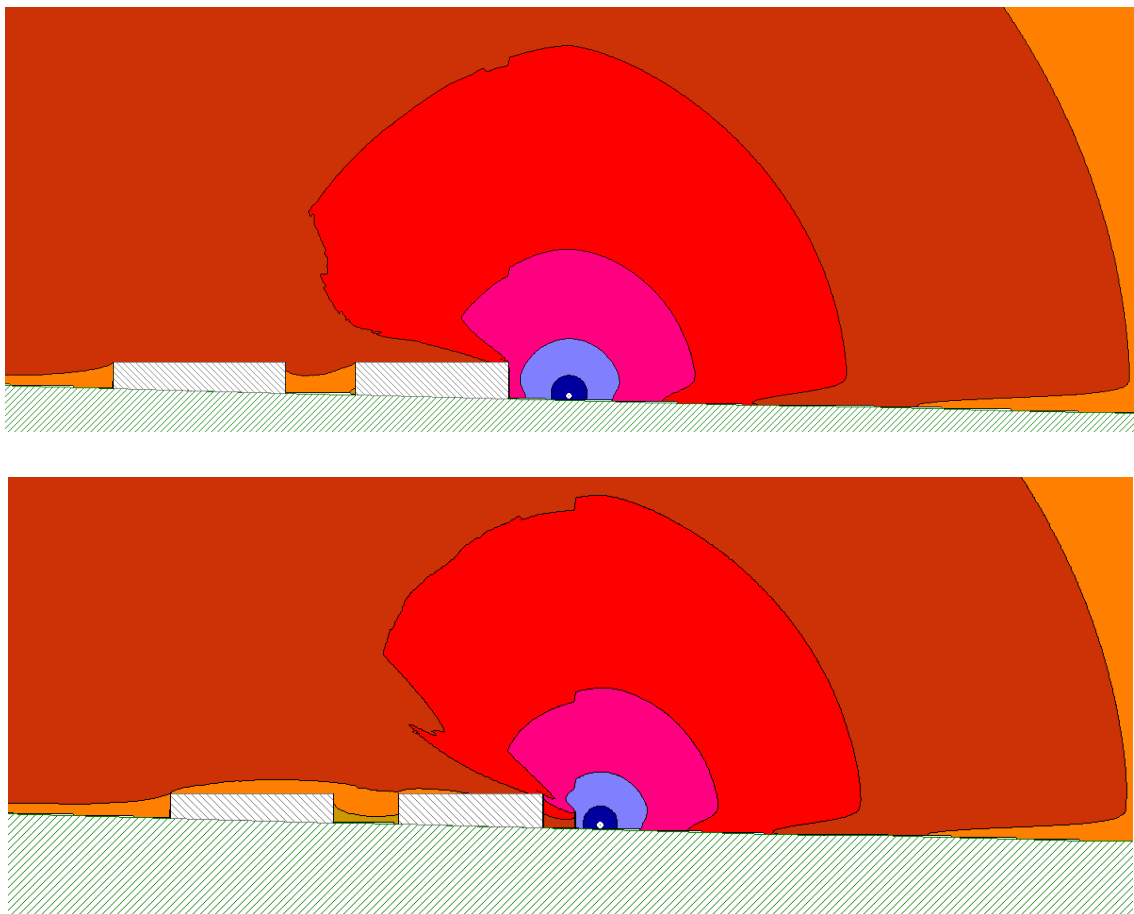
Figura 5 Rumore generato dalla lavorazione di posa cavidotto prima e dopo le opere di mitigazione ricettore RC01
