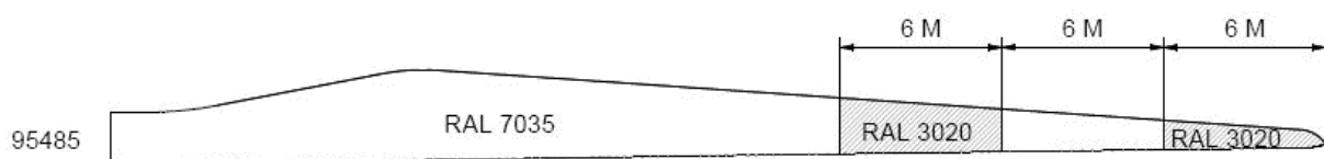
Figura 6.1 – Schema indicativo colorazione pale (la larghezza effettiva delle bande colorate sarà apposta in accordo con quanto specificato in Tabella 6.1)
