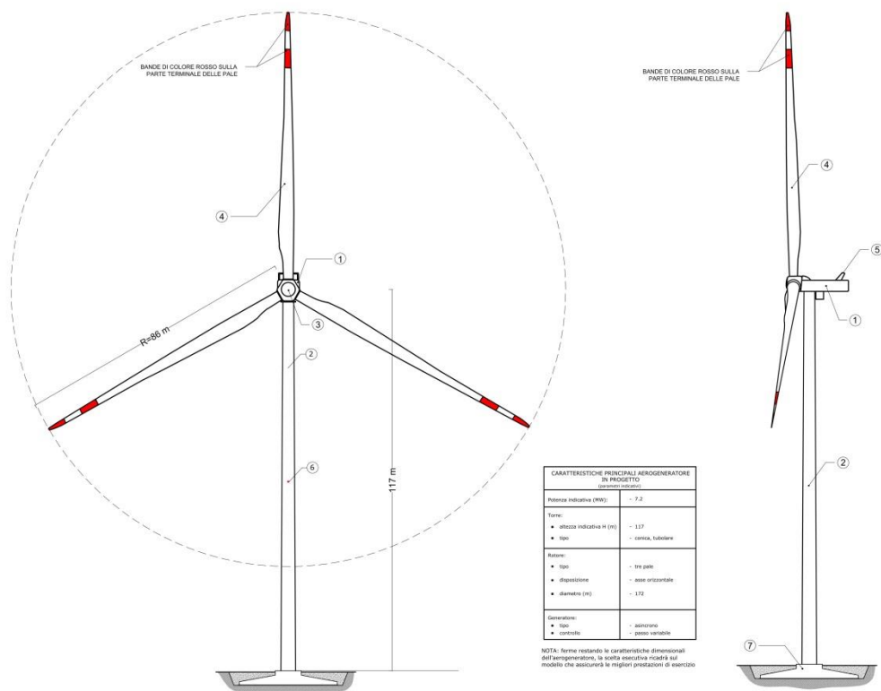
Figura 4.1 – Aerogeneratore di progetto con altezza al mozzo 117 m e diametro rotore di 172 m
