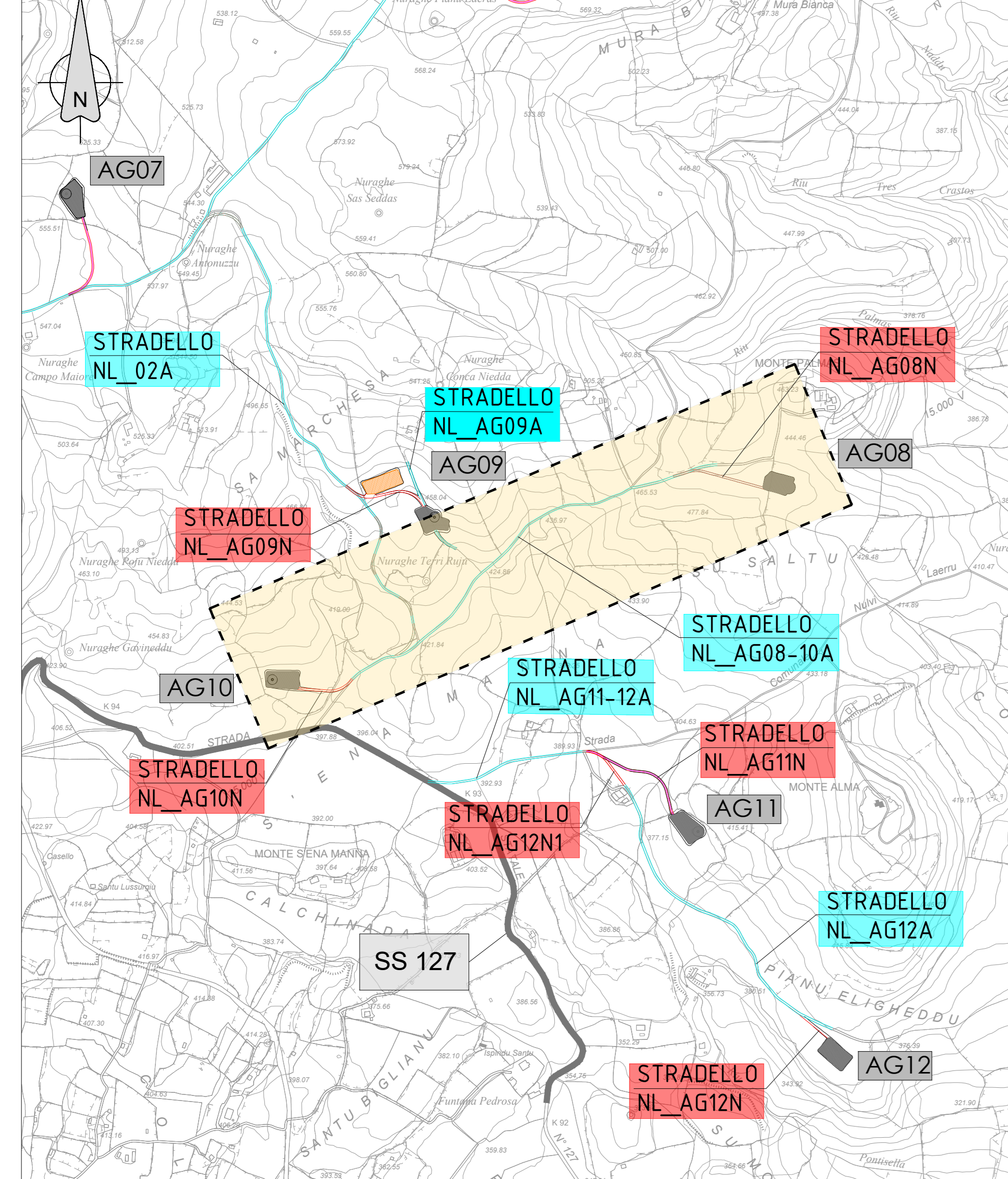
QUADRIAMO GENERALE INTERVENTI REALIZZAZIONE ADEGUAMENTI VIABILITA' ESISTENTE - SCALA 1:10.000
