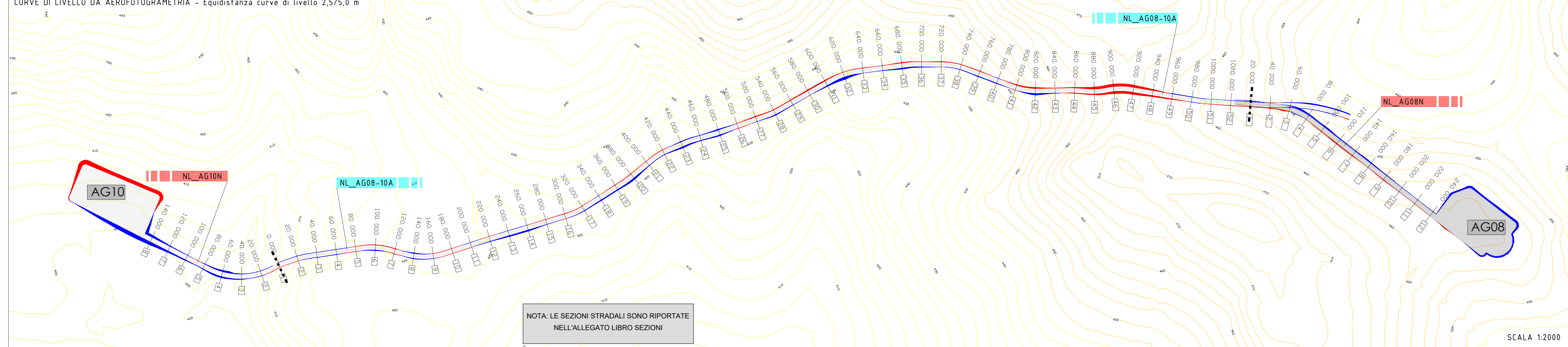
PLANIMETRIA ADEGUAMENTI VIABILITA' ESISTENTE (NL_AG08-10A) E NUOVA VIABILITA' (NL_AG08N e NL_AG10N) SU CURVE DI LIVELLO DA RILIEVO LIDAR
