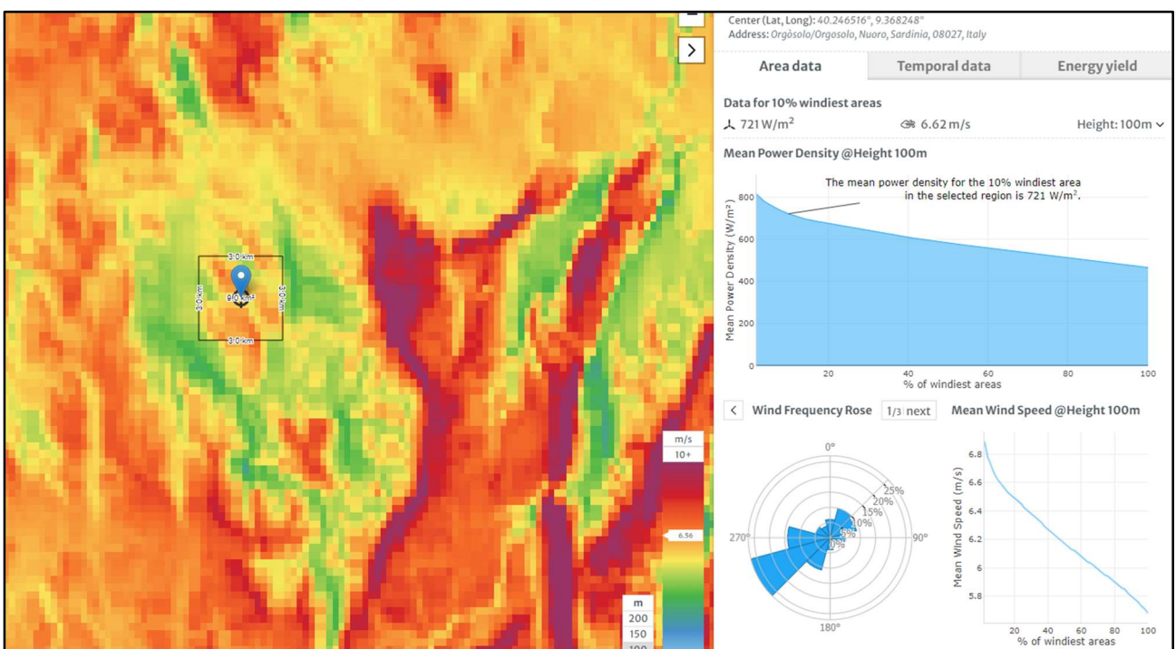
Figura 8.1.1c: Mappa di ventosità dell'area di progetto e rosa dei venti (Fonte globalwindatlas.info/en )
