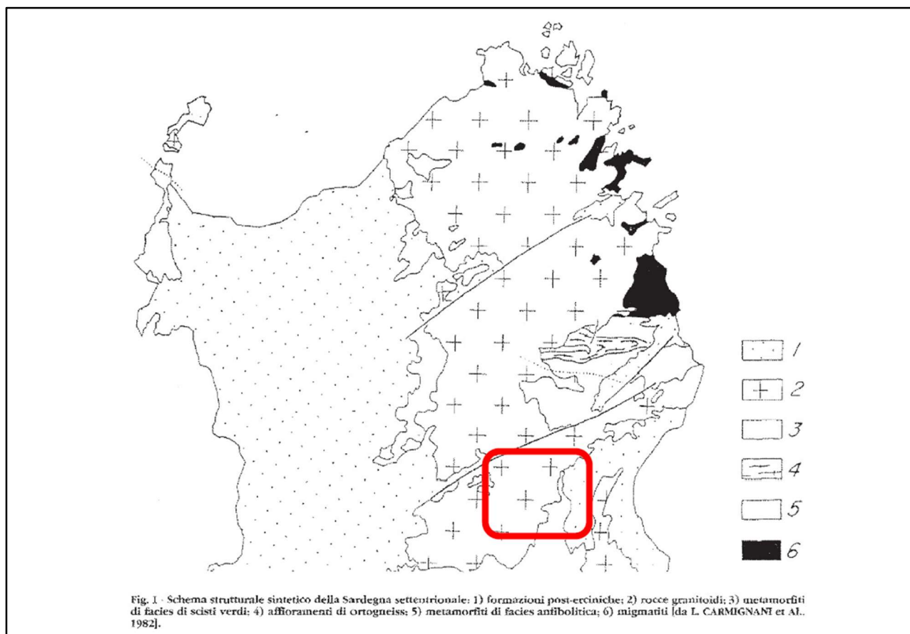
Figura 8.2.1: Schema strutturale sintetico della Sardegna Settentrionale
