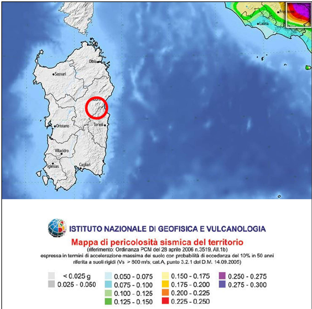
Figura 8.3.1: Classificazione sismica dei comuni interessati dal progetto (Fonte INGV)
