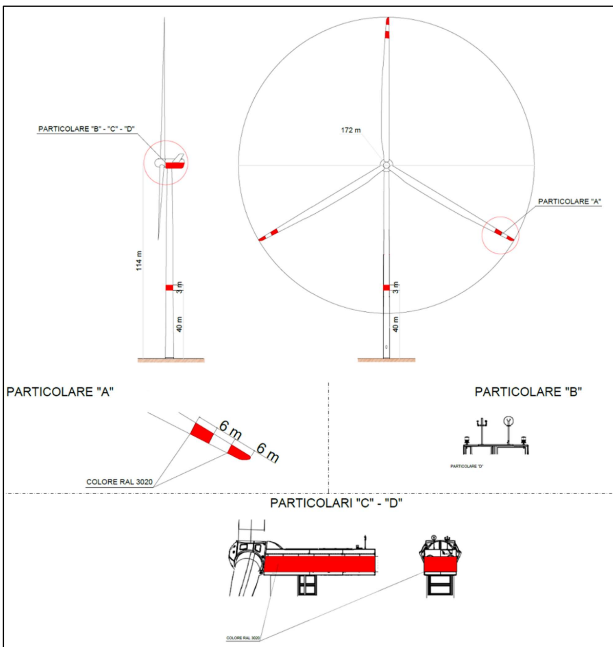
Figura 6.1.1: Profilo aerogeneratore V172 – 7,2 MWp – HH = 114 m – D = 172 m
