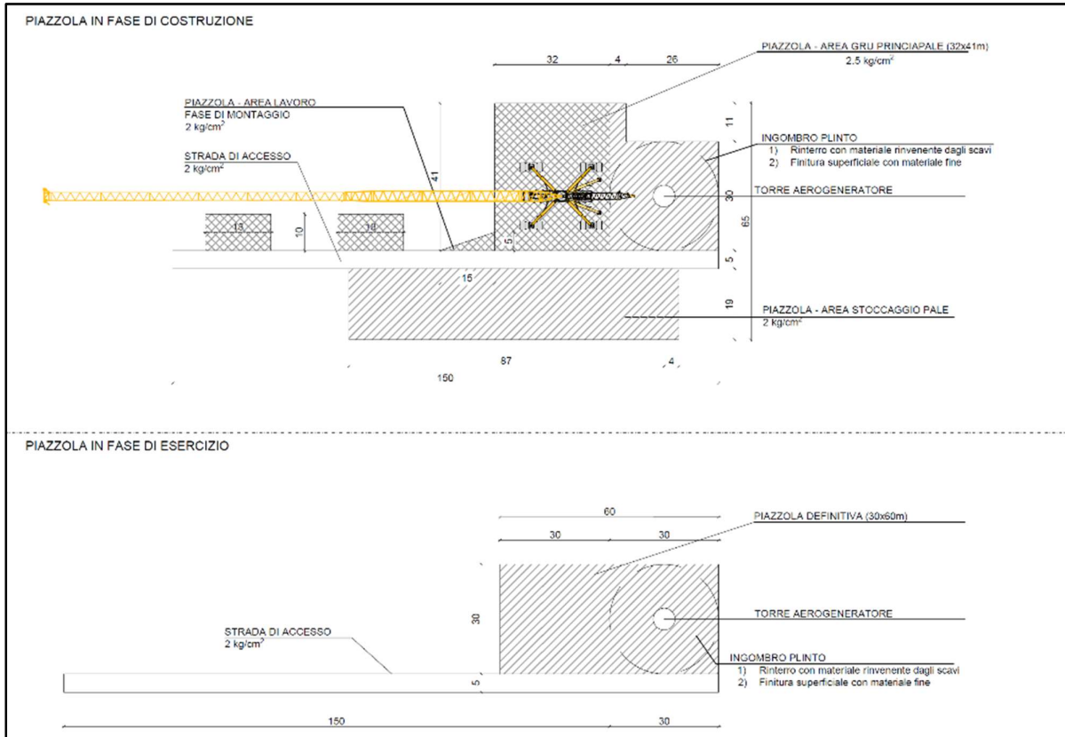
Figura 6.2.2: Planimetria piazzola tipo per la fase di installazione e fase di esercizio e manutenzione
