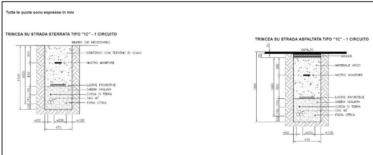
Figura 6.3.4.2: Sezioni tipiche delle trincee cavidotto per una terna di cavi in parallelo su strada sterrata e asfaltata
