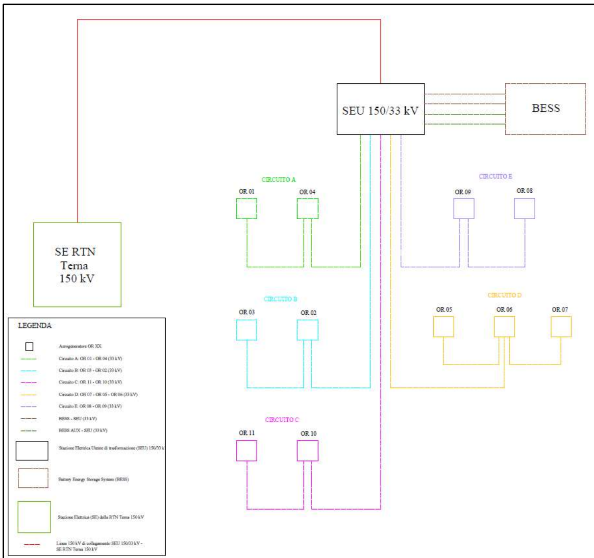
Figura 6.3.4.1: Schema a blocchi del Parco Eolico Orgosolo - Oliena
