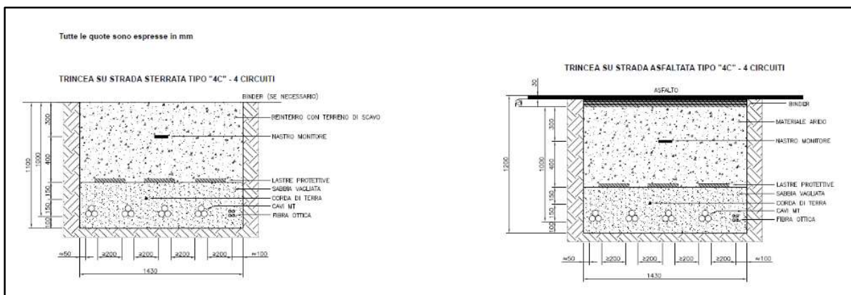
Figura 6.3.4.5: Sezioni tipiche delle trincee cavidotto per quattro terne di cavi in parallelo su strada sterrata e asfaltata
