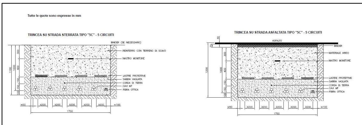
Figura 6.3.4.6: Sezioni tipiche delle trincee cavidotto per cinque terne di cavi in parallelo su strada sterrata e asfaltata
