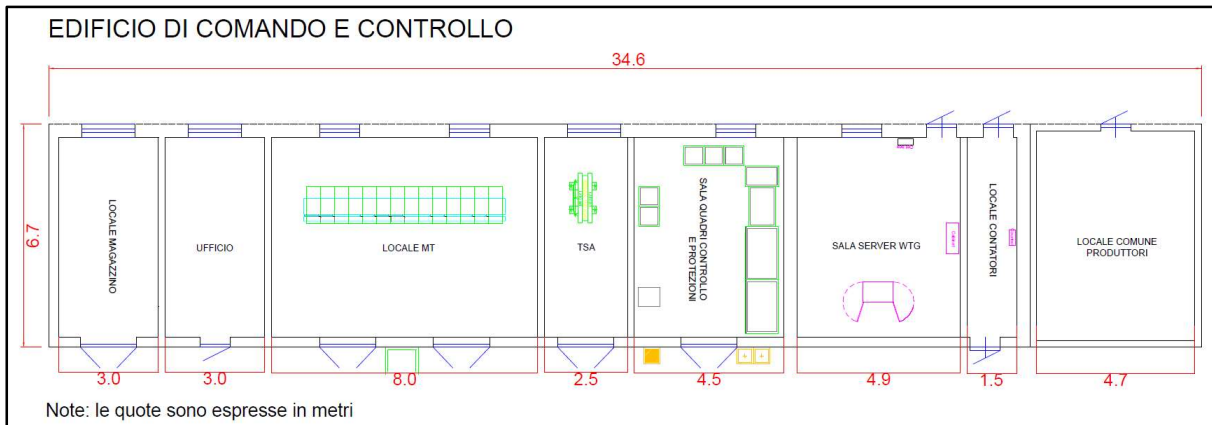
Figura 6.3.3.2: Pianta edificio di comando e controllo della SEU 150/33 kV
