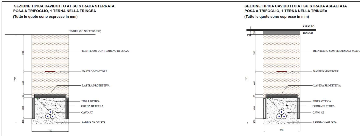
Figura 6.3.5.1: Sezione tipica del cavidotto AT
