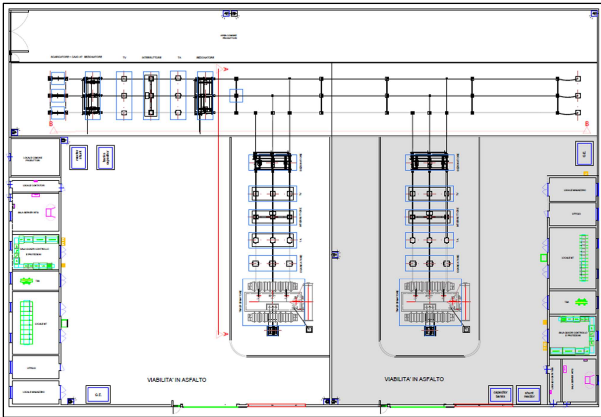
Figura 6.3.3.1: Planimetria elettromeccanica della Stazione Elettrica Utente 150/33 kV
