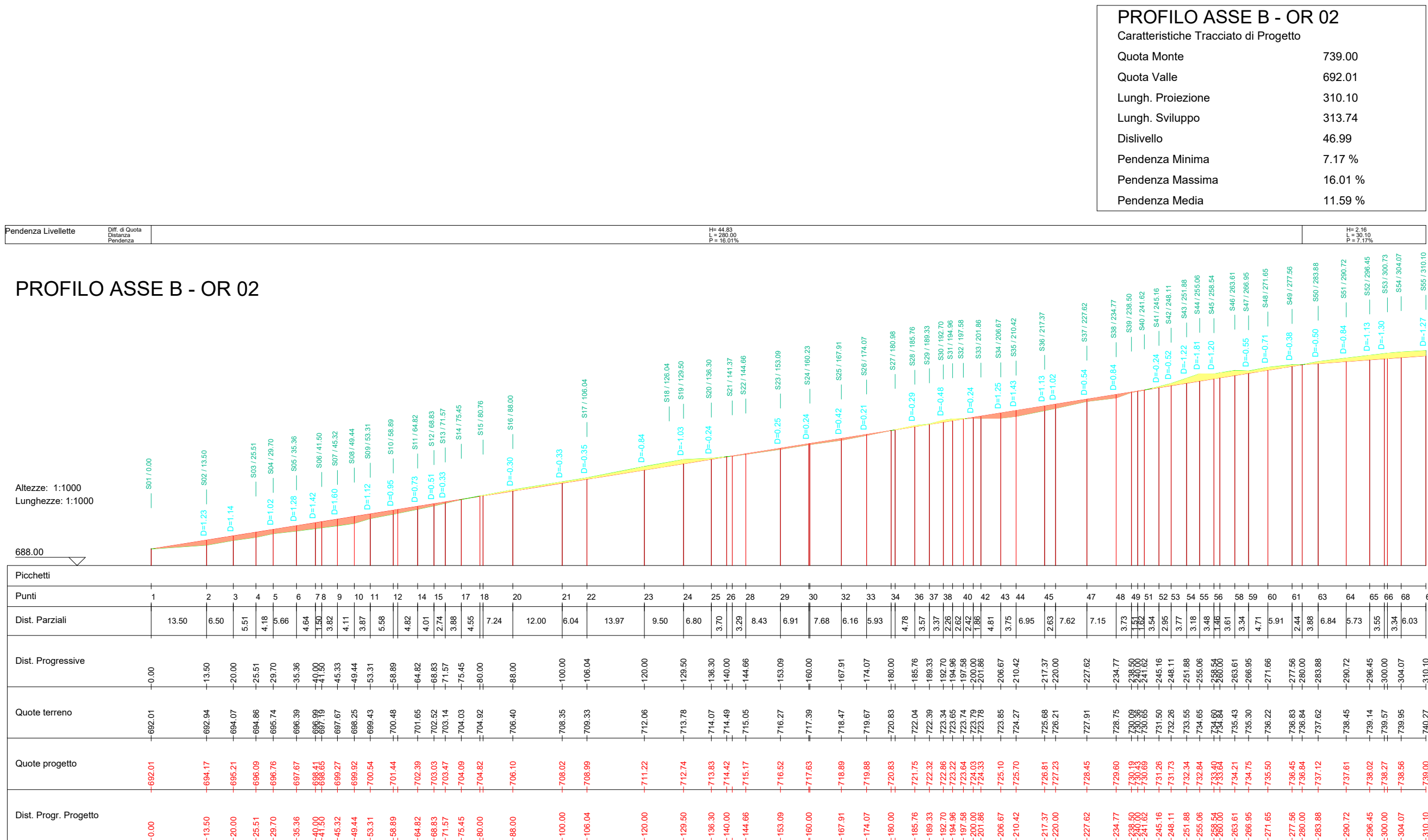
PLANIMETRIA PIAZZOLA OR02 E PROFILO B - OR02 SU CURVE DI LIVELLO_SCALA 1:1.000
