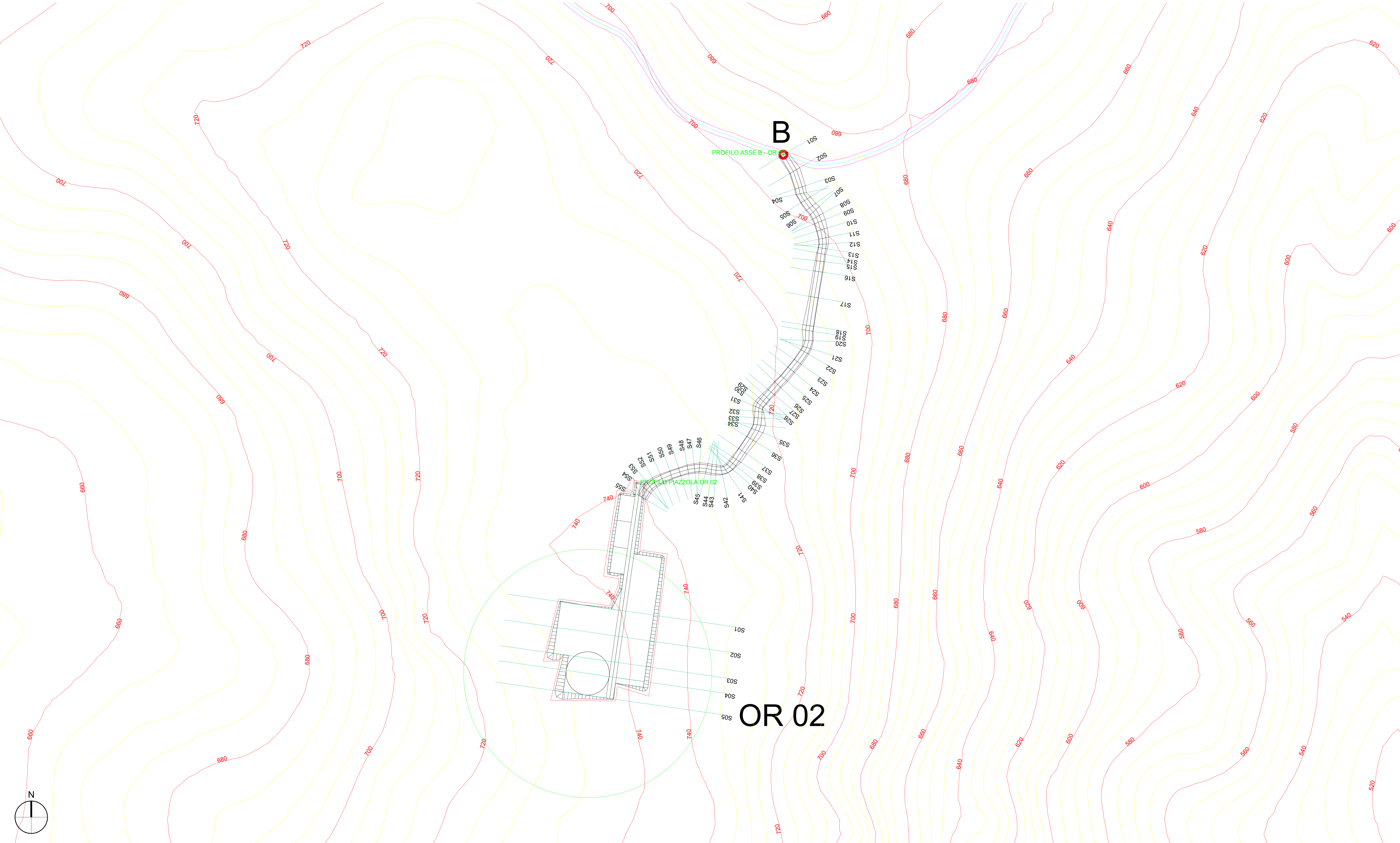
PLANIMETRIA PIAZZOLA OR02 E PROFILO B - OR02 SU CURVE DI LIVELLO_SCALA 1:1.000
