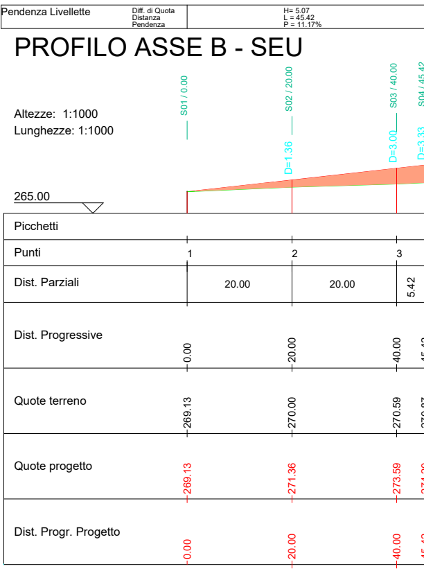
PLANIMETRIA AREA SEU - BESS E PROFILO AREA SEU - BESS CURVE DI LIVELLO_SCALE 1:1.000
