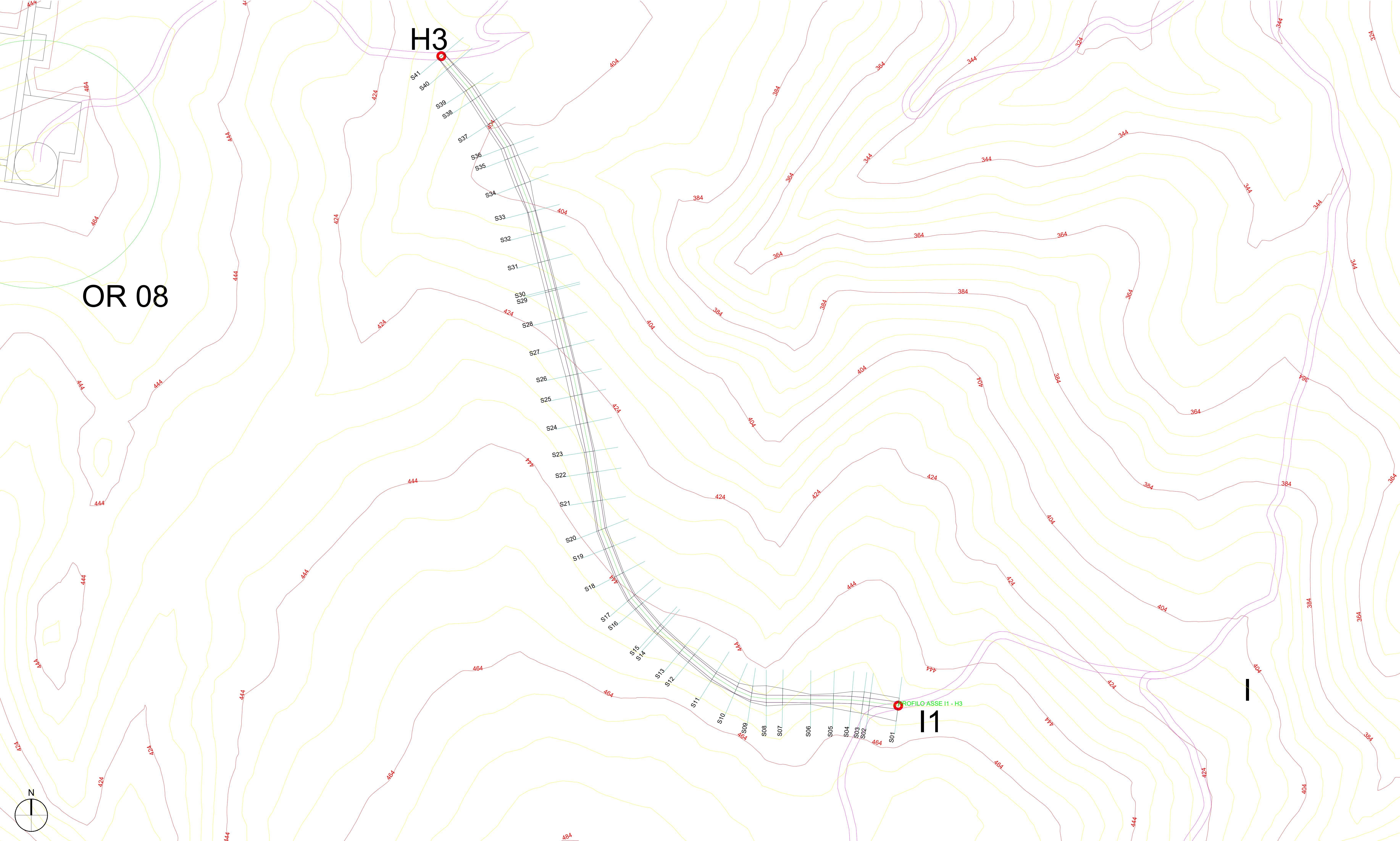
PLANIMETRIA ASSE I1 - H3 E PROFILO I1 - H3 SU CURVE DI LIVELLO_SCALA 1:1.000
