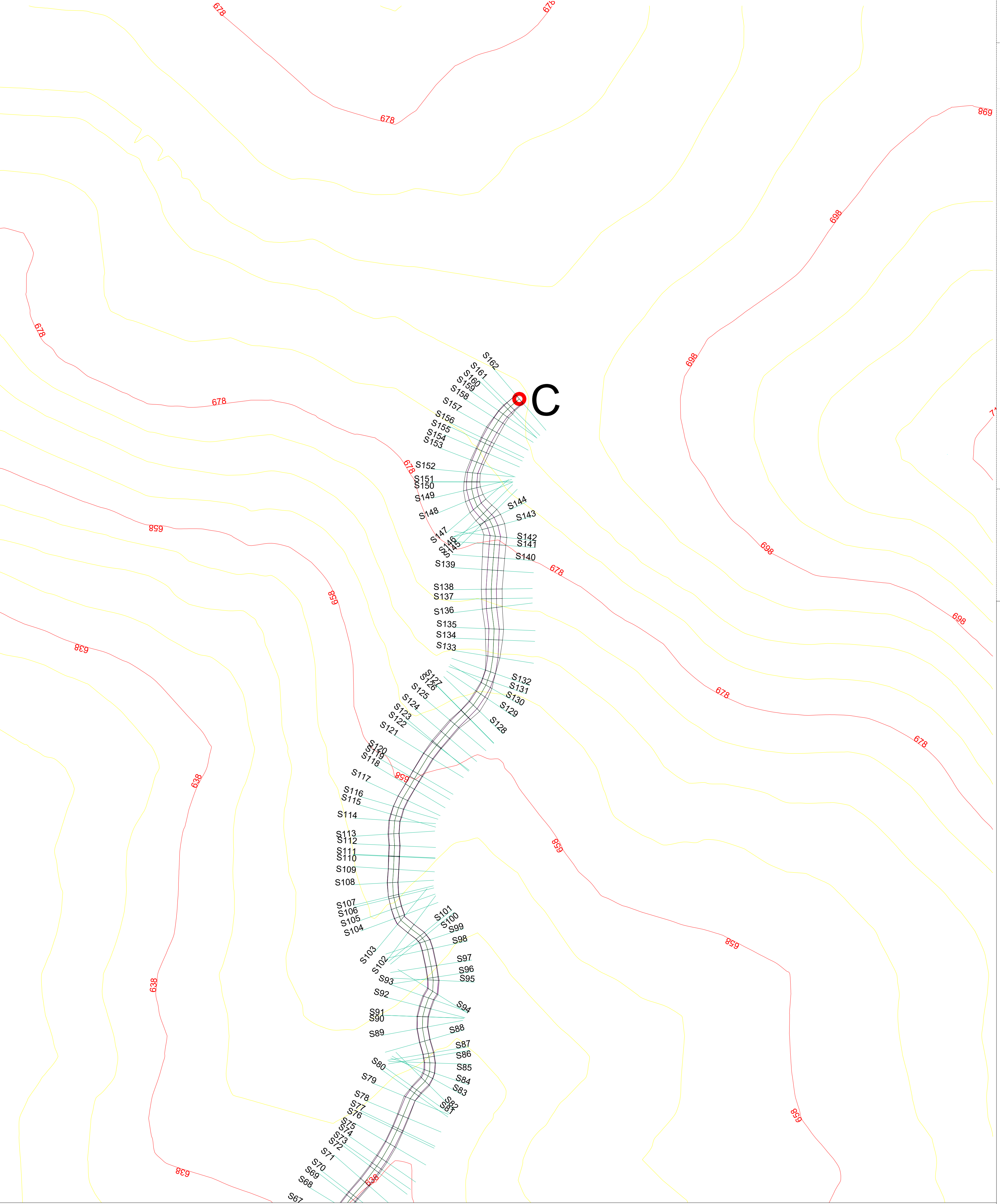
PLANIMETRIA C1 - C (SEZIONI DA 69 - 162) E PROFILO C1 - C SU CURVE DI LIVELLO_SCALE 1:1.000
