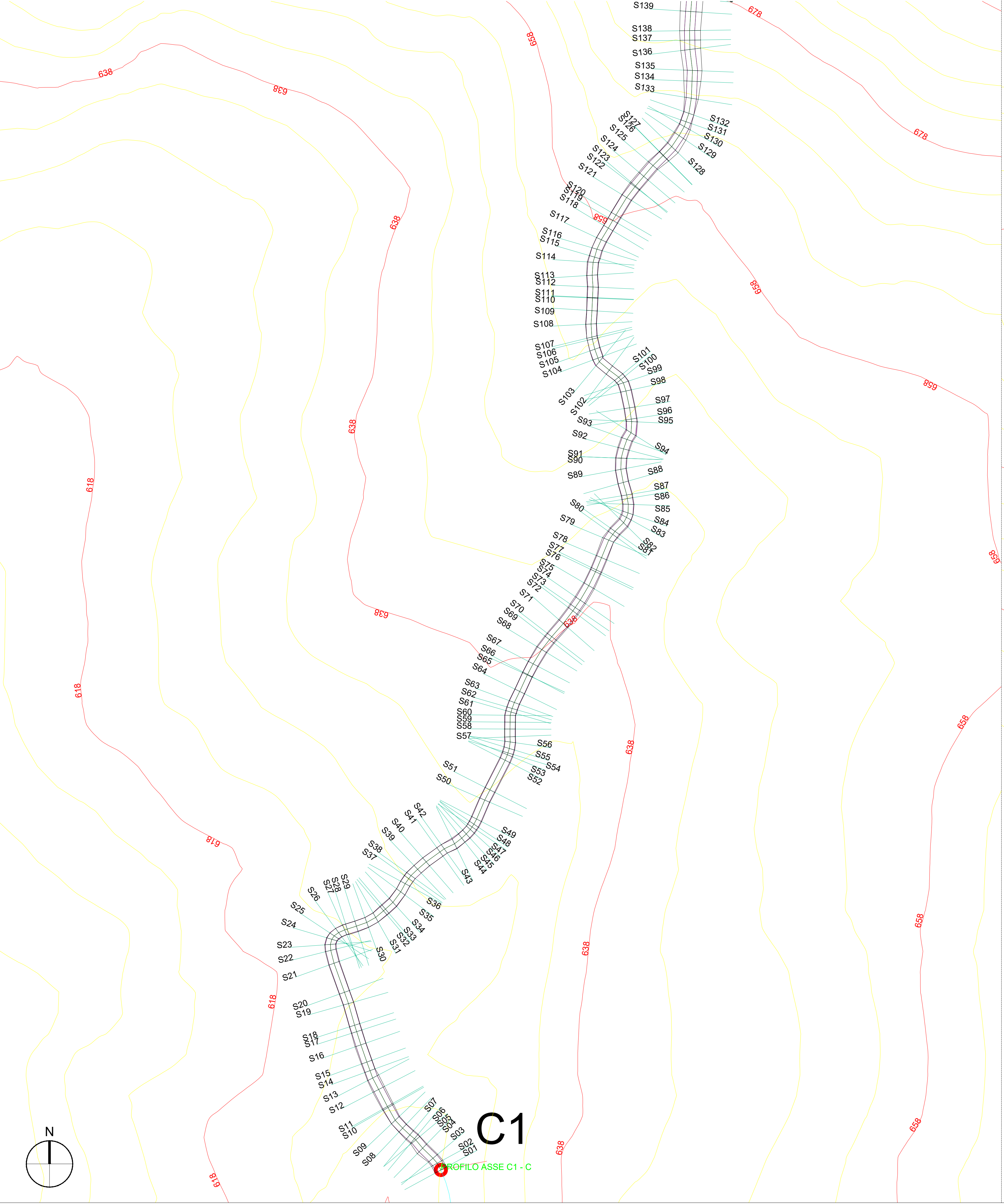
PLANIMETRIA C1 - C (SEZIONI DA 1 - 139) E PROFILO C1 - C SU CURVE DI LIVELLO_SCALE 1:1.000
