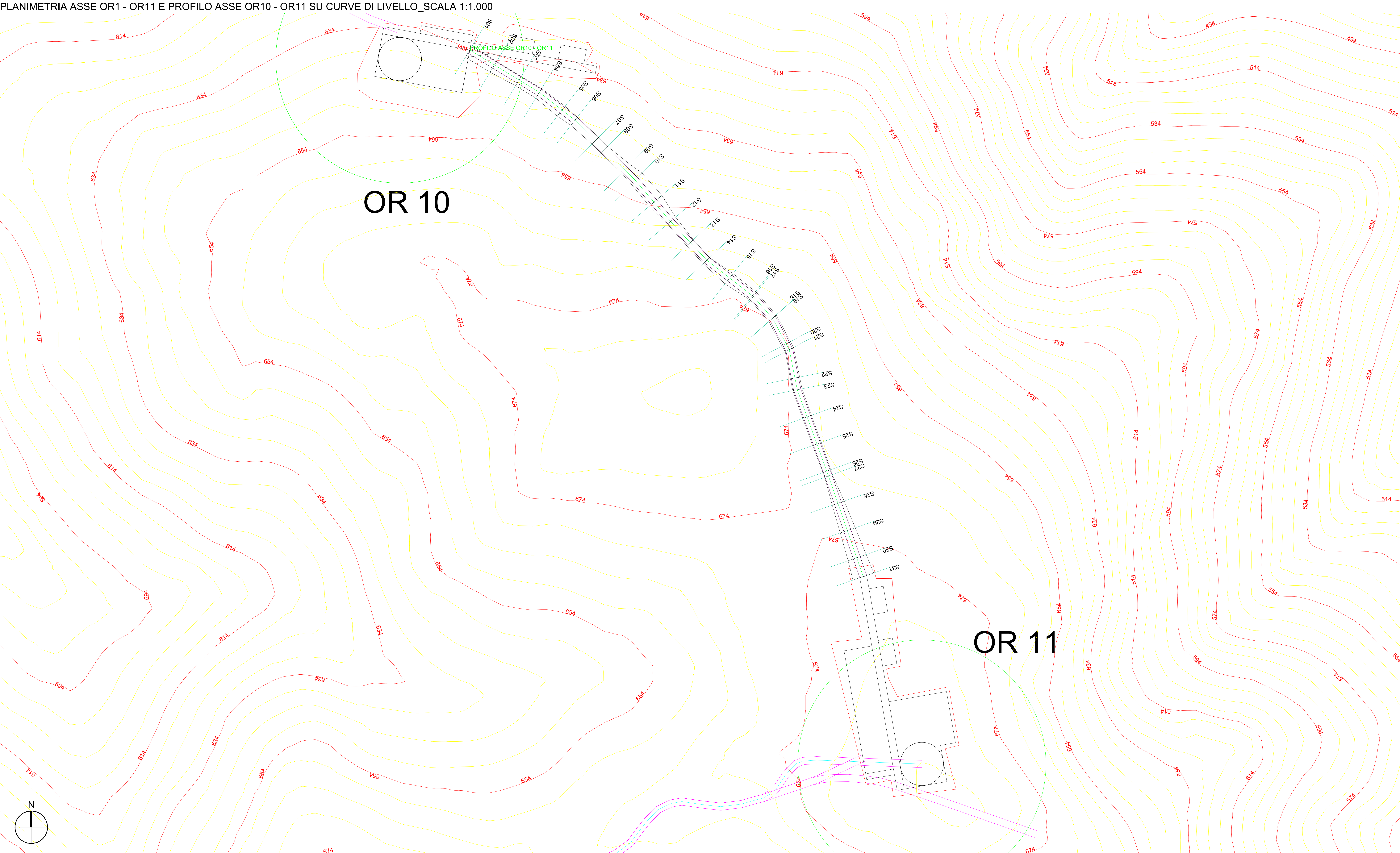
PLANIMETRIA ASSE OR1 - OR11 E PROFILO ASSE OR10 - OR11 SU CURVE DI LIVELLO_SCALA 1:1.000
