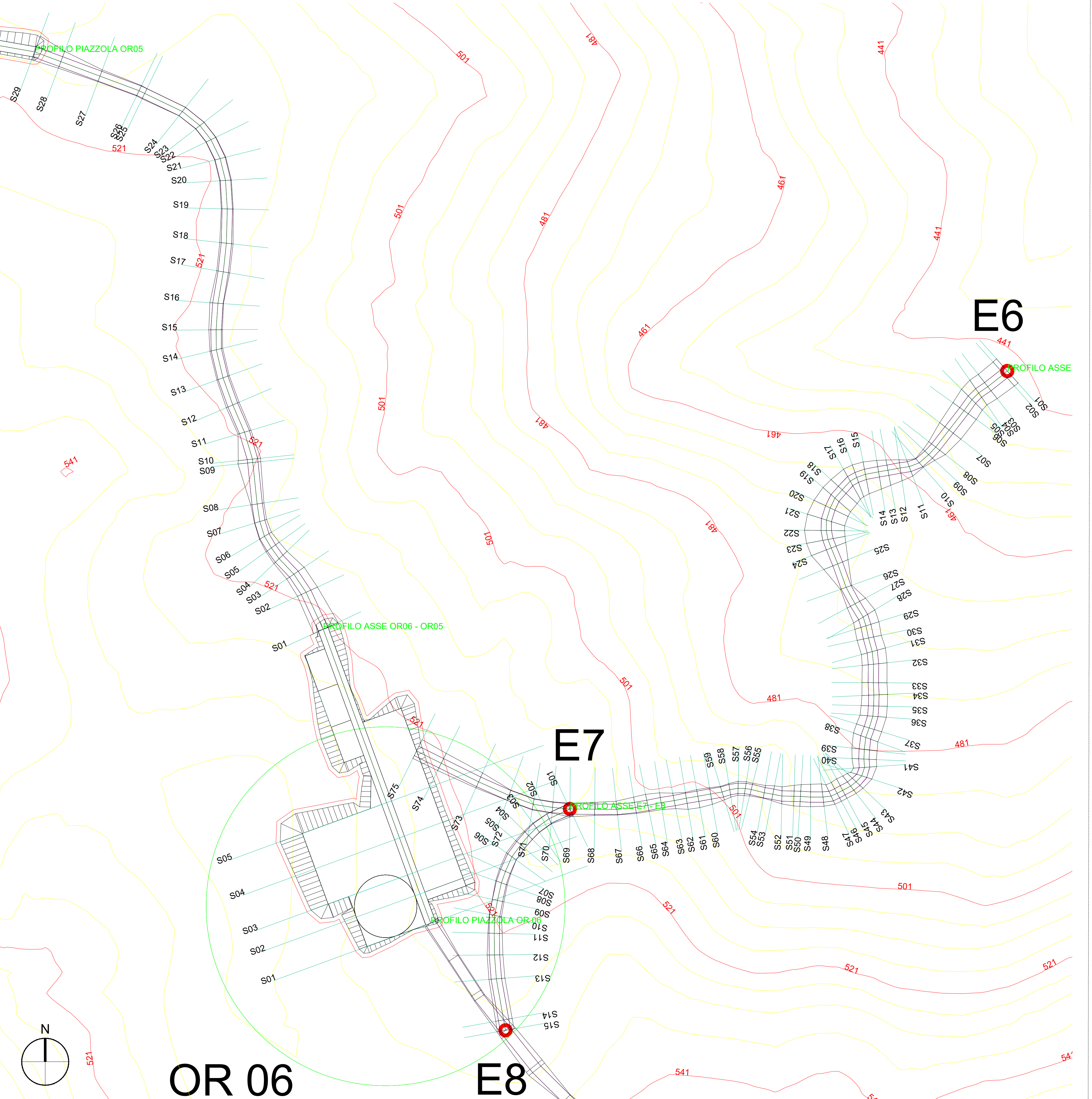
PLANIMETRIA PIAZZOLA OR06 E PROFILO E7 - E8 - E6 - OR06 SU CURVE DI LIVELLO_SCALE 1:1.000
