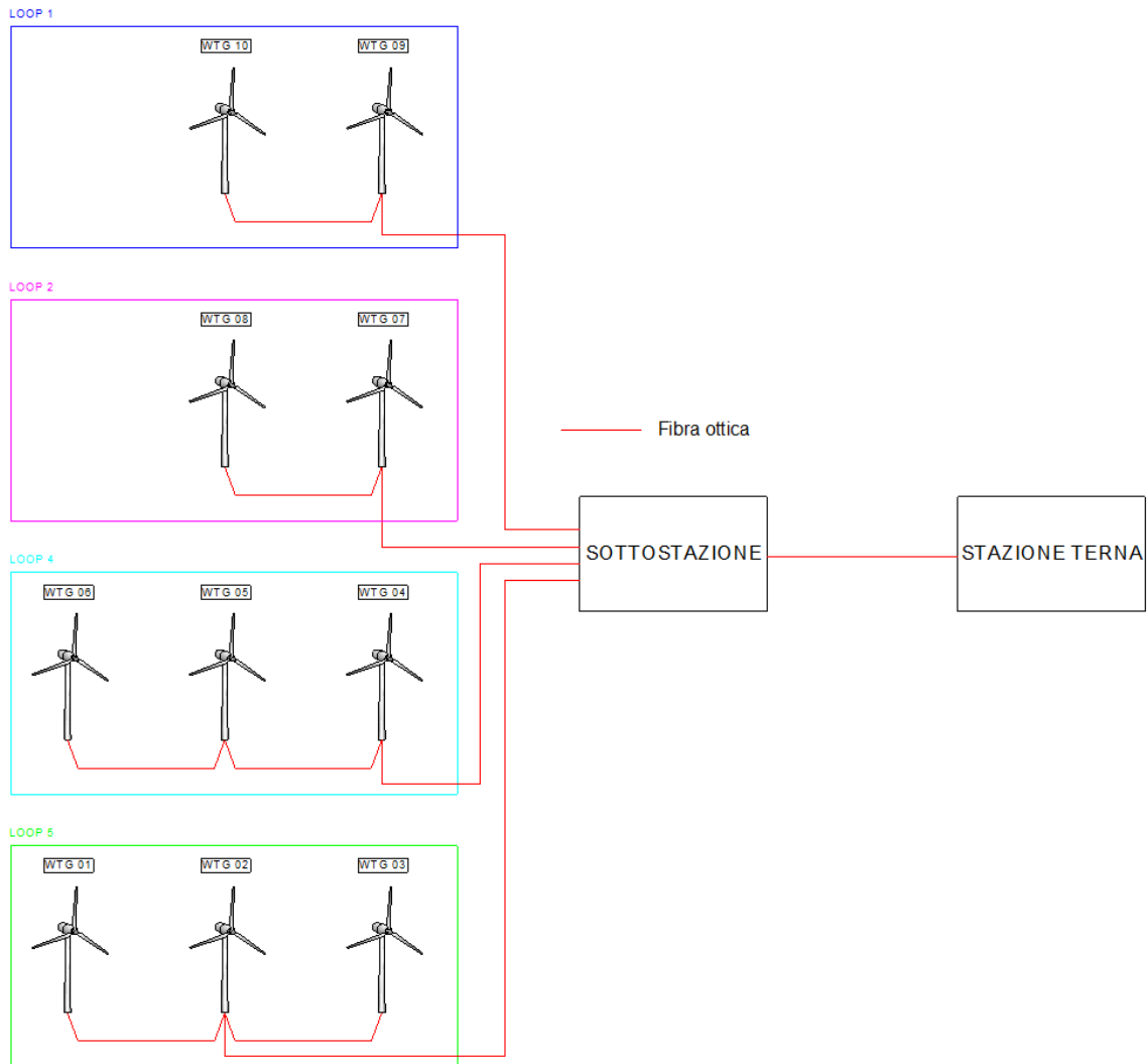
Figura 1 - Schema fibra ottica
