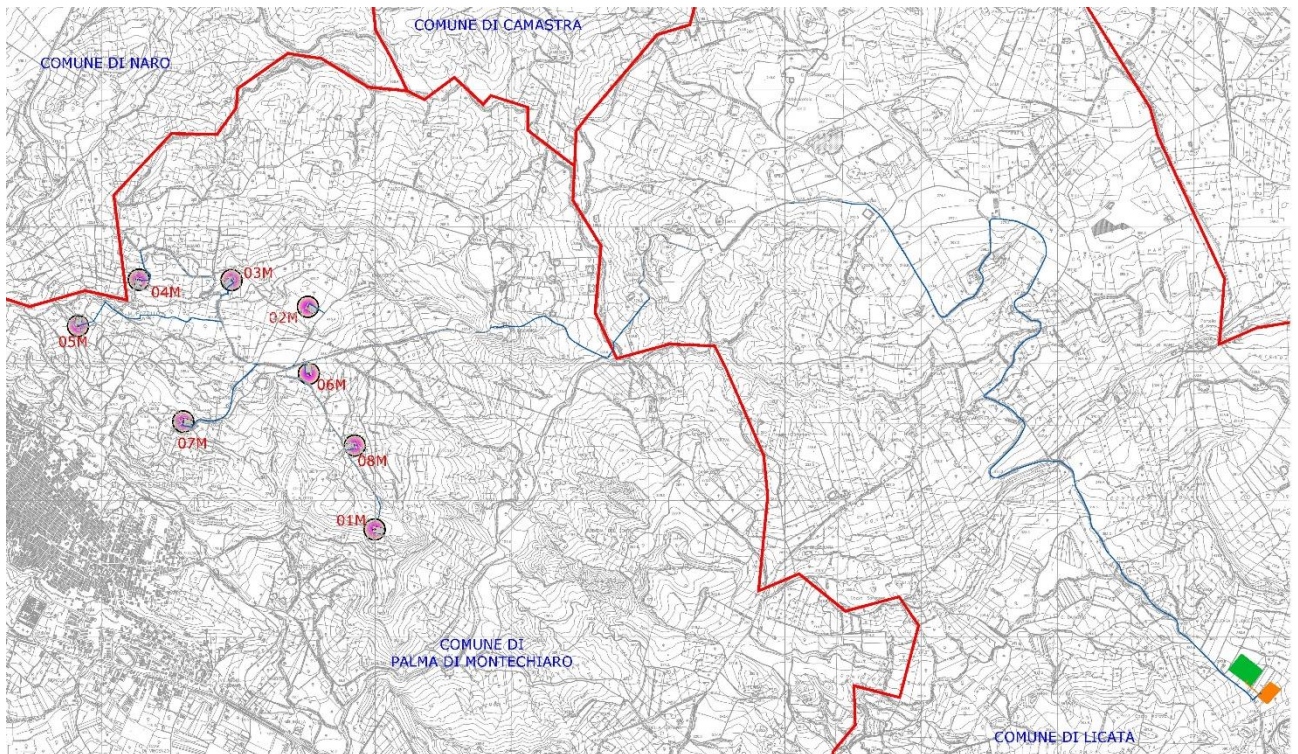
Fig.2a- Inquadramento impianto su CTR 1:10.000
