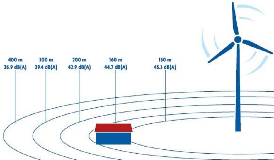
Figura 26 Curve isofoniche e potenziali recettori di impatto acustico; fonte: ANEV 2022
