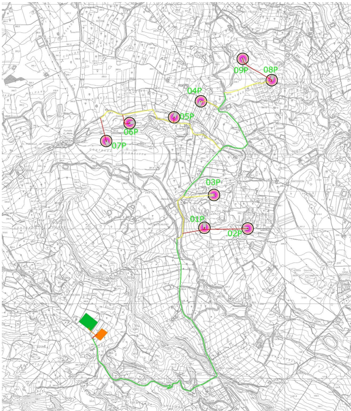
Figura 5 Schema della viabilità di accesso al parco eolico
