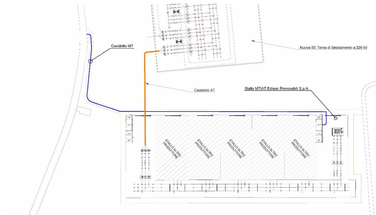
Inquadramento dell'area della Stazione Elettrica Condivisa tra i Produttori
