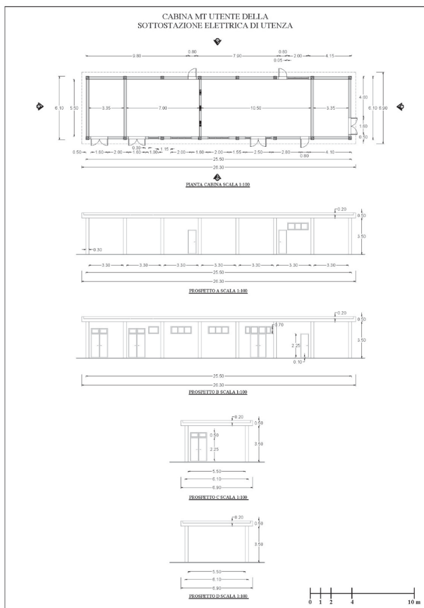
Particolari della cabina MT all'interno della Sottostazione elettrica di Utenza
