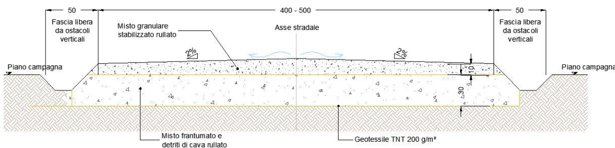
Figura 6 Sezione tipo pista di impianto; misure in centimetri
