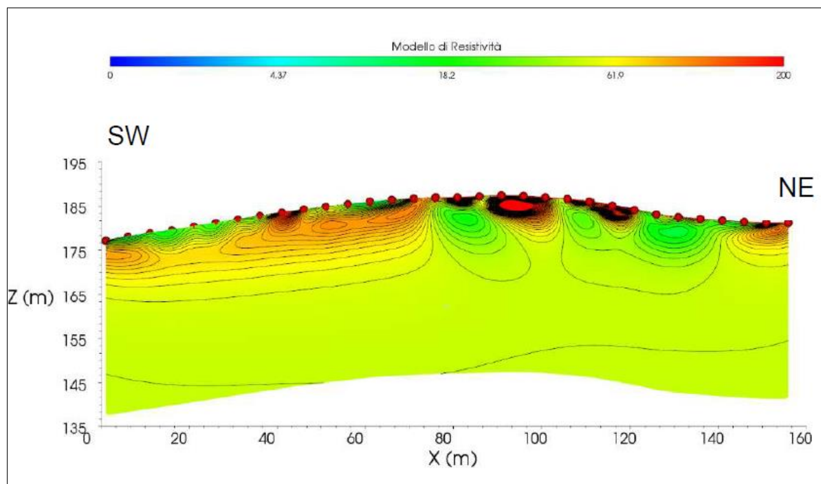
Figura 7-B: Tomografia elettrica ERT18_SM_L
