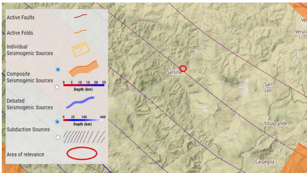
Figura 6-H: Stralcio database DISS versione 3.3.0 (2021, INGV) relativamente all’area di interesse.
