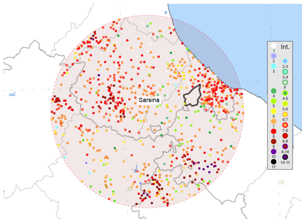
Figura 6-A: Mappa dei terremoti storici avvenuti dall'anno 1000 al 2020 in un raggio di 50 km dal Comune di Sarsina (da Catalogo Parametrico dei Terremoti Italiani, CPTI15 v. 4.0, Rovida et. al. 2022, INGV). http://emidius.mi.ingv.it/CPTI15-DBMI15 .
