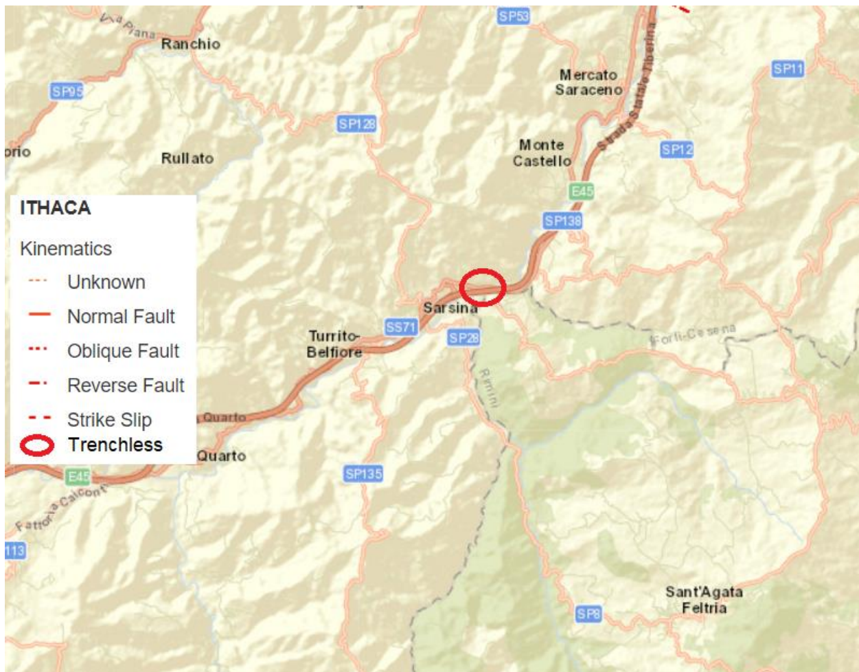
Figura 6-I: Stralcio database ITHACA (ISPRA) relativamente all'area di interesse. Accessibile al link https://sgi.isprambiente.it/ithaca/viewer/index.html
