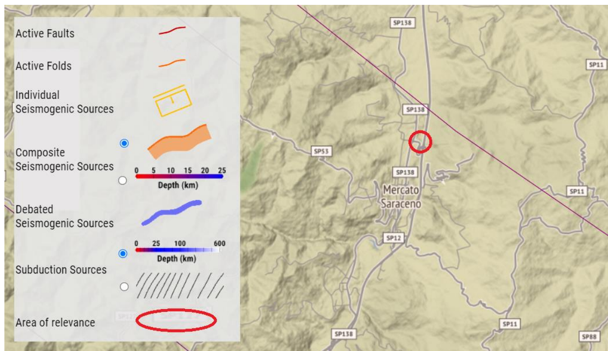
Figura 6-H: Stralcio database DISS versione 3.3.0 (2021, INGV) relativamente all’area di interesse.
