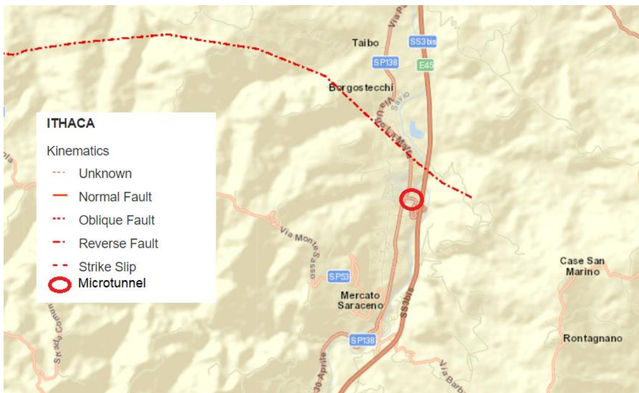
Figura 6-I: Stralcio database ITHACA (ISPRA) relativamente all'area di interesse. Accessibile al link http://sgi.isprambiente.it/ithaca/viewer/index.html#
