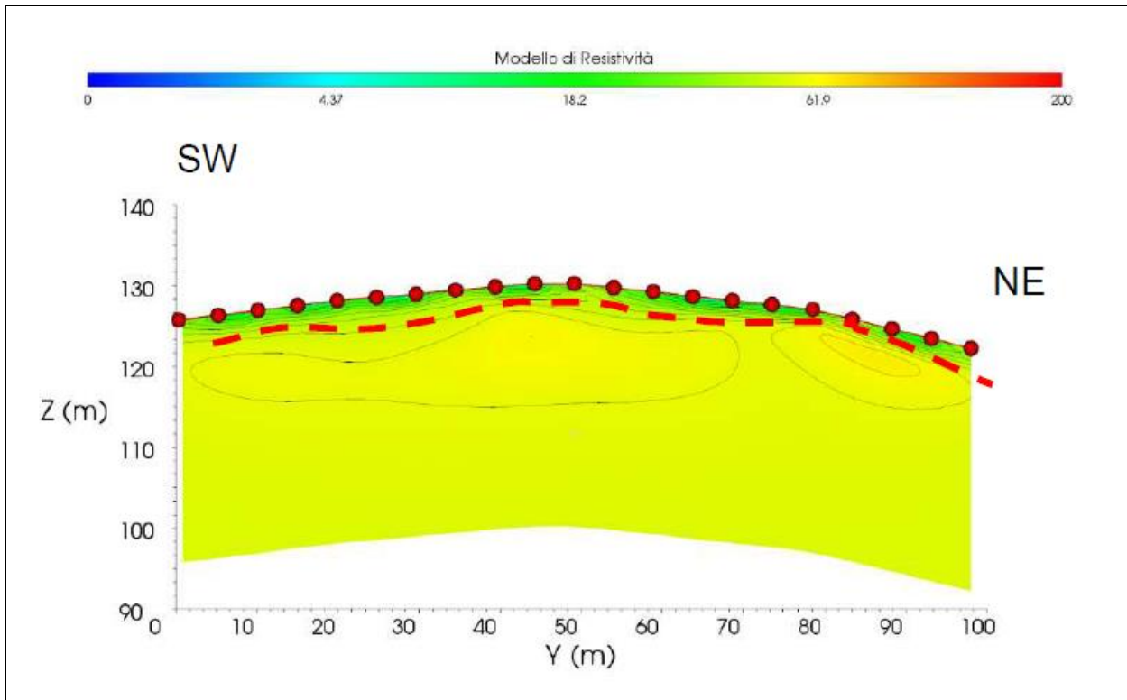
Figura 7-B: Tomografia elettrica ERT23_SM_L
